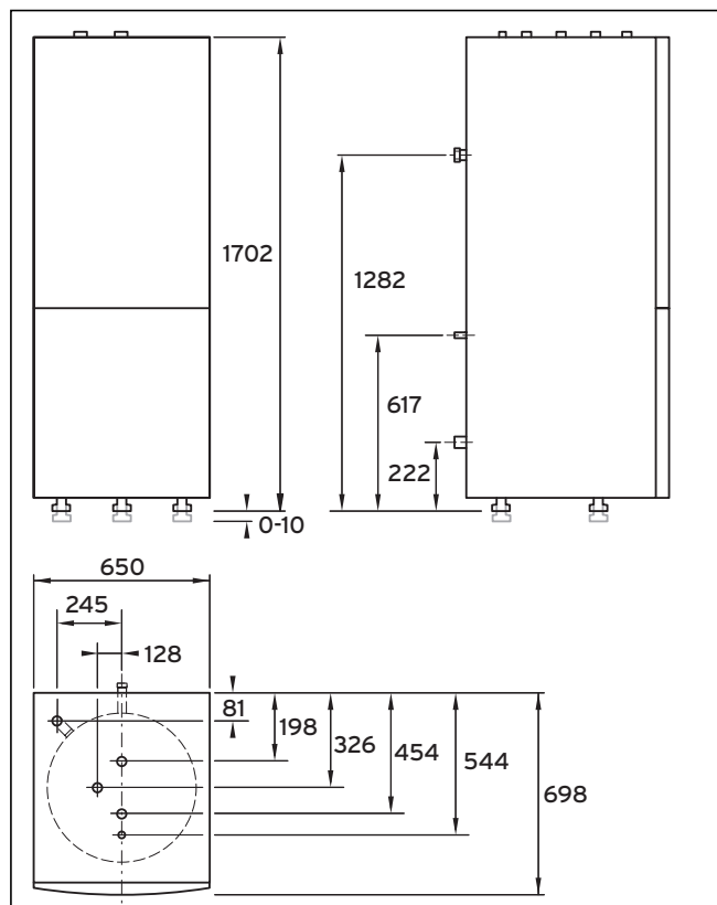
Fig. 4.2 Mål
