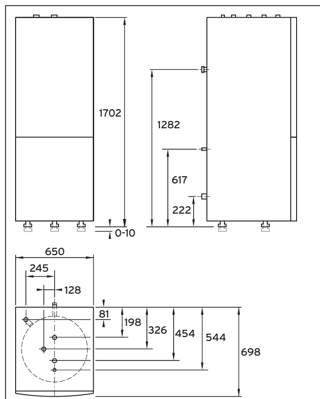
Afb. 4.2 Afmetingen
