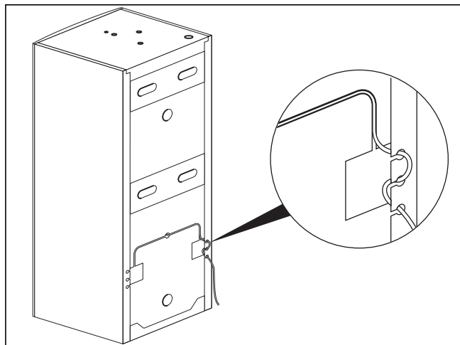
Obr. 5.1 Připojení vedení čidla zásobníku
