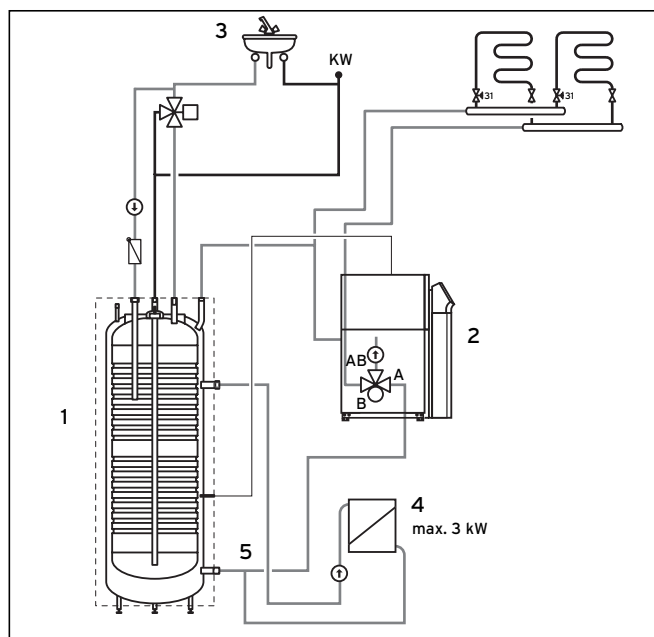
Fig. 4.5 Installation du ballon d'eau chaude sanitaire avec radiateur additionnel
