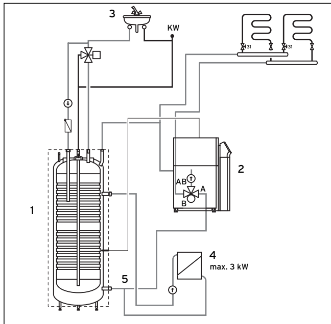
Fig. 4.5 Installation som varmtvandsbeholder med ekstra radiator
