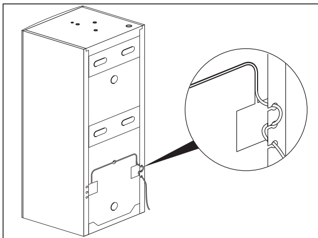
Abb. 5.1 Speicherfühlerleitung anschließen
