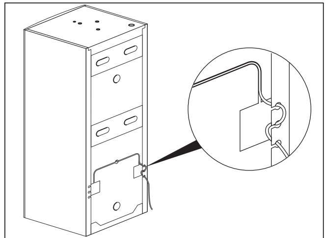
Rys. 5.1 Podłączanie przewodu czujnika zasobnika
