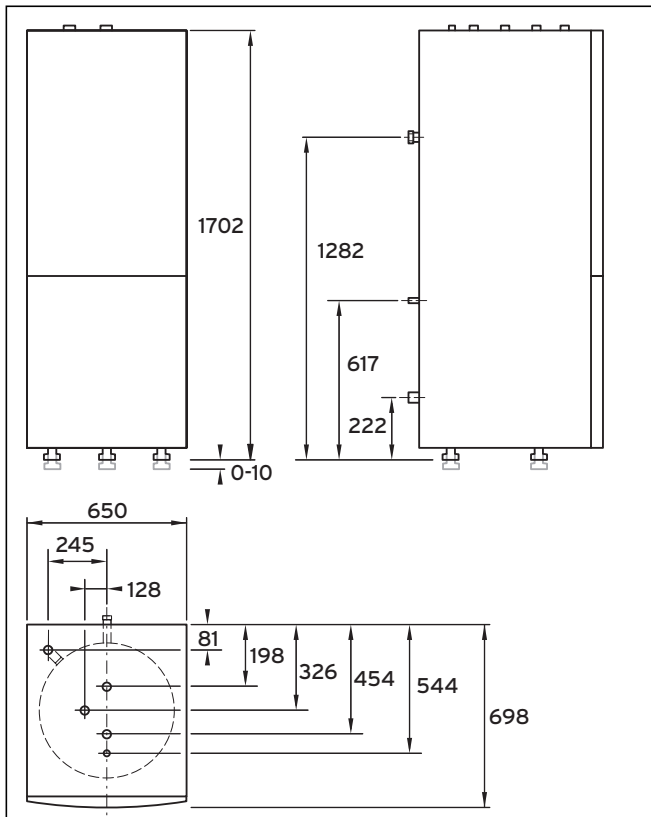
Bild 4.2 Mått
