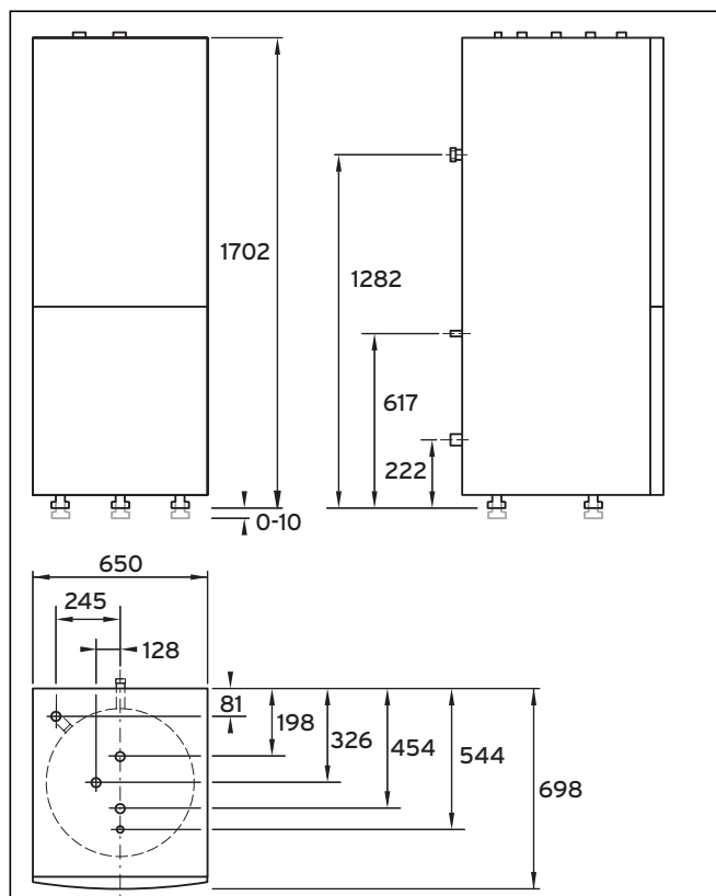
Obr. 4.2 Rozměry
