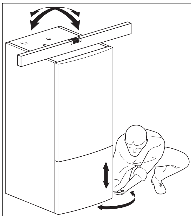
Kuva 4.3 Laitteen suuntaaminen
