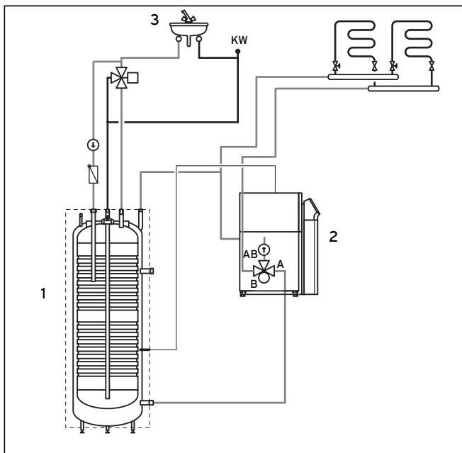
Bild 4.4 Installation av varmvattenberedaren utan radiator
