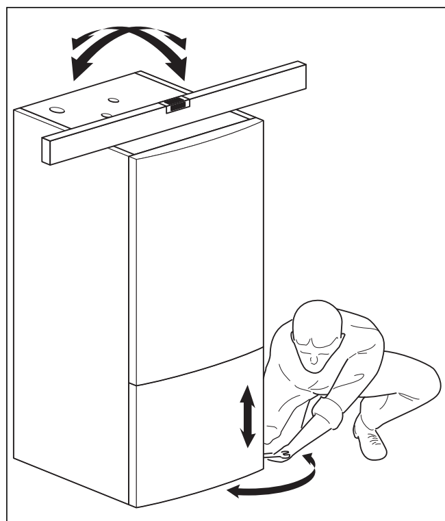
Obr. 4.3 Vyrovnání zařízení
