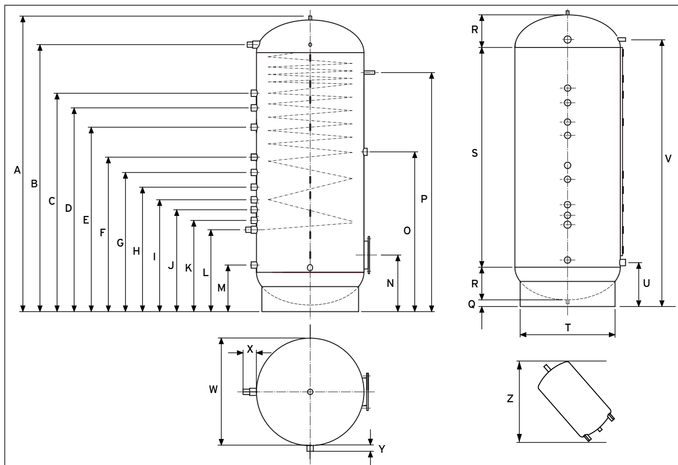
Bild 4.3 Mått
