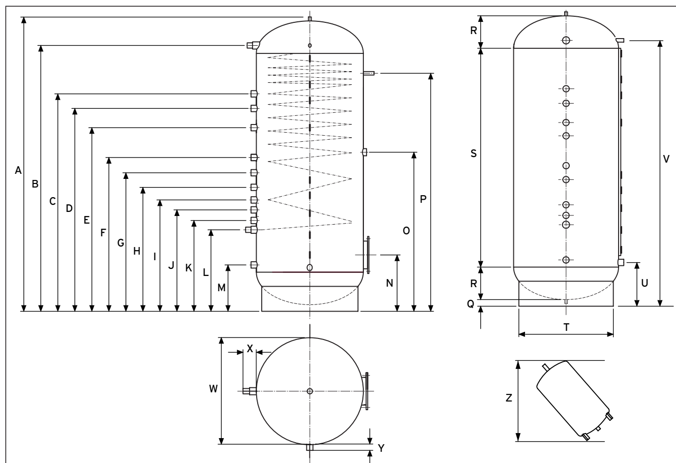
Fig. 4.3 Dimensions
