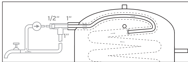
Bild 4.2 Cirkulationsstav
