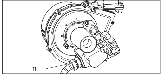
Abb. 8.8 Gasdichtheit prüfen
