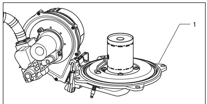
Abb. 8.5 Brennentürdichtung ersetzen
