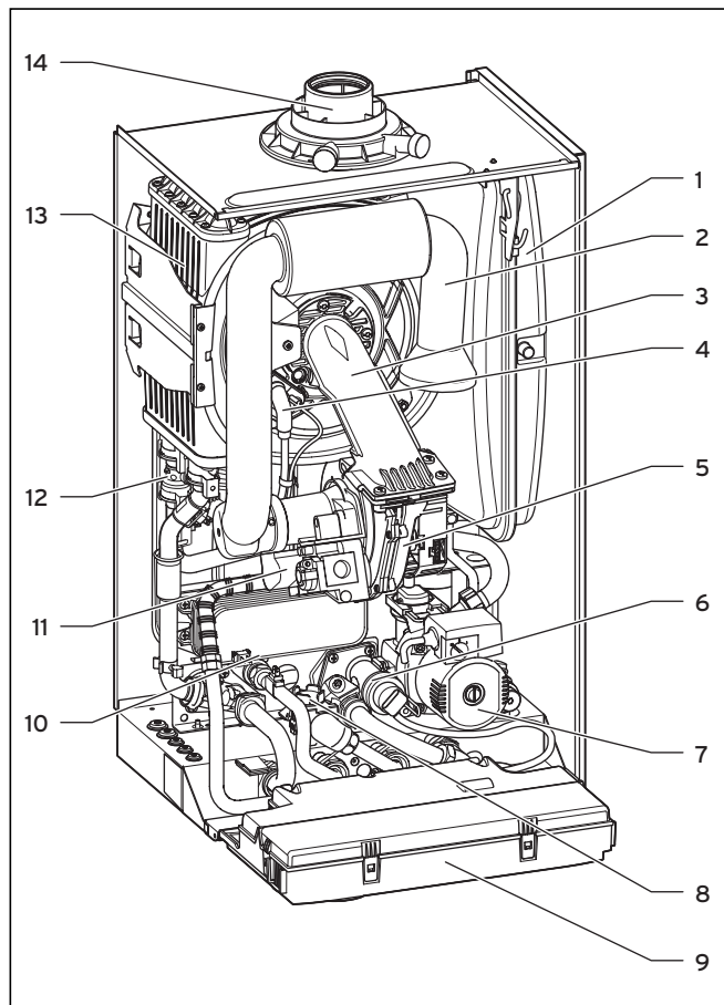
Abb. 2.1 Funktionselemente VCW
