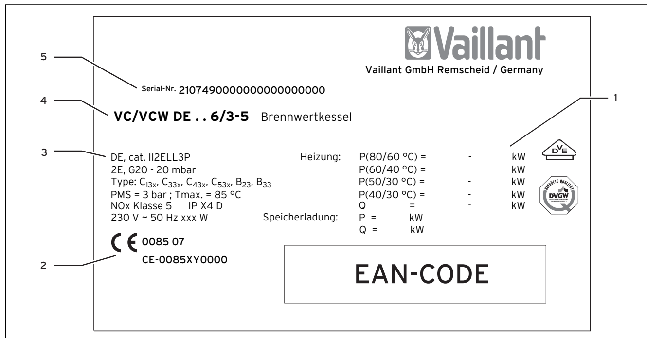
Abb. 1.1 Typenschild
