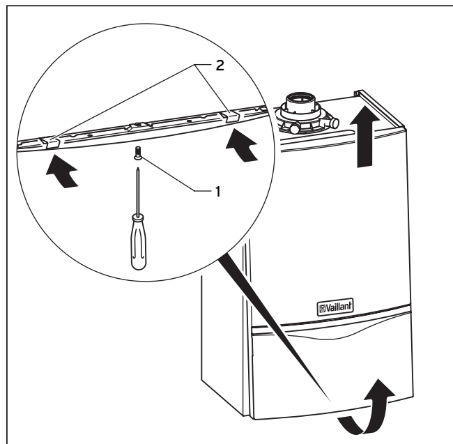
Abb. 4.8 Geräteverkleidung abnehmen
