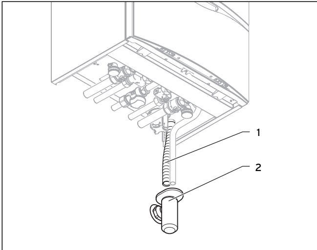
Abb. 5.8 Kondenswasserablauf
