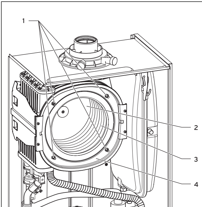
Abb. 8.3 Integral-Kondensations-Wärmetauscher reinigen
