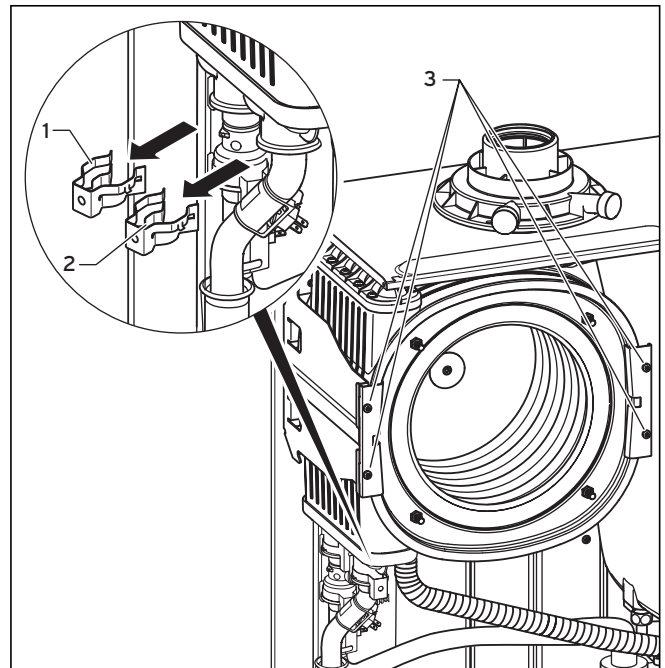
Abb. 10.5 Primärwärmetauscher austauschen
