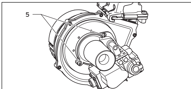
Abb. 10.3 Verschaubung Gasarmatur/Gebläse
