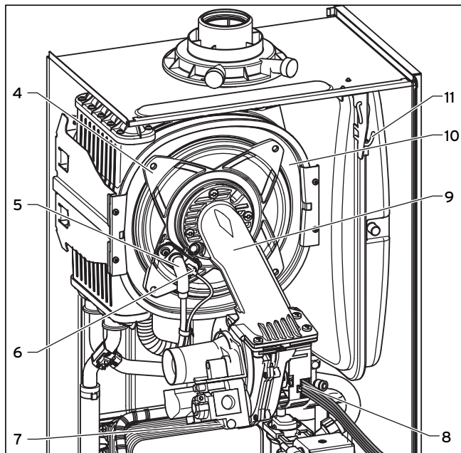
Abb. 8.2 Thermo-Kompaktmodul ausbauen
