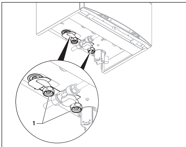
Abb. 5.3 Speicheranschluss montieren
