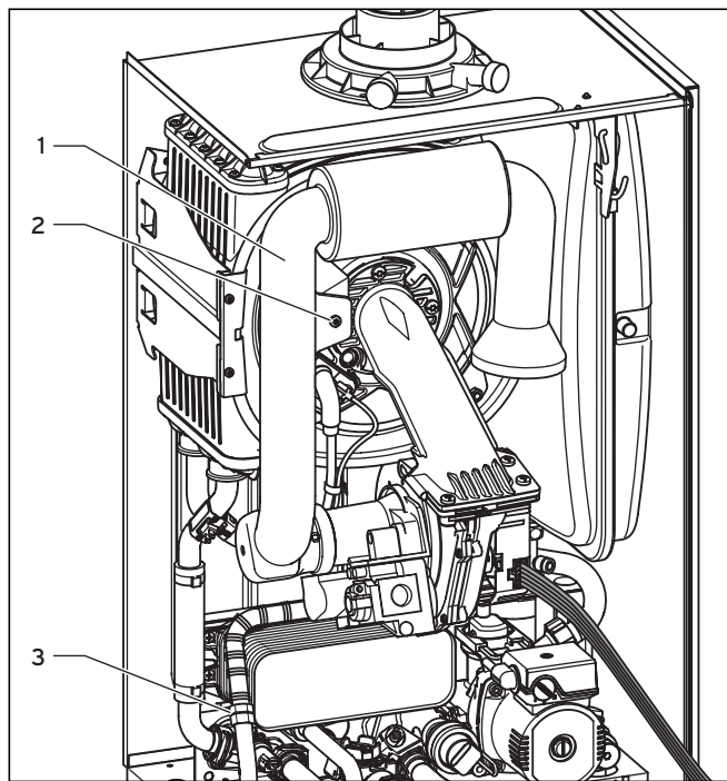
Abb. 8.1 Luftansaugrohr ausbauen
