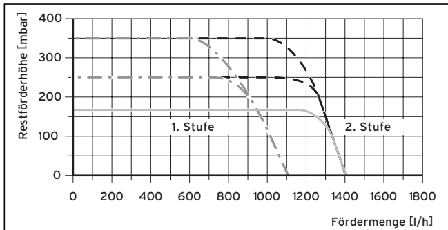
Abb. 7.2 Pumpenkennlinie
