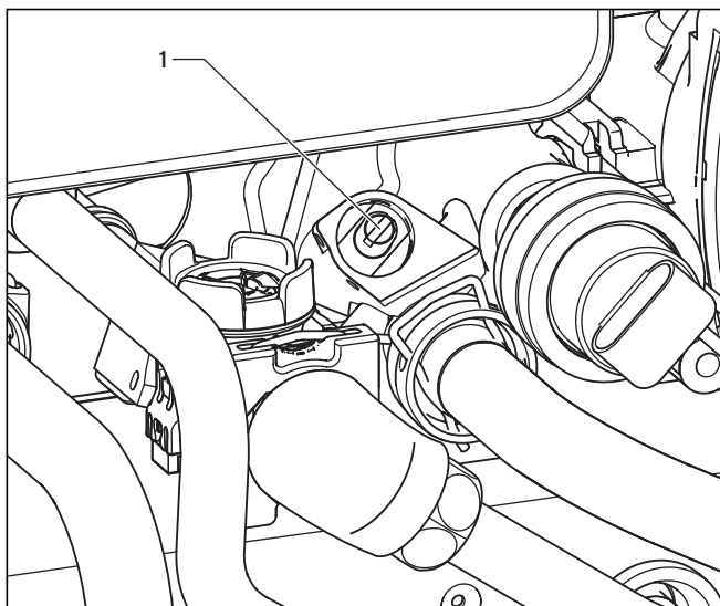
Abb. 7.3 Überströmventil einstellen
