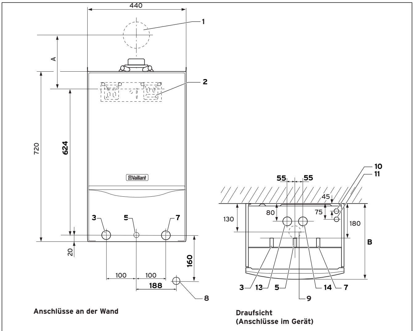
Abb. 4.4 Anschlussmaße in mm (VC-Geräte)
