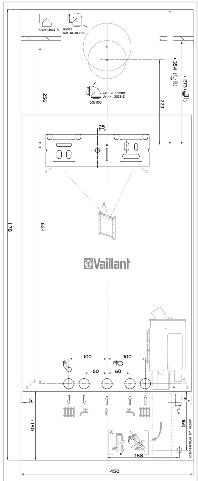
Abb. 4.6 Montageschablone/Montagefreiräume
