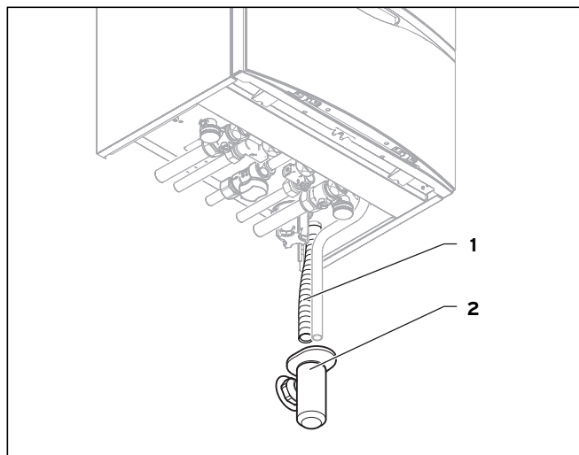
Abb. 5.8 Kondenswasserablauf
