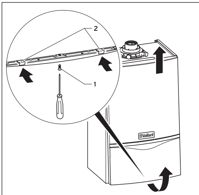
Abb. 4.8 Geräteverkleidung abnehmen
