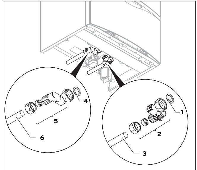
Abb. 5.2 Kalt- und Warmwasseranschluss montieren
