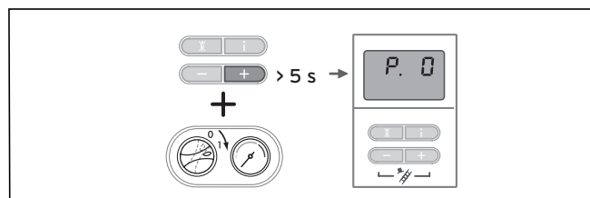
Abb. 9.2 Prüfprogramme aktivieren
