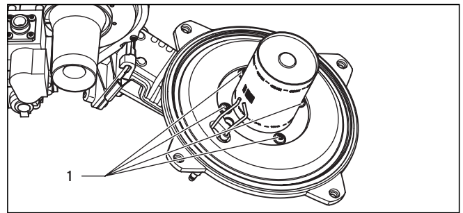
Abb. 10.1 Brenner austauschen
