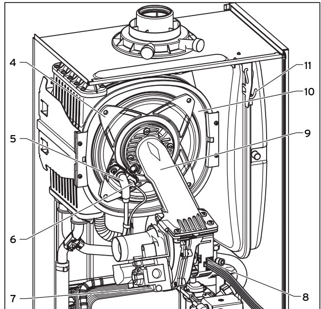
Abb. 8.2 Thermo-Kompaktmodul ausbauen
