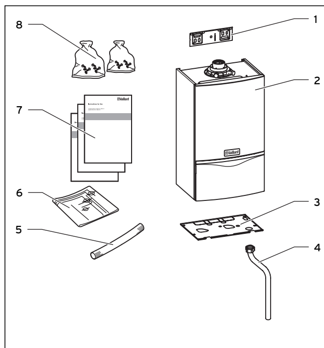
Abb. 4.2 Lieferumfang VC-Geräte
