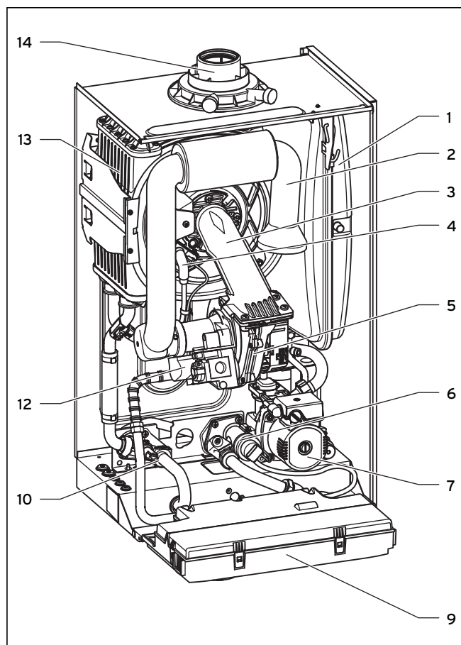
Abb. 2.2 Funktionselemente VC
