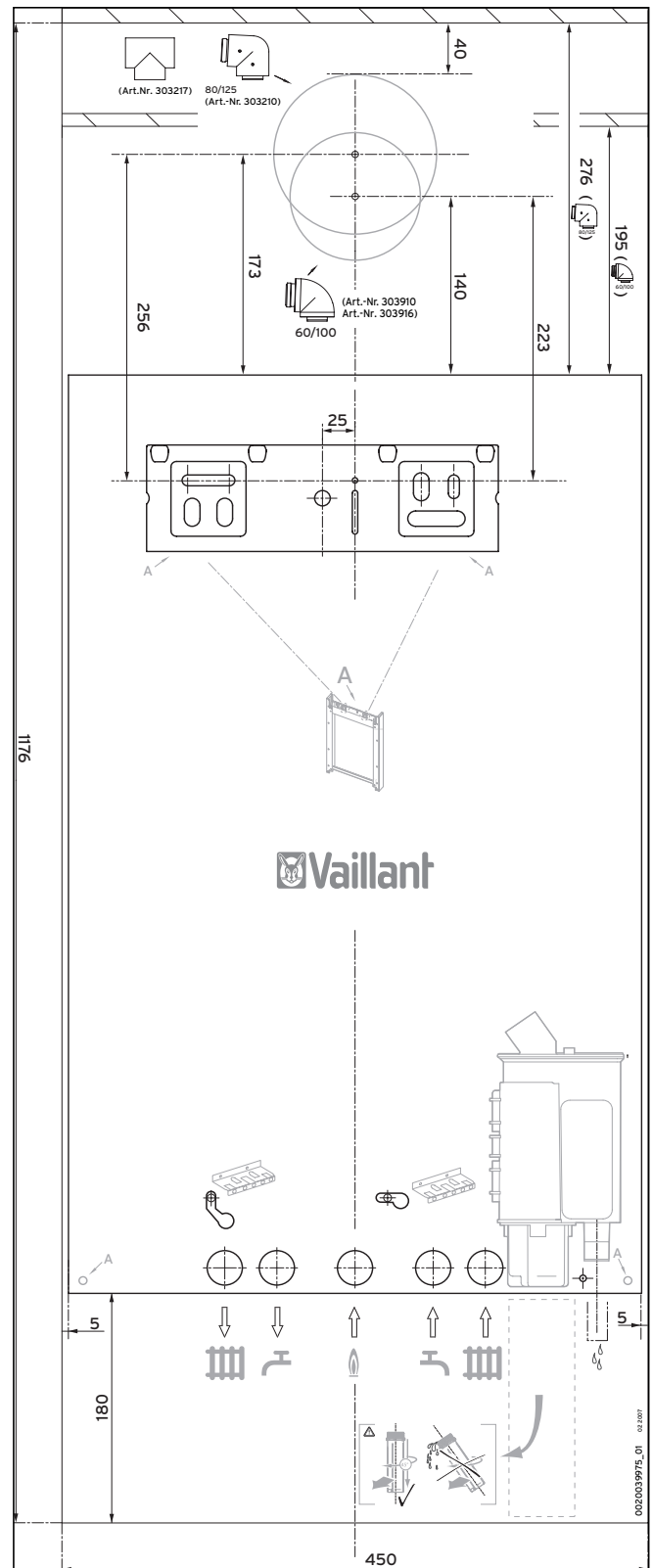
Abb. 4.6 Montageschablone/Montagefreiräume
