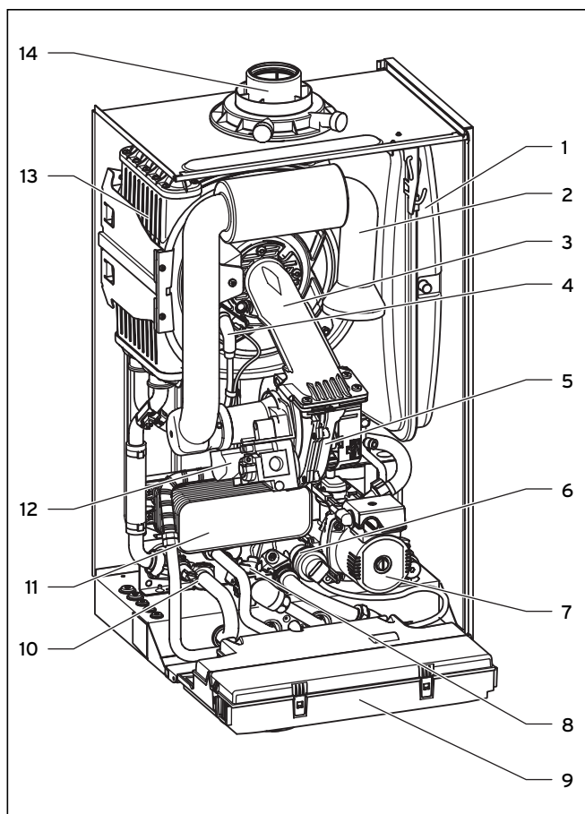
Abb. 2.1 Funktionselemente VCW
