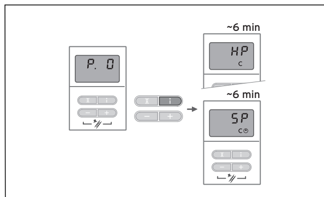
Abb. 9.5 Displayanzeige Entlüftungsprogramm
