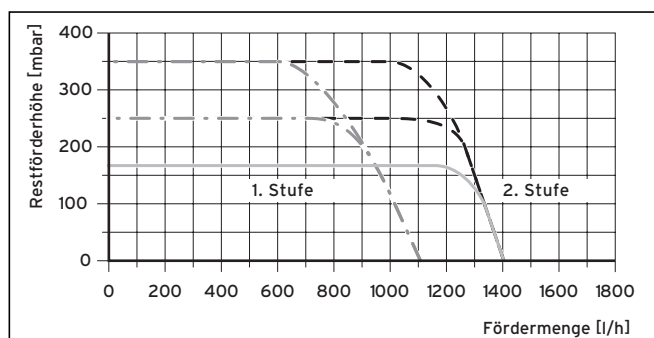
Abb. 7.2 Pumpenkennlinie
