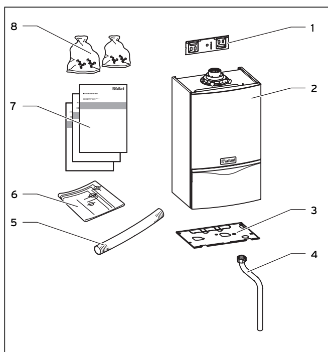
Abb. 4.1 Lieferumfang VCW-Geräte
