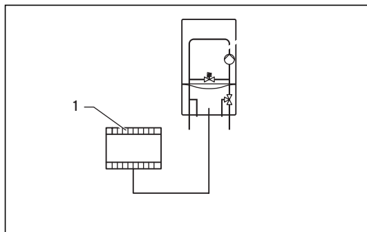
Fig. 5.1 Raccordement de l'interface 0-10 V
