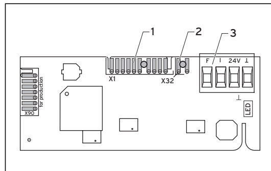
Abb. 3.3 Anschlüsse bei Leistungssollwert (ohne Stecker X1)
