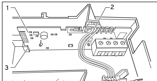
Afb. 4.2 Interface-printplaat 0-10 V inbouwen
