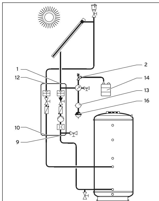
Abb. 4.2 Hydraulische Einbindung der Solarstation
