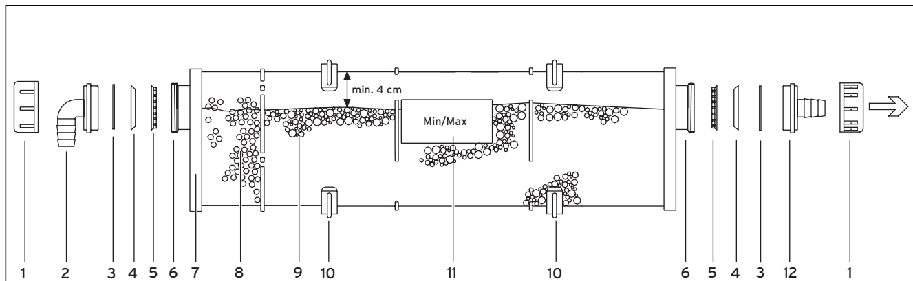
Fig. 3.1 Opbygning olieneutralisationsanordning
