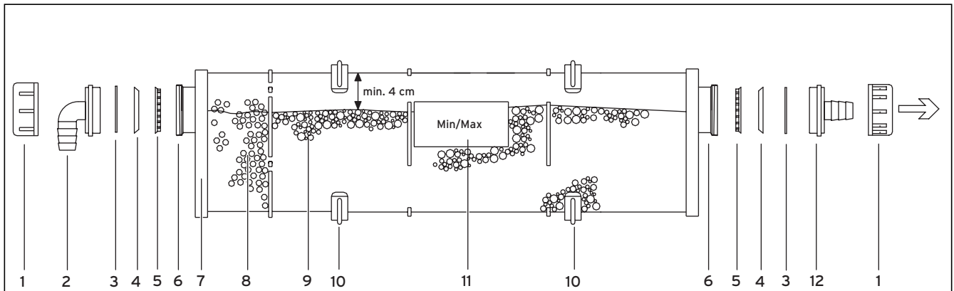
Abb. 3.1 Aufbau Öl-Neutralisations-Einrichtung
