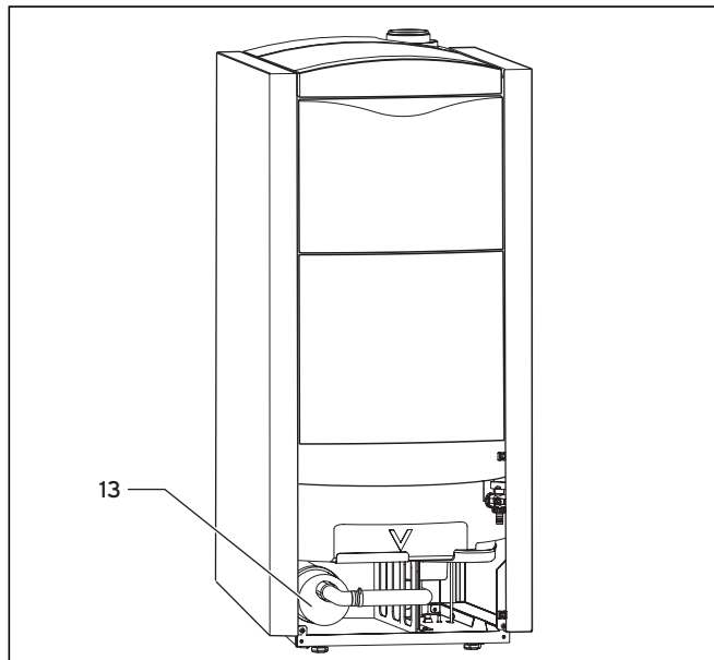
Abb. 4.1 Öl-Neutralisations-Einrichtung platzieren
