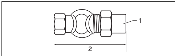
Sl. 3.2 Zaporni gasni ventil u prolaznoj varijanti Model-br. GCSN DN 15, 20, 25
