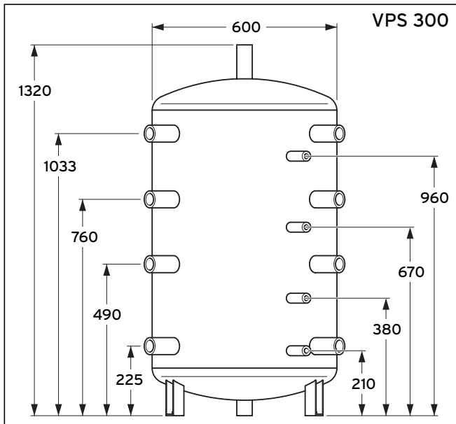
Abb. 4.2 Abmessungen VPS 300 *
