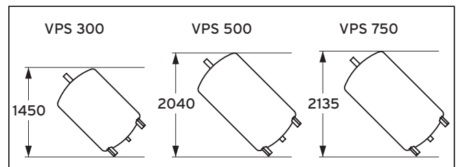
Abb. 4.6 Kippmaße
