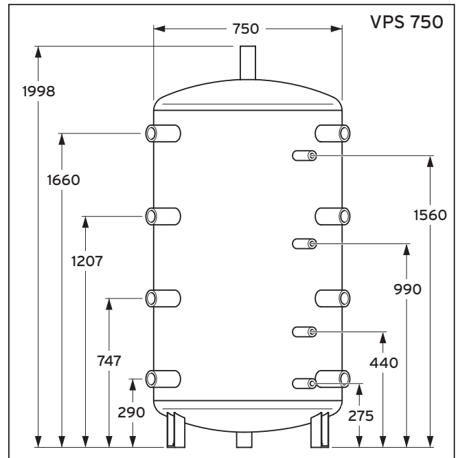
Abb. 4.4 Abmessungen VPS 750 *
