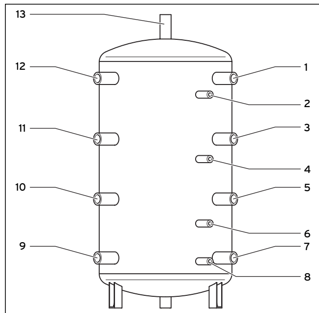
Fig. 2.2 Raccords (arrière)
