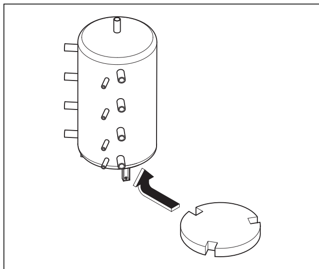
Afb. 4.7 Voetvulling aanbrengen
