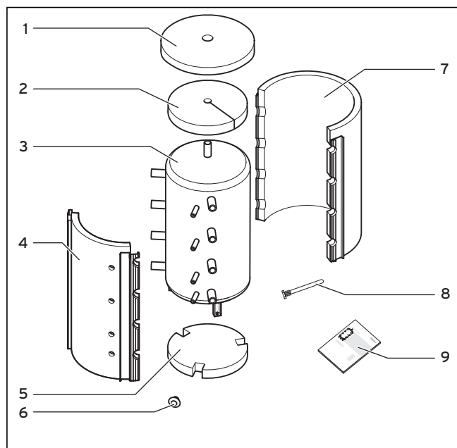
Bild 4.1 Leveransomfattning
