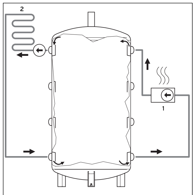
Bild 2.1 Ackumulatortankens funktionsprincip
