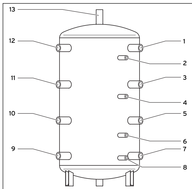
Abb. 2.2 Anschlüsse (hinten)
