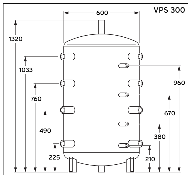
Fig. 4.2 Mål VPS 300 *
