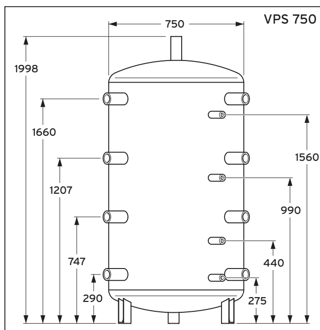
Fig. 4.4 Mål VPS 750 *
