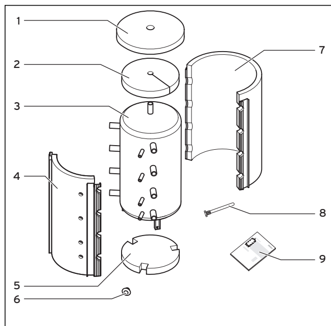
Fig. 4.1 Leveringsomfang
