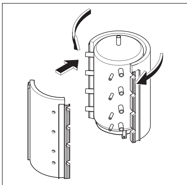
Afb. 4.8 Isolaties aanbrengen
