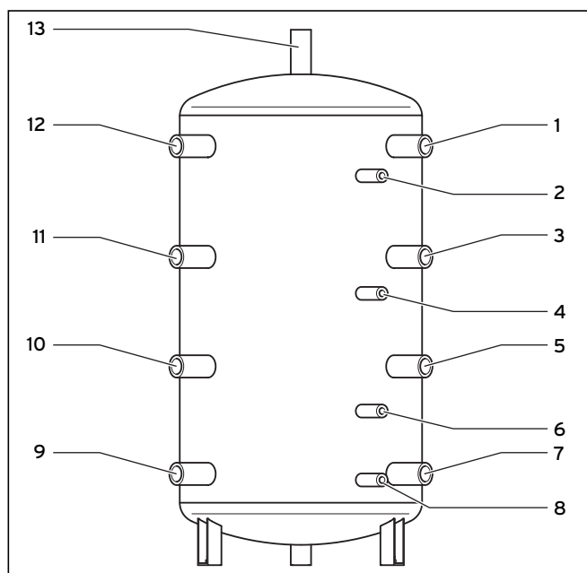
Fig. 2.2 Raccords (arrière)
