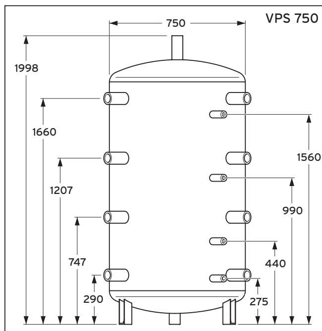
Afb. 4.4 Afmetingen VPS 750 *
