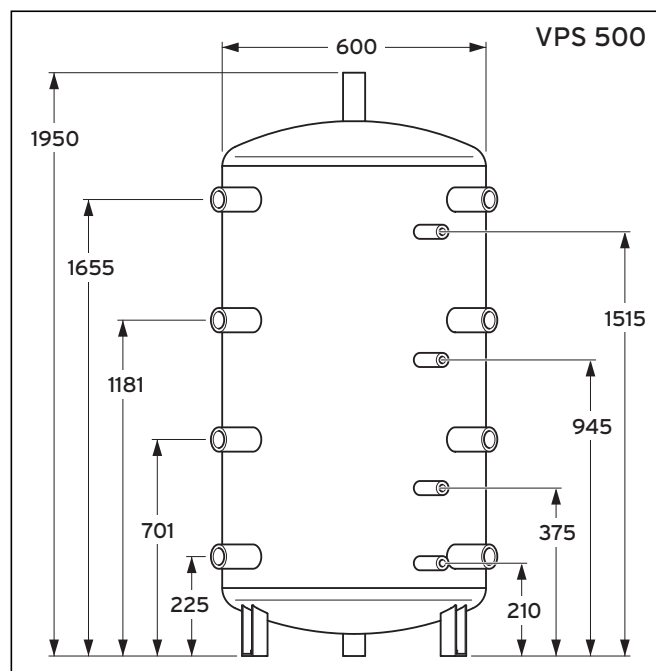
Abb. 4.3 Abmessungen VPS 500 *
