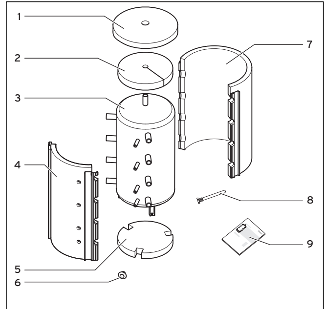
Abb. 4.1 Lieferumfang
