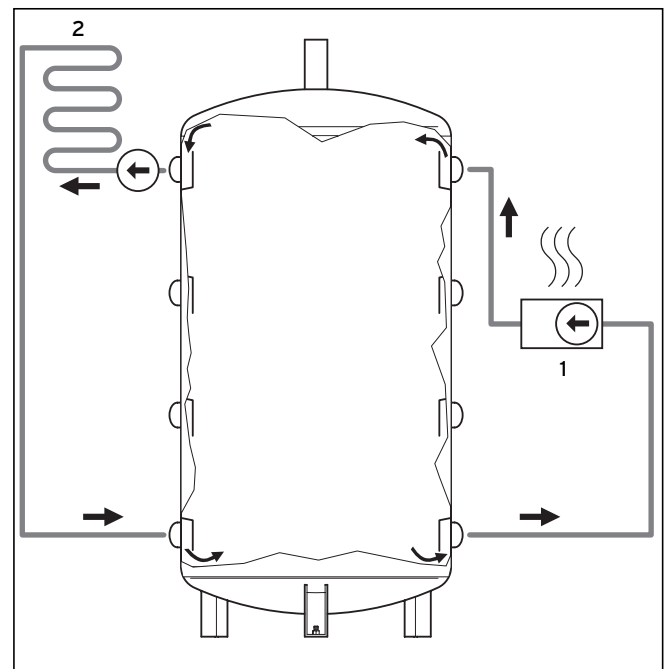
Fig. 2.1 Bufferbeholderens funktionsprincip
