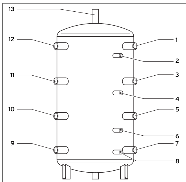
Fig. 2.2 Tilslutninger (bagsiden)
