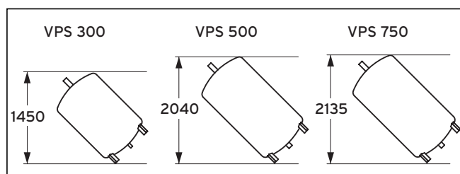
Afb. 4.6 Kantelafmetingen
