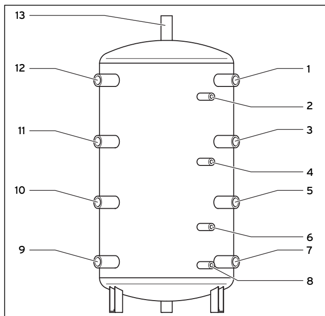
Abb. 2.2 Anschlüsse (hinten)
