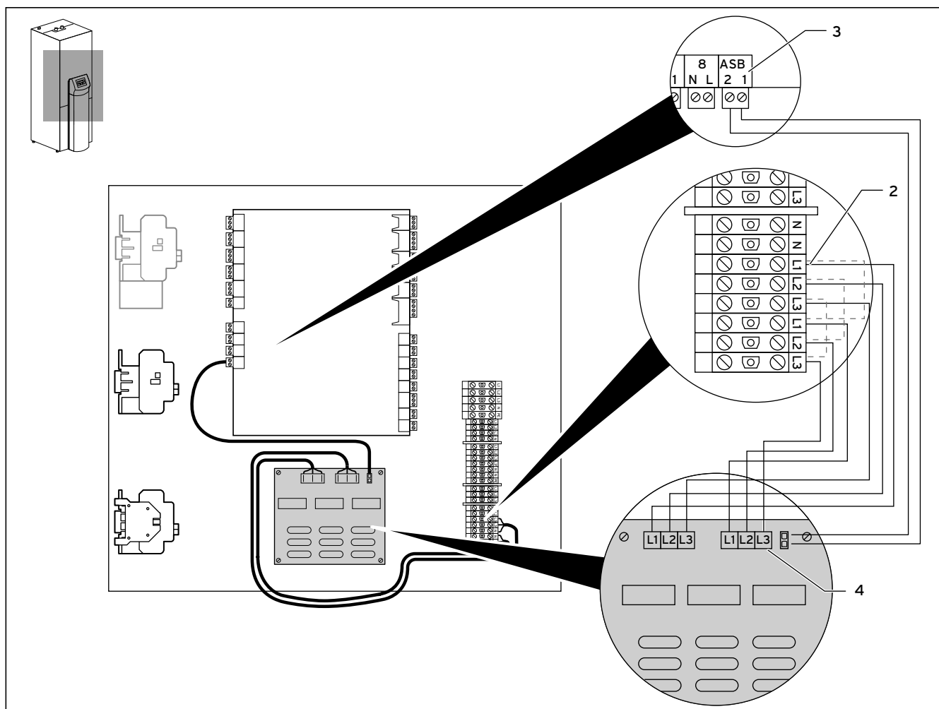
4.6 pav. Prijungimas prie geoTHERM VWS/VWW/VWL-S ..2 ir VWS ..3
