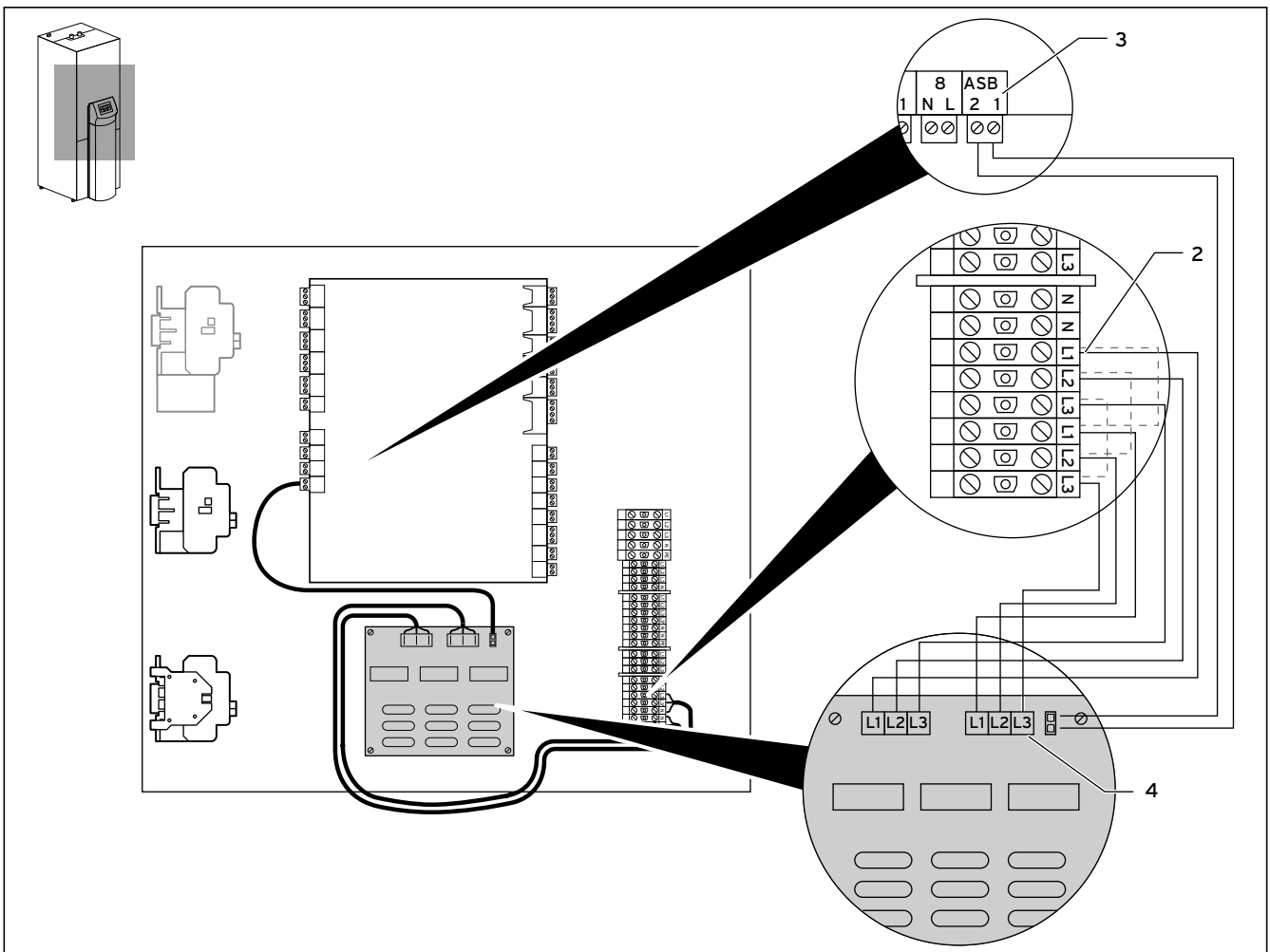
Afb. 4.6 Aansluiting aan geoTHERM VWS/VWW/VWL-S ..2 en VWS ..3
