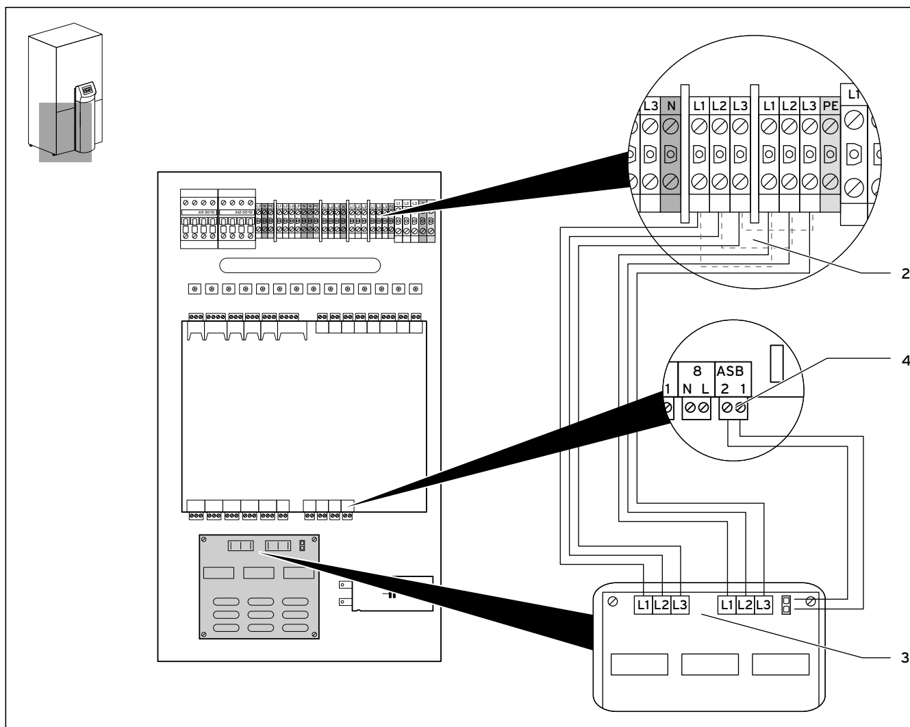
4.2 pav. Prijungimas prie geoTHERM VWL
