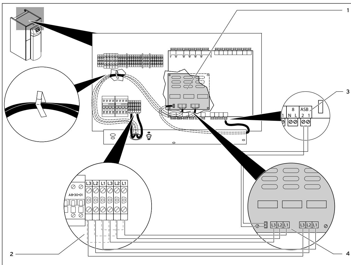
Fig. 4.4 Anslutning till geoTHERM VWS/VWW/VWL-S ..1 och VWS ..4
