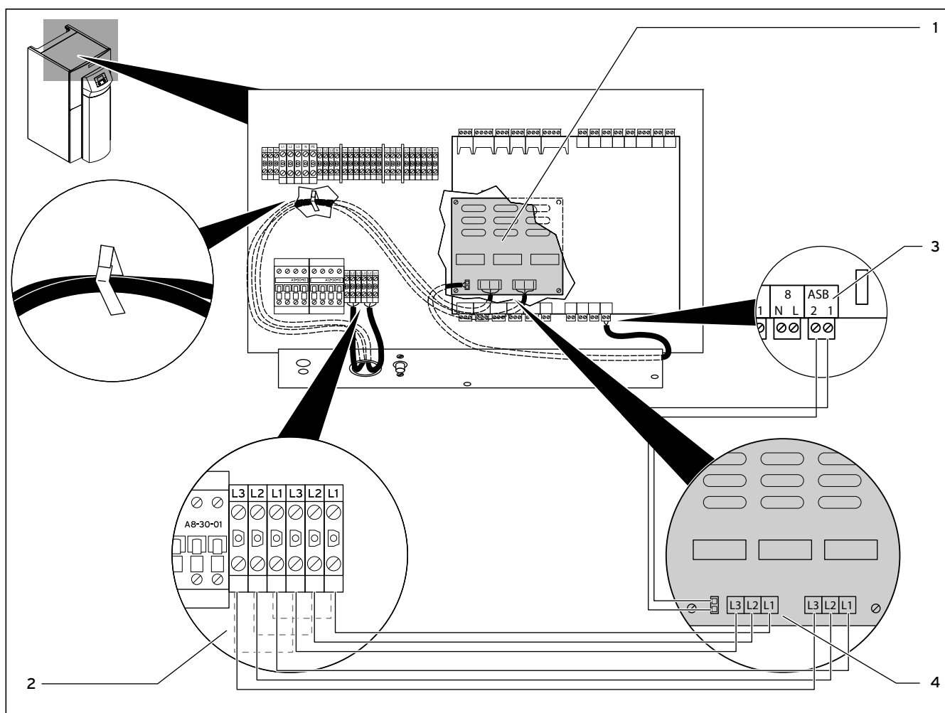
Rys. 4.4 Podłączenie do geoTHERM VWS/VWW/VWL-S ..1 i VWS ..4
