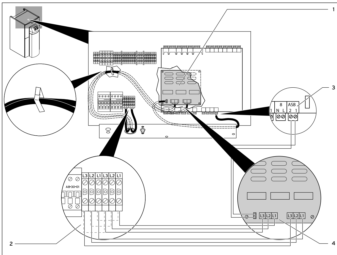
4.4. att. Pieslēgšana pie geoTHERM VWS/VWW/VWL-S ..1 un VWS ..4
