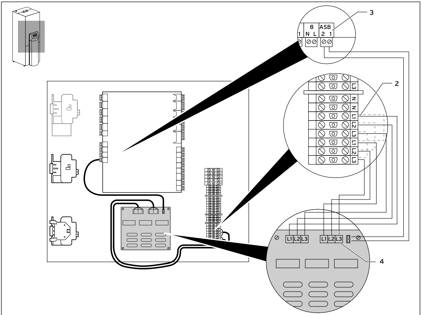
Kuva 4.6 Liitäntä laitteisiin geoTHERM VWS/VWW/VWL-S ..2 ja VWS ..3
