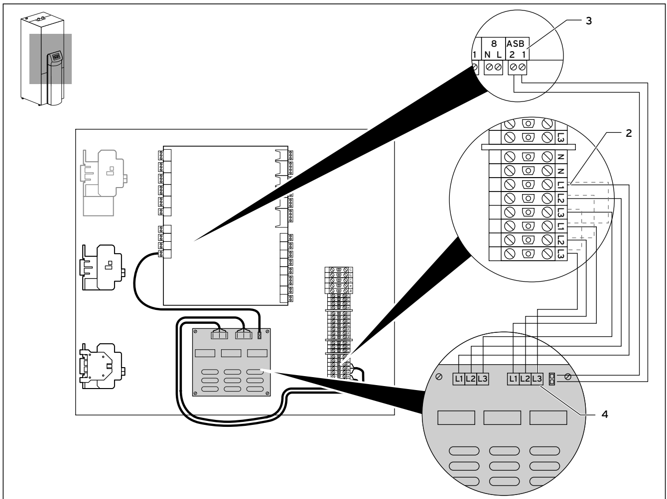
Abb. 4.6 Anschluss an geoTHERM VWS/VWW/VWL-S ..2 und VWS ..3
