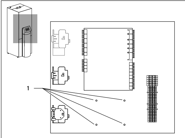
Kuva 4.5 Kiinnittimien asennus laitteisiin geoTHERM VWS/VWW/VWL-S ..2 ja VWS ..3
