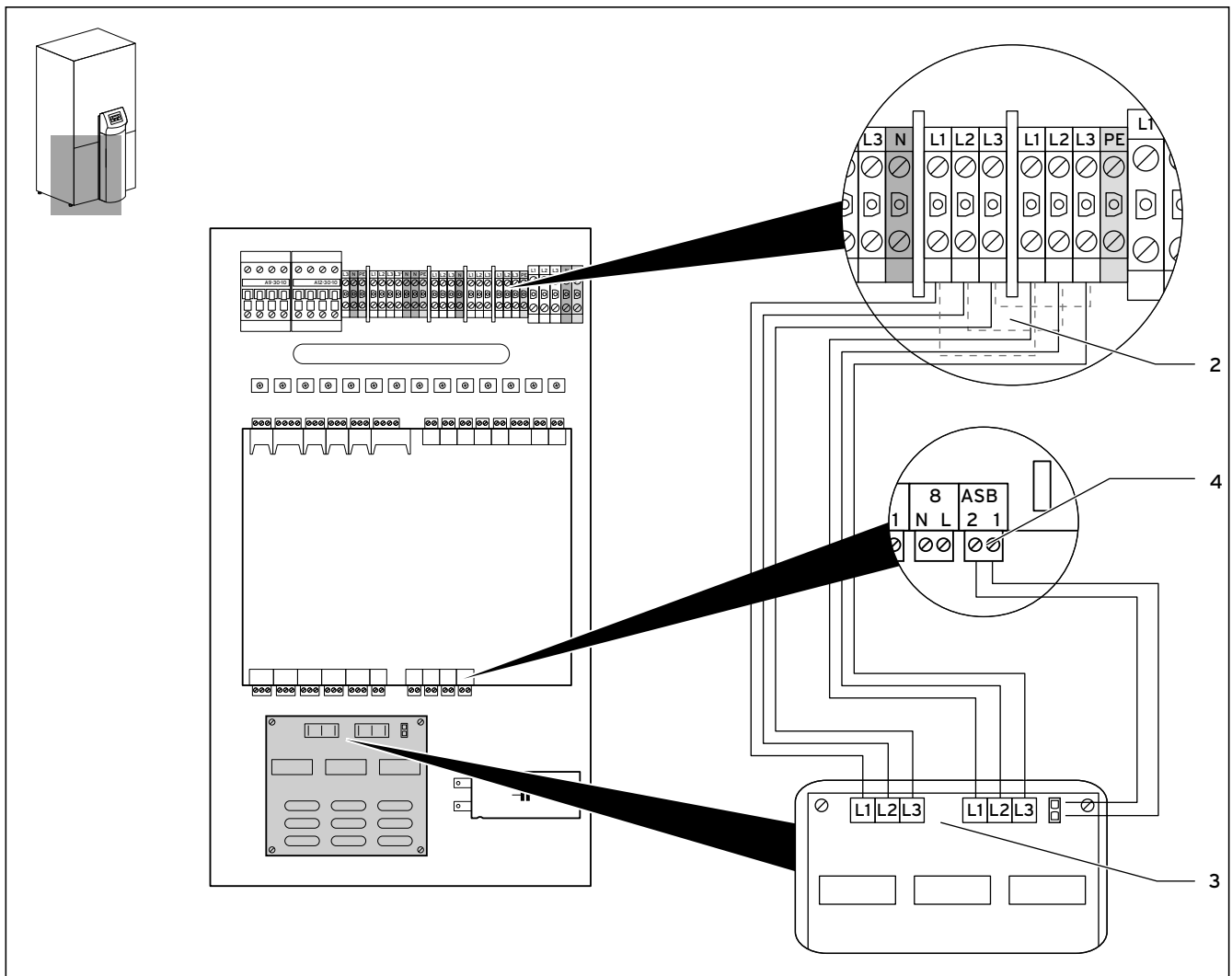
Abb. 4.2 Anschluss an geoTHERM VWL
