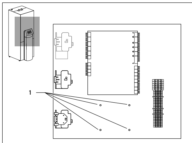
Fig. 4.5 Montering af monteringsskinner til geoTHERM VWS/VWW/VWL-S ..2 og VWS ..3
