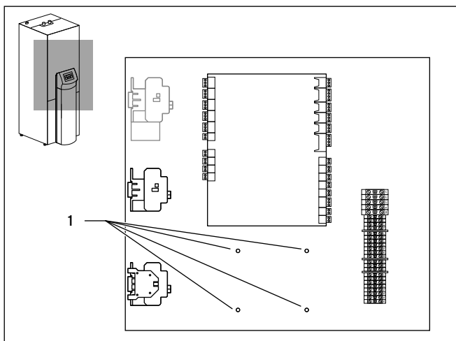
Fig. 4.5 Montera fästplattorna geoTHERM VWS/VWW/VWL-S ..2 och VWS ..3
