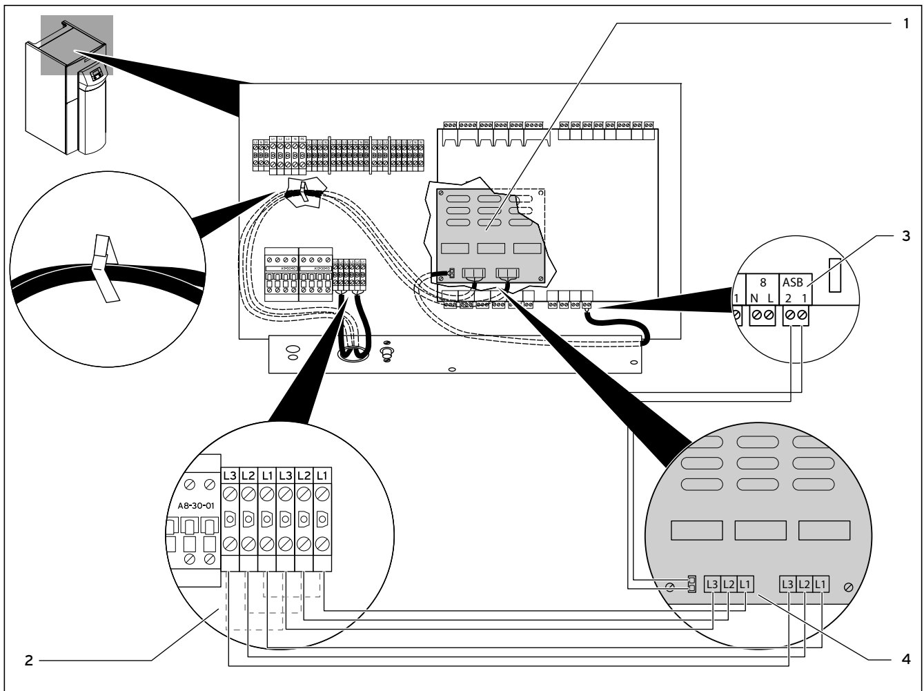
4.4 pav. Prijungimas prie geoTHERM VWS/VWW/VWL-S ..1 ir VWS ..4
