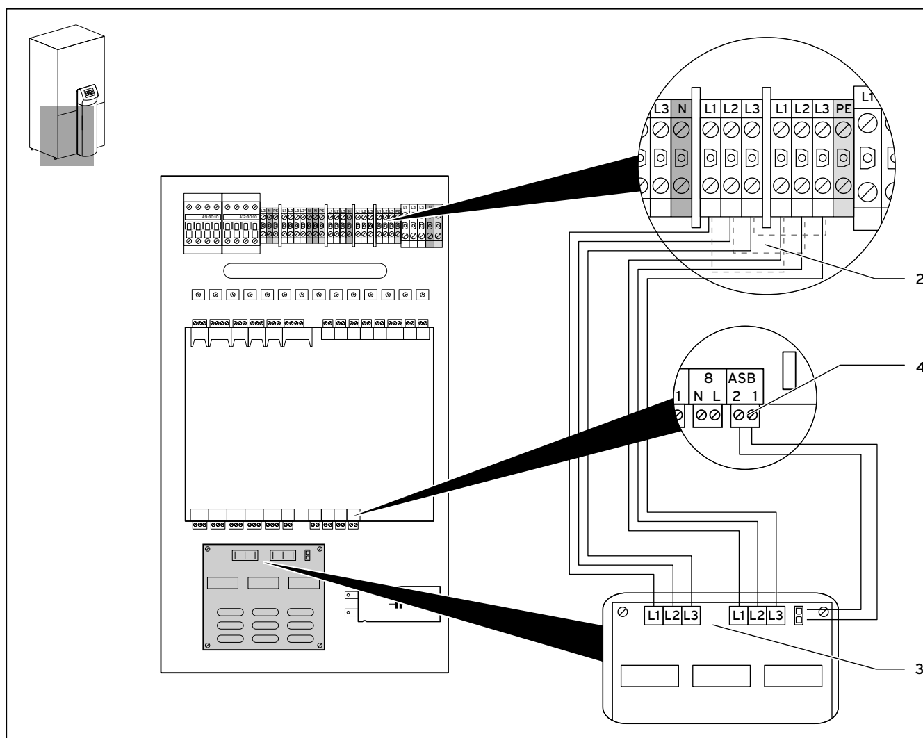
Rys. 4.2 Podłączenie do geoTHERM VWL
