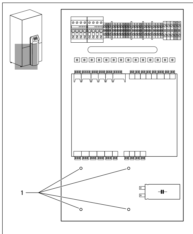
Fig. 4.1 Montering av fästplattor på geoTHERM VWL
