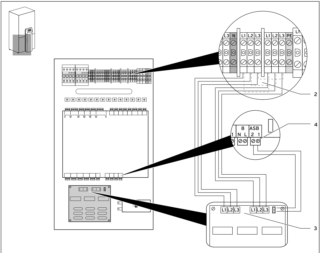
Kuva 4.2 Liitäntä geoTHERM VWL-lämpöpumppuun
