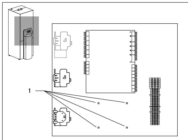
4.5. att. Fiksācijas pāreju montāža pie geoTHERM VWS/VWW/ VWL-S ..2 un VWS ..3
