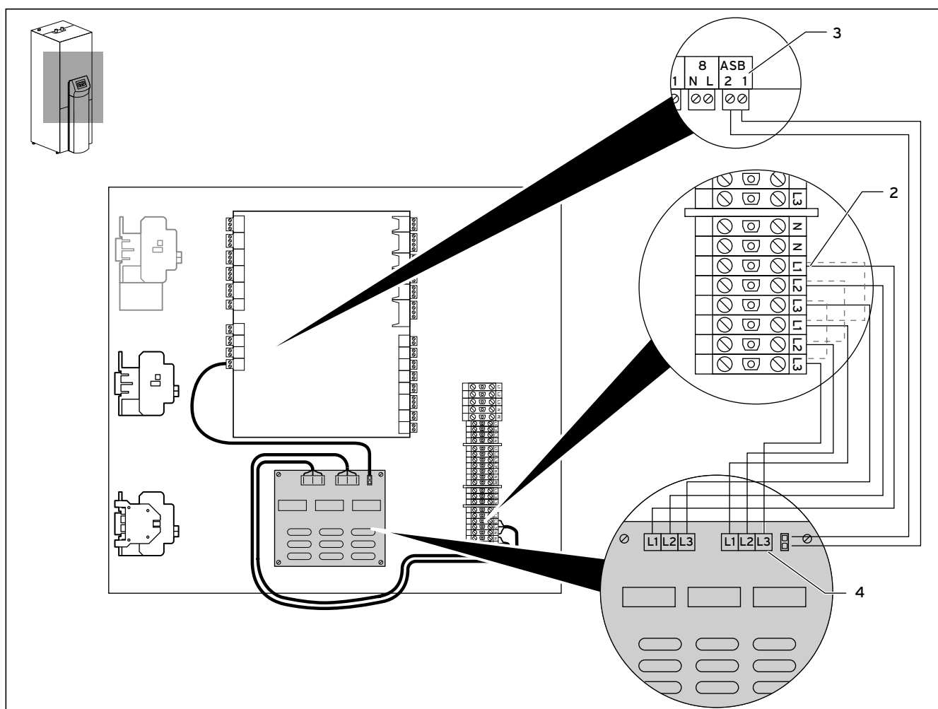
Fig. 4.6 Tilkobling til geoTHERM VWS/VWW/VWL-S ..2 og VWS ..3
