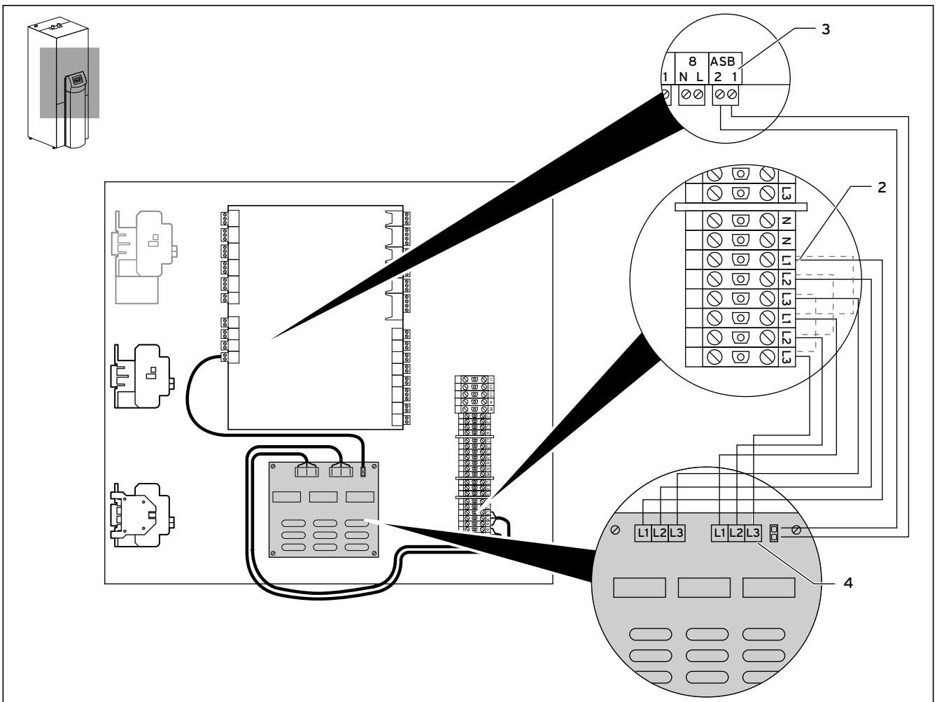
Joon. 4.6 Ühendamine geoTHERM VWS/VWW/VWL-S ..2 ja VWS ..3 külge
