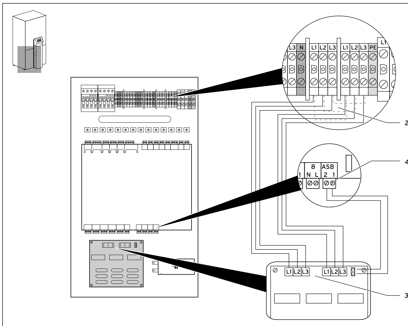
Fig. 4.2 Tilkobling til geoTHERM VWL
