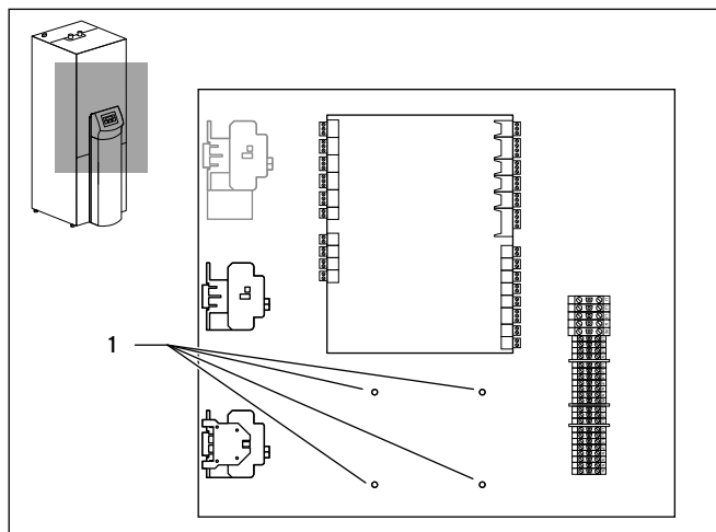
Rys. 4.5 Montaż wsporników mocujących w geoTHERM VWS/VWW/VWL-S ..2 i VWS ..3
