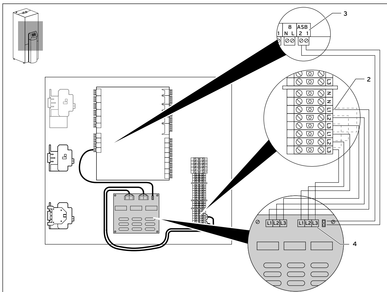
Fig. 4.6 Raccordement à geoTHERM VWS/VWW/VWL-S ..2 et VWS ..3
