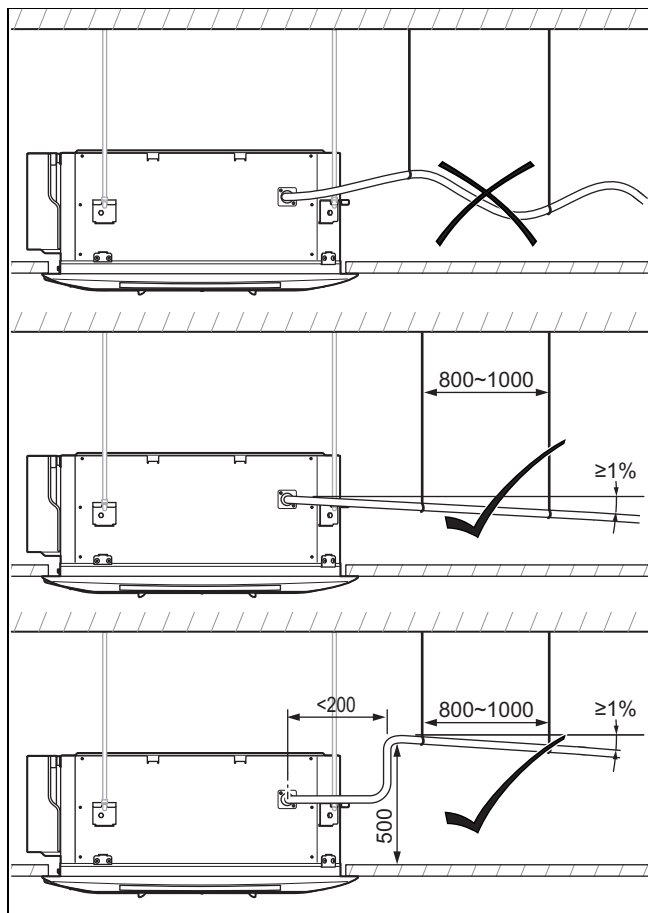
Postavljanje cijevi kondenzata od unutarnje jedinice kazete.
