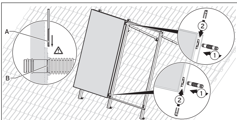
Abb. 5.22 Hydraulischen Verbinder anbringen
