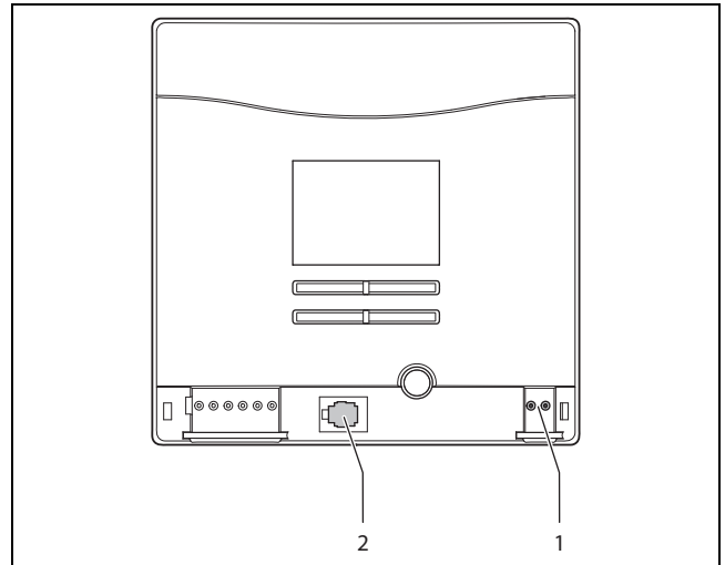
1 eBUS-Anschluss 2 Serviceanschluss
