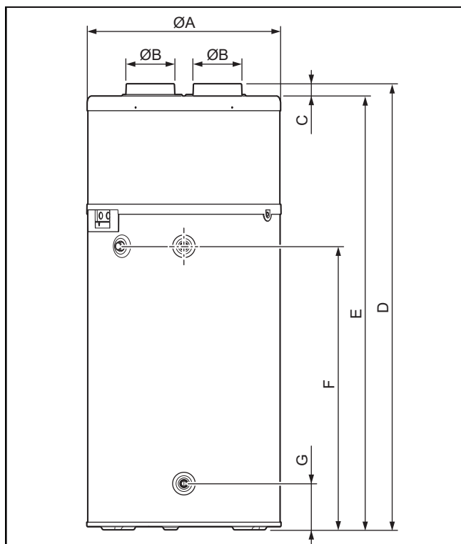
Geräteabmessungen und Anschlussmaße
