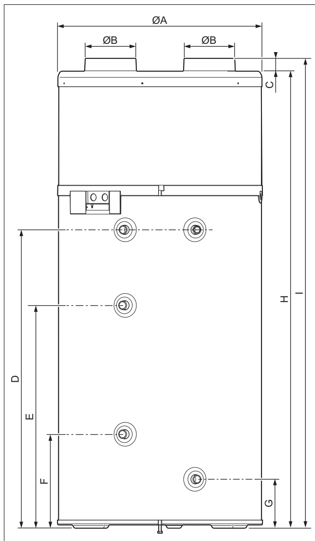
Geräteabmessungen und Anschlussmaße bei 200 und 270 l
