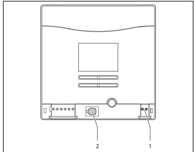
1 eBUS-Anschluss 2 Serviceanschluss
