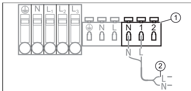
1 Steuerrelais
