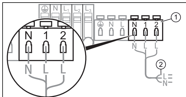
1 Steuerrelais
