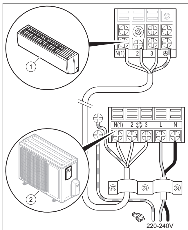
1 Unutarnja jedinica.
