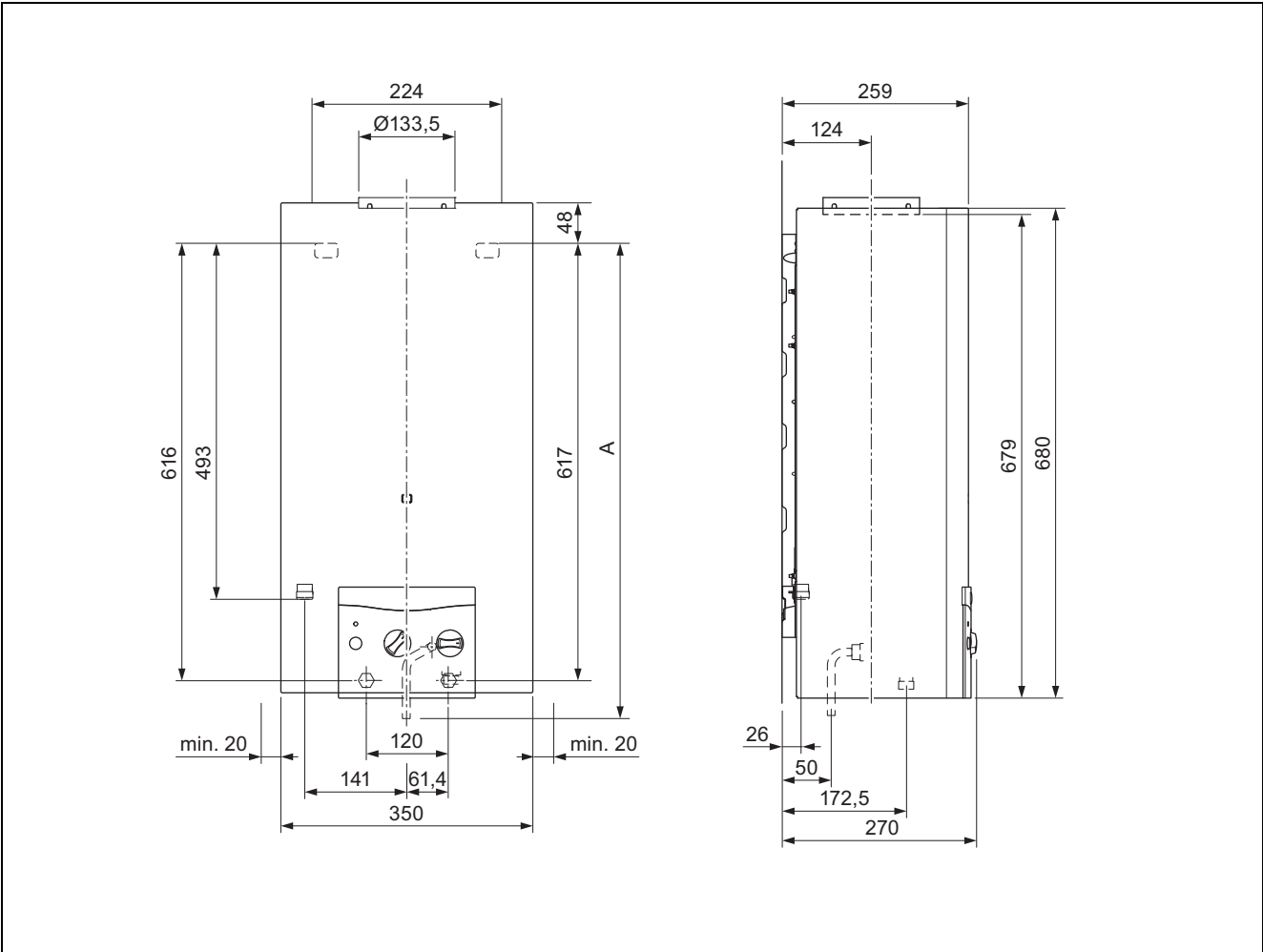
Hauteur, cote A
