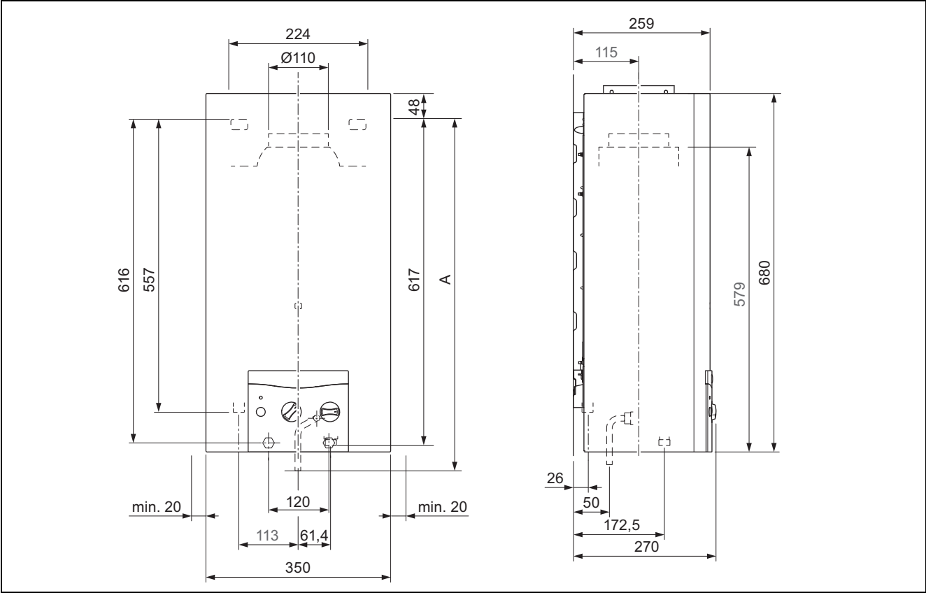
Hauteur, cote A
