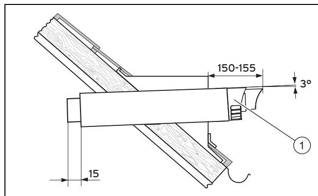
2 Entfernte Installation
