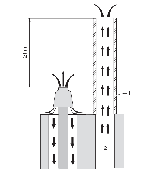
1 Schornsteinaufsatz 2 Rauchgas
