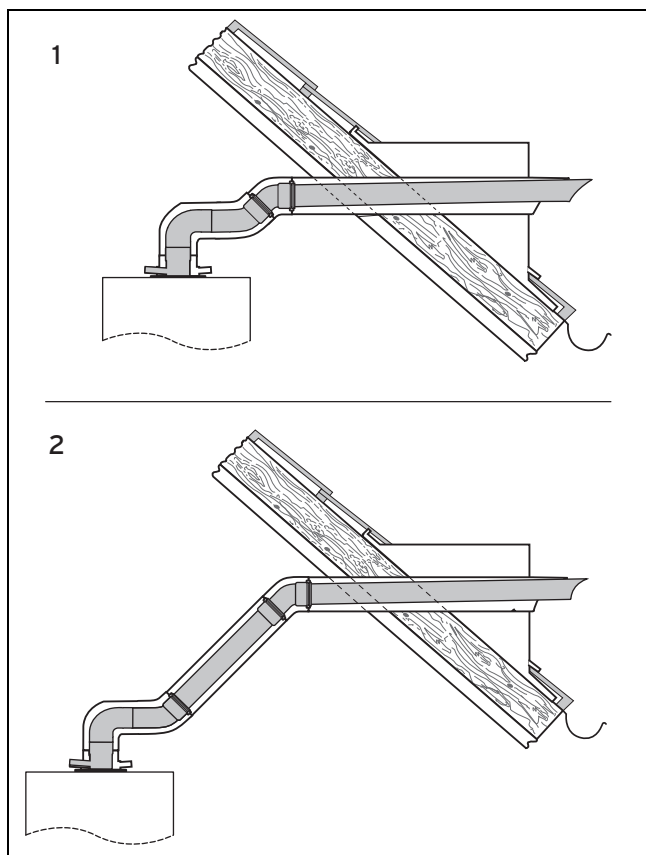
1 Direkte Installation
