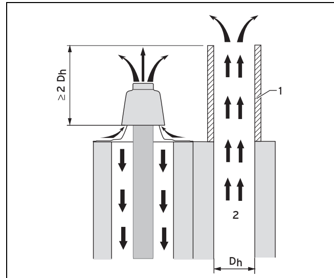
1 Schornsteinaufsatz 2 Rauchgas
