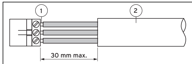
1 Anschlussdrähte 2 Isolierung
