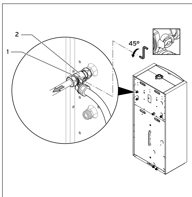
7.16 Absperrreinrichtung am Speichervorlauf in 45°-Position bringen
