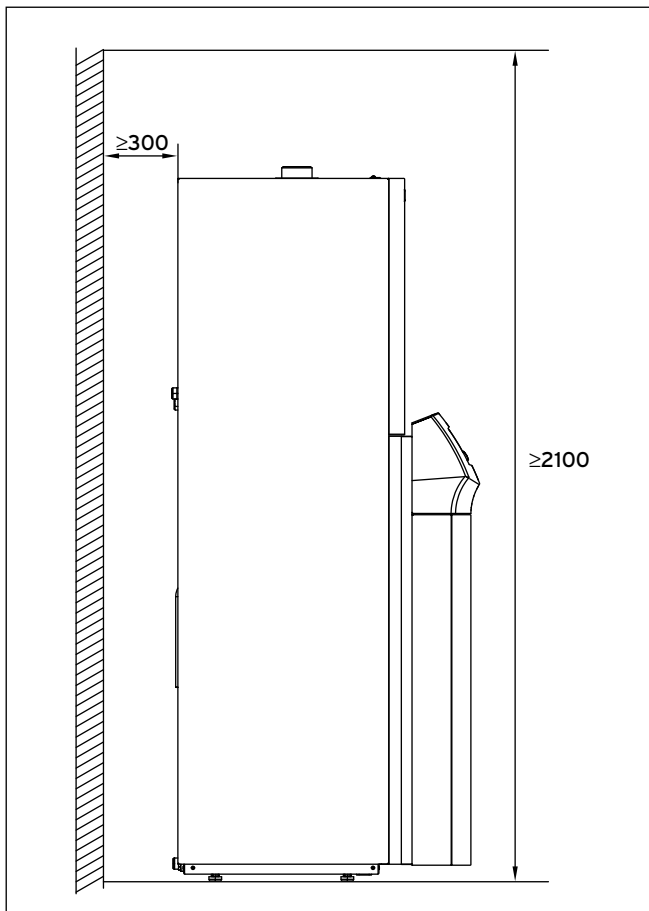
4.1 Mindestabstände (Maße in mm)
