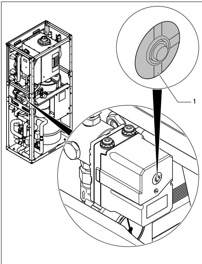
7.23 Werkseinstellung „Desorption Bypass“ des Vorrangumschaltventils
