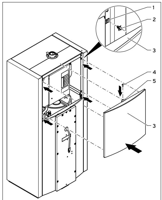
7.35 Obere Frontverkleidung montieren
