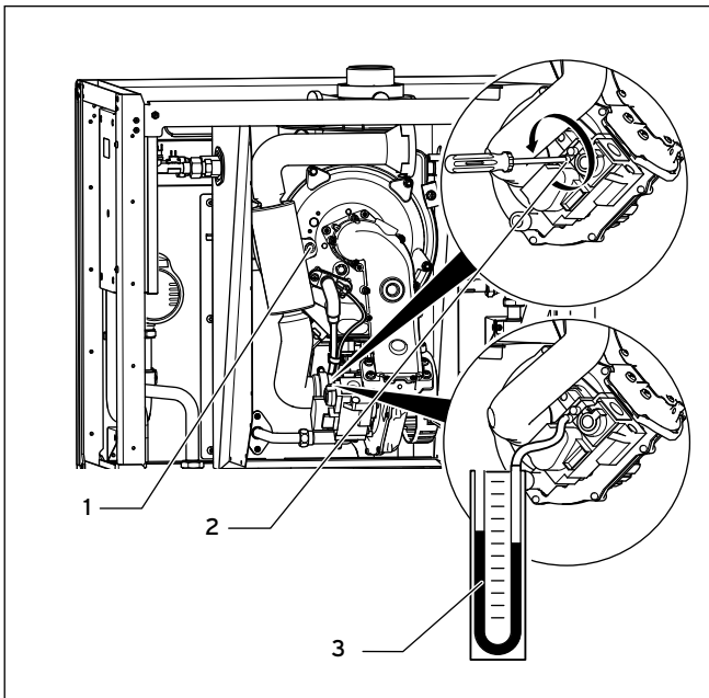
8.4 Anschlussdruck (Gasfließdruck) messen
