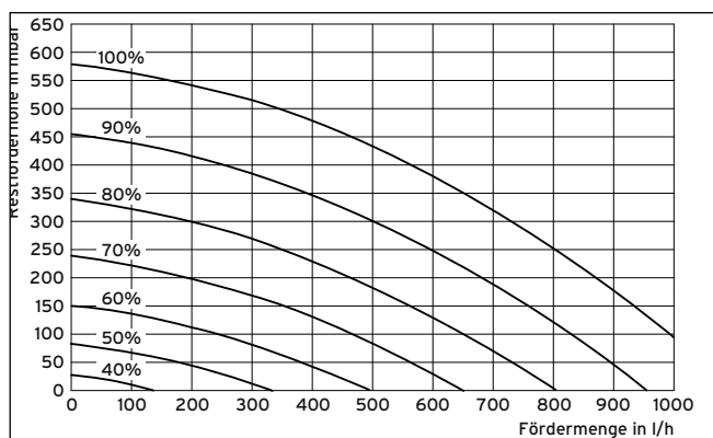
16.3 Pumpendiagramm Solekreis SHU
