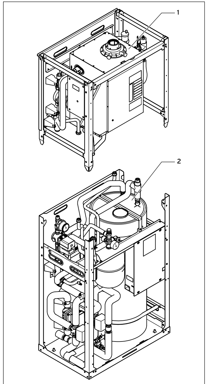
4.9 Brennwerteinheit und Zeolith-Einheit
