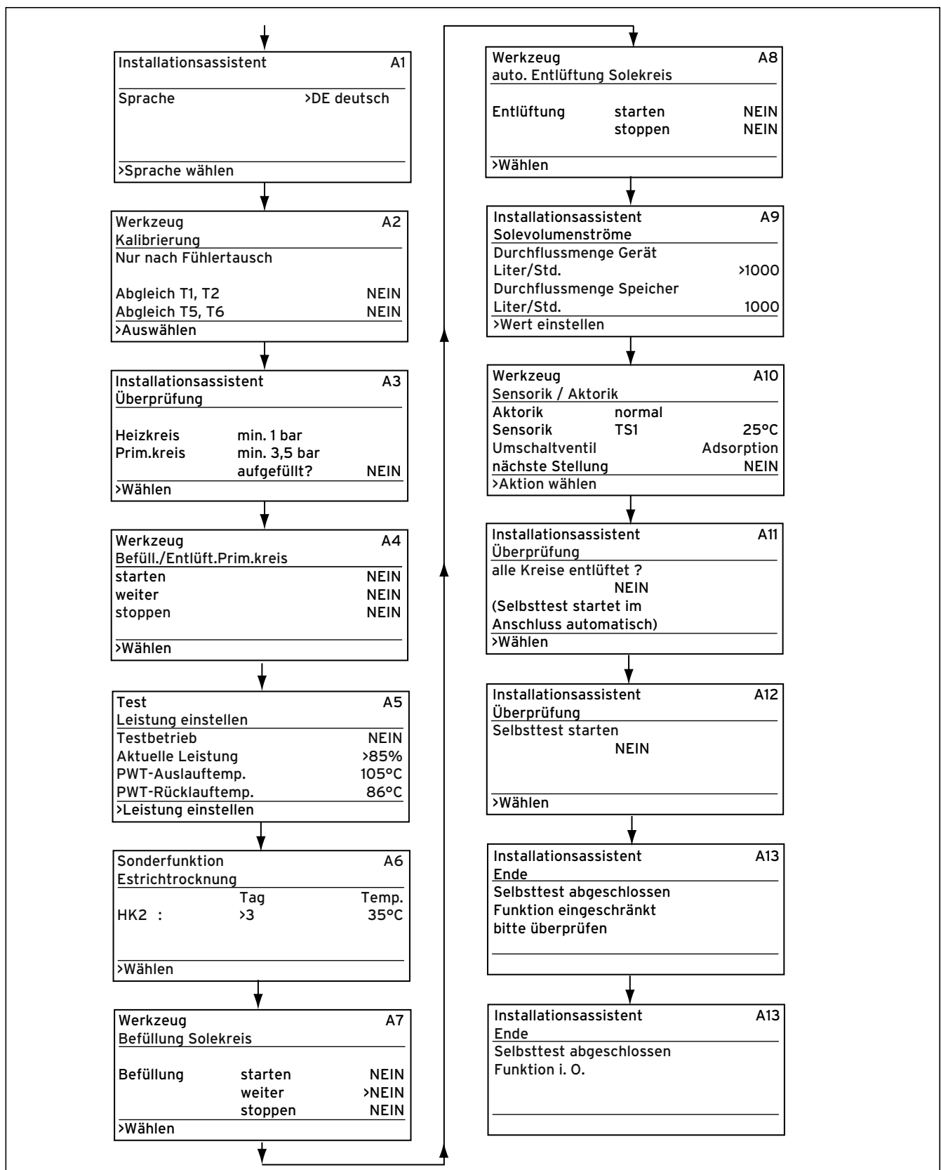
10.4 Displays in der Codeebene (Fortsetzung)
