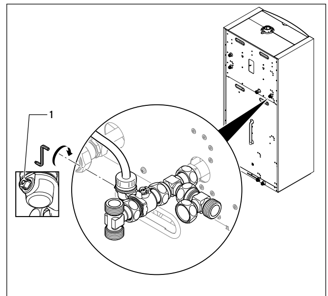
7.11 Wartungshahn am Heizungsrücklauf öffnen
