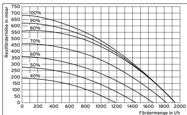
16.1 Pumpendiagramm Heizkreis
