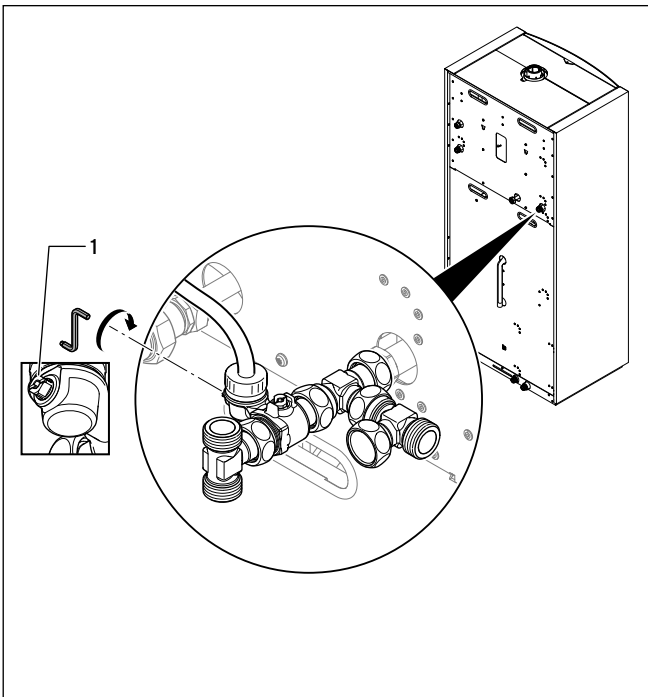
7.6 Wartungshahn am Heizungsrücklauf öffnen
