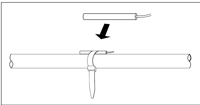
6.5 Standardfühler VR 11 als Ertragsfühler
