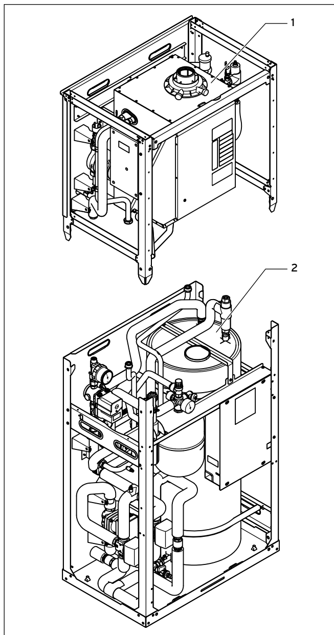
3.7 Brennwerteinheit (oben) und Zeolith-Einheit (unten)
