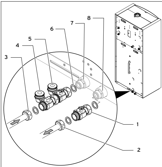
5.4 Solareintritt und Solaraustritt montieren
