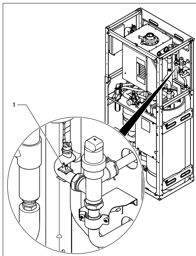
4.11 Elektrische Verbindung trennen
