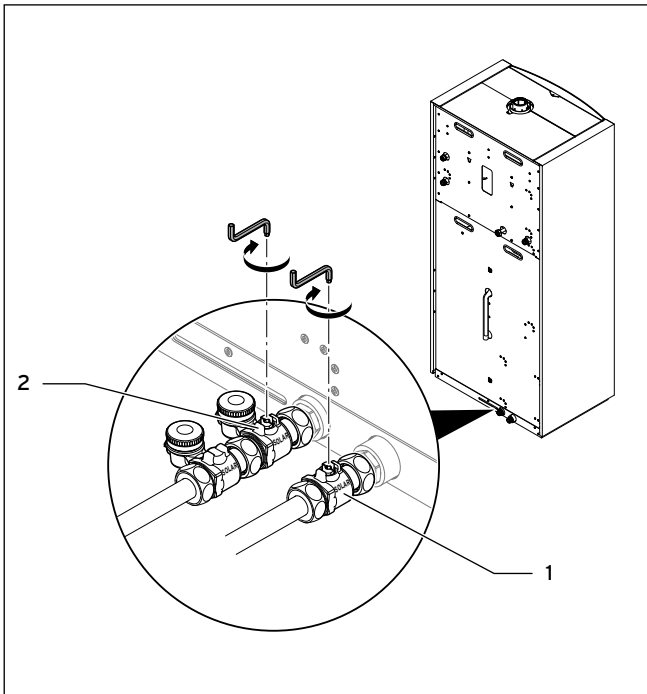
7.25 Absperrhähne an der zeoTHERM schließen
