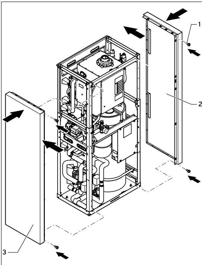
7.32 Seitenteile montieren
