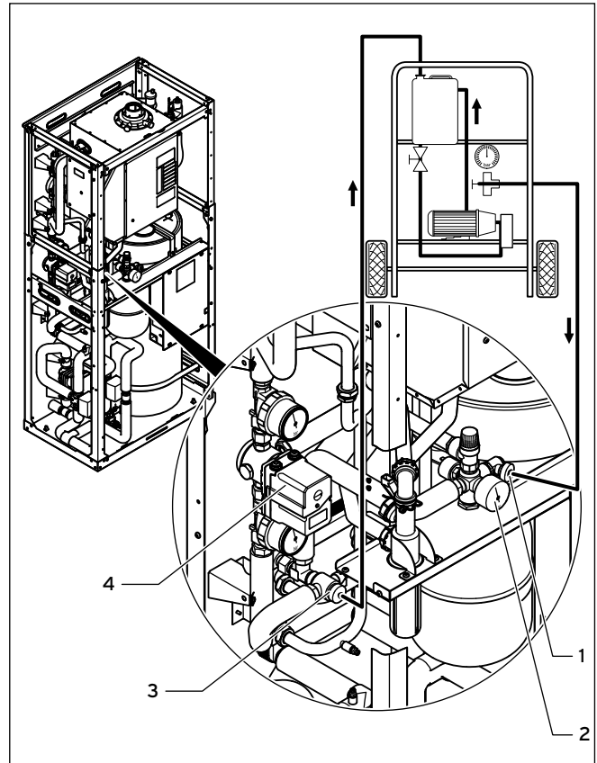
7.22 Primärkreis befüllen hier: mit Befüll-Trolley (Art.-Nr. 0020042548)
