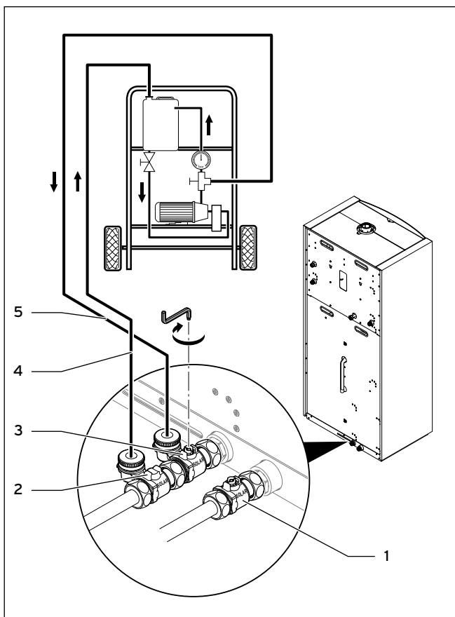
7.29 Befüllschläuche und Wartungshähne an der zeoTHERM
