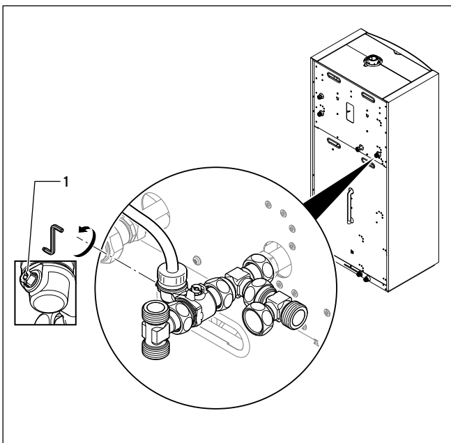
7.20 Wartungshahn am Heizungsrücklauf schließen
