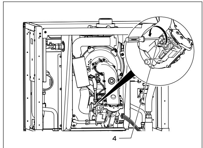
8.5 Luftzahl einstellen
