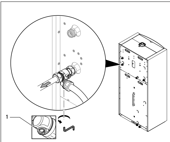
7.13 Wartungshahn am Heizungsanlauf schließen
