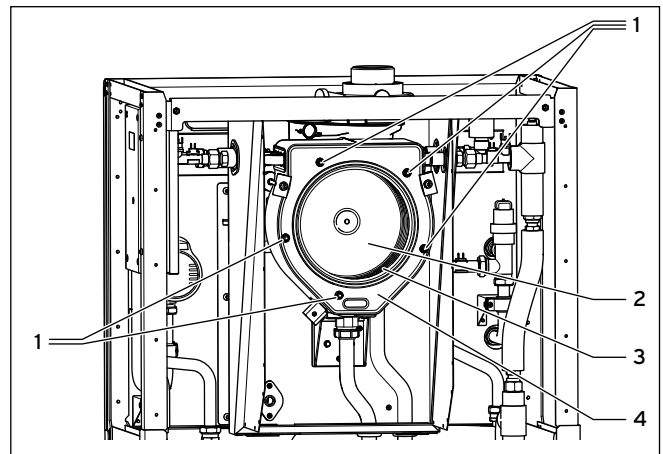
11.3 Integral-Kondensations-Wärmetauscher reinigen
