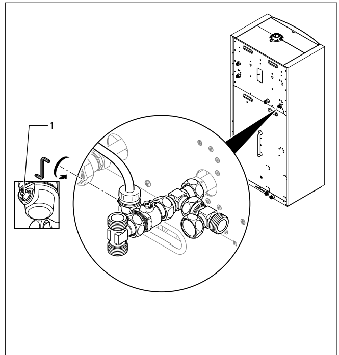
7.8 Wartungshahn am Heizungsrücklauf schließen
