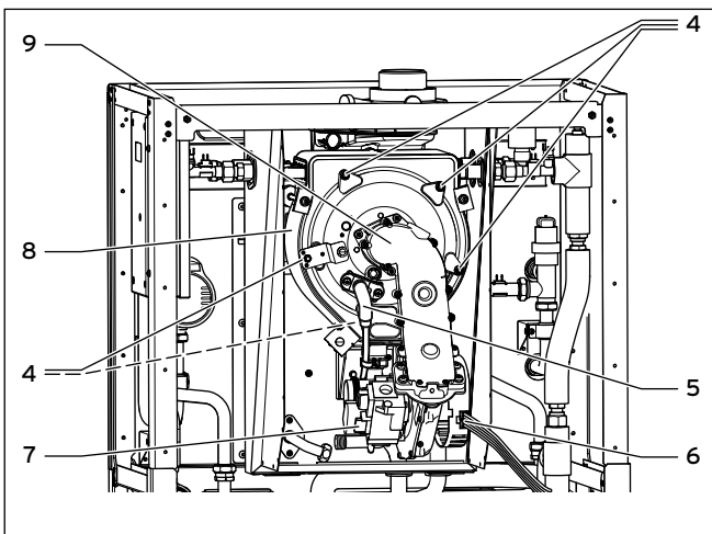
11.2 Thermo-Kompaktmodul ausbauen
