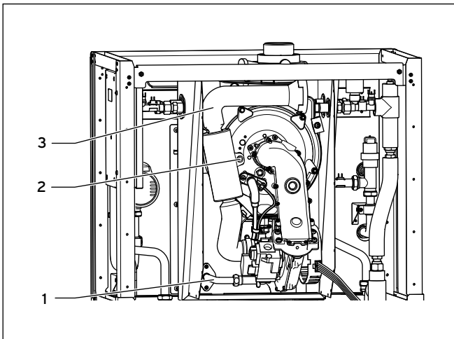
11.1 Luftansaugrohr ausbauen
