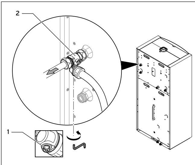
7.19 Wartungshahn am Speichervorlauf schließen
