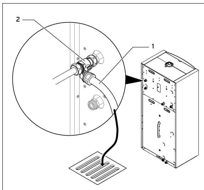
7.15 Spülschlauch am Speichervorlauf anbringen
