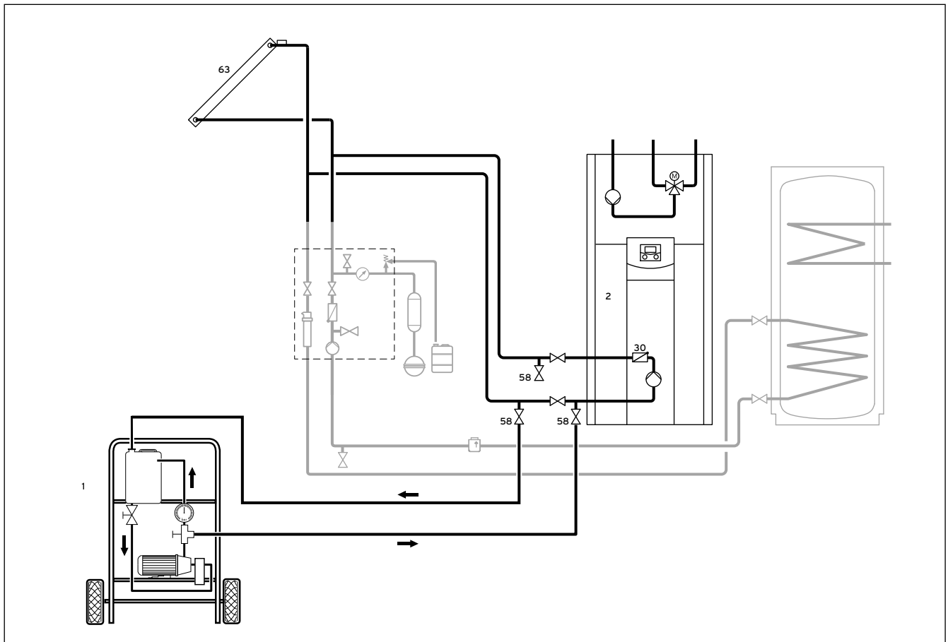
7.28 Schema: Solekreis und Befülleinrichtung Beispiel hier: Befüllung zeoTHERM/Kollektor
