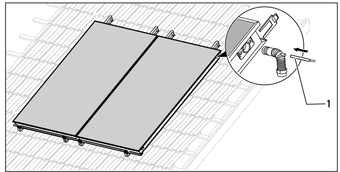
6.6 Kollektorfühler in den Hydraulikanschluss eines Kollektors einfügen (Beispiel Flachkollektoren)
