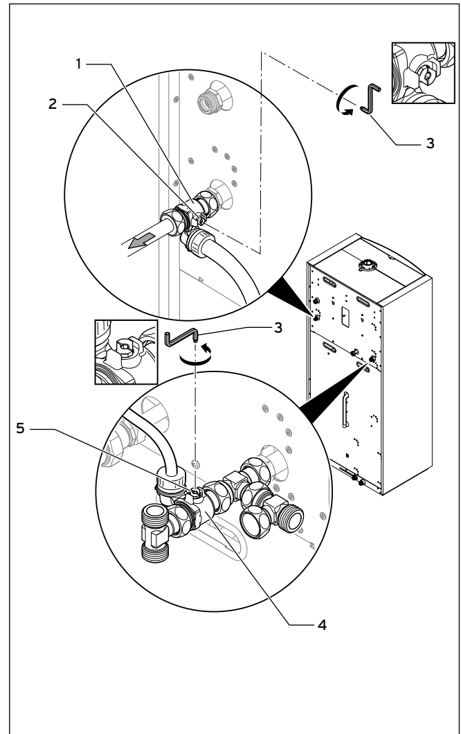
7.14 Absperrvorrichtungen am Heizungsanlauf und Heizungsrücklauf öffnen
