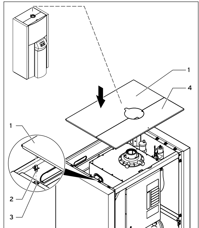
7.33 Obere Abdeckung montieren
