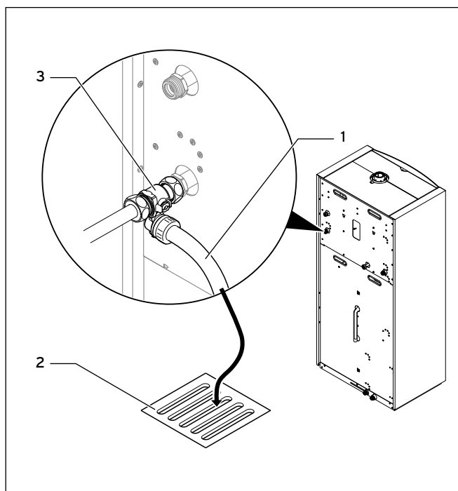
7.4 Spülschlauch am Heizungsanlauf
