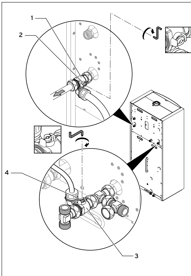
7.9 Absperreinrichtungen am Heizungsanlauf und Heizungs- rücklauf schließen
