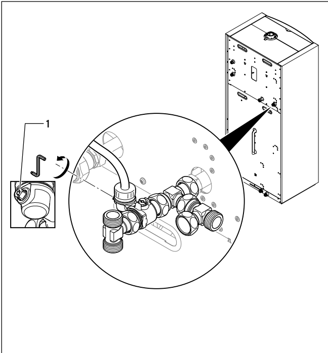
7.12 Wartungshahn am Heizungsrücklauf schließen
