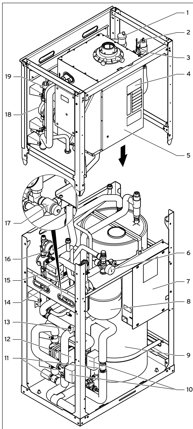
3.8 Komponenten der zeoTHERM
