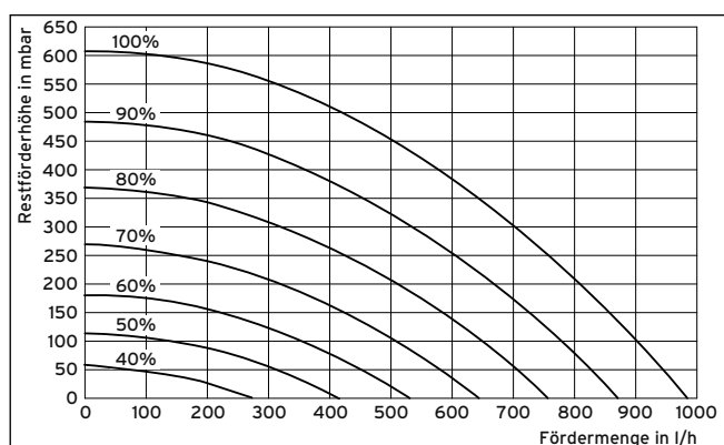
16.2 Pumpendiagramm Solekreis Adsorption
