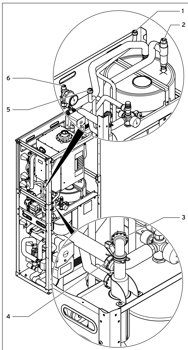
4.10 Rohre und Schläuche trennen
