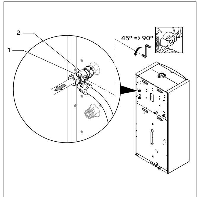
7.21 Absperreinrichtung am Speichervorlauf öffnen
