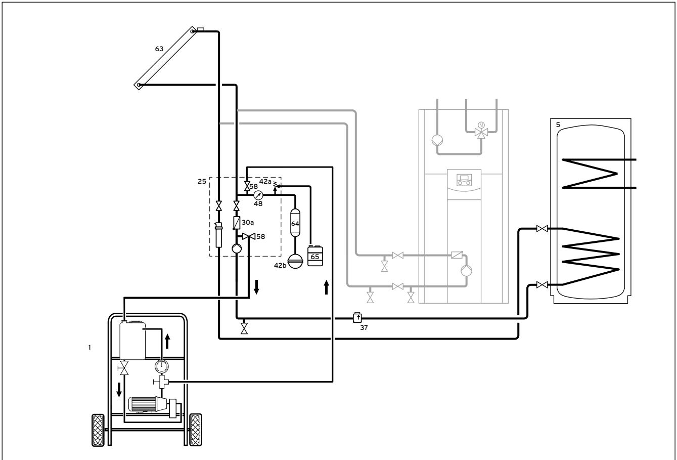
7.24 Schema: Solekreis und Befüllereinrichtung Beispiel hier: Befüllung Speicher/Kollektor
