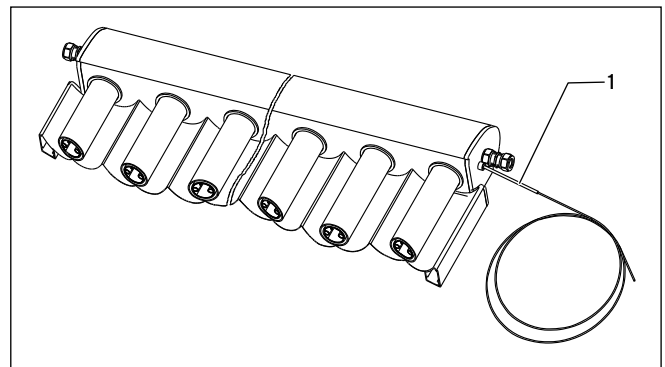
6.7 Kollektorfühler in den Hydraulikanschluss eines Kollektors einfügen (Beispiel Röhrenkollektoren)
