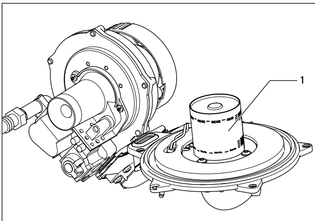
11.4 Brenner prüfen
