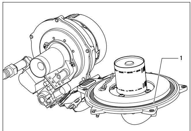
11.5 Brenntürdichtung ersetzen
