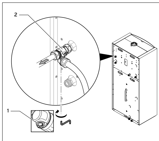
7.17 Wartungshahn am Speichervorlauf öffnen
