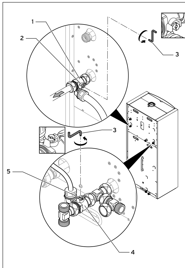
7.5 Absperreinrichtungen am Heizungsanlauf und Heizungs-rücklauf öffnen
