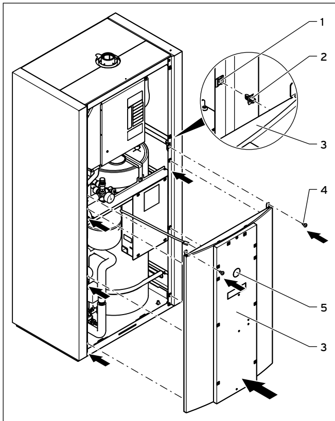
7.34 Untere Frontverkleidung montieren
