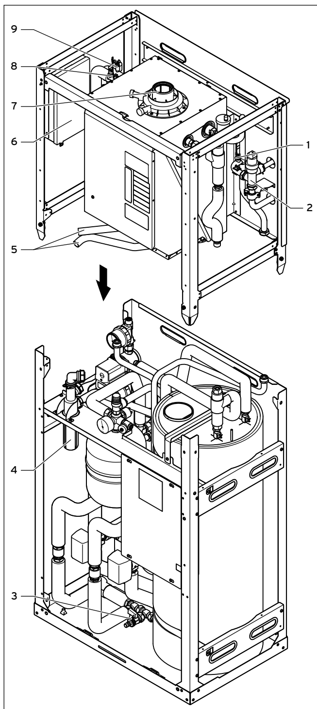
3.9 Komponenten der zeoTHERM
