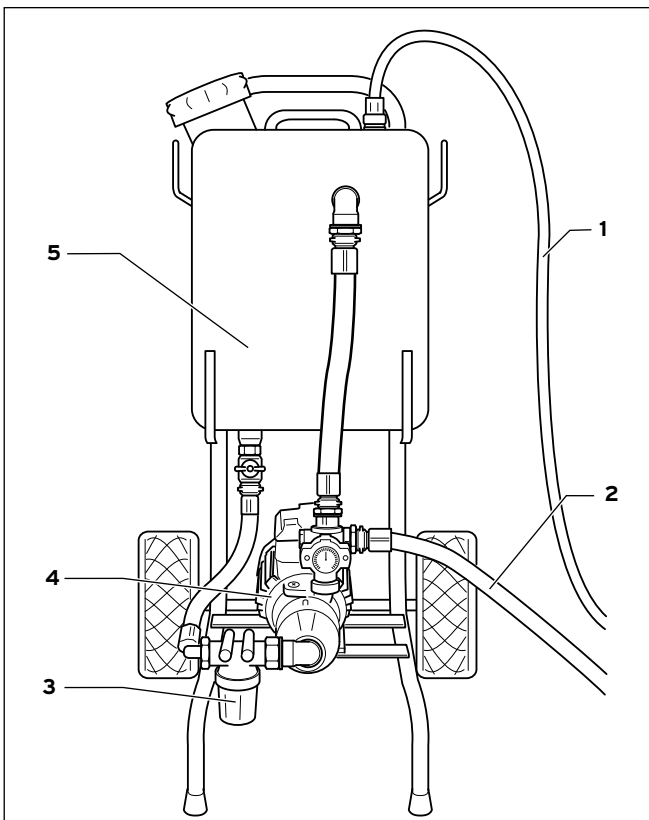
7.27 Anschlüsse an der Befüllanlage Beispiel: hier Befüll-Trolley (Art.-Nr. 0020042548)
