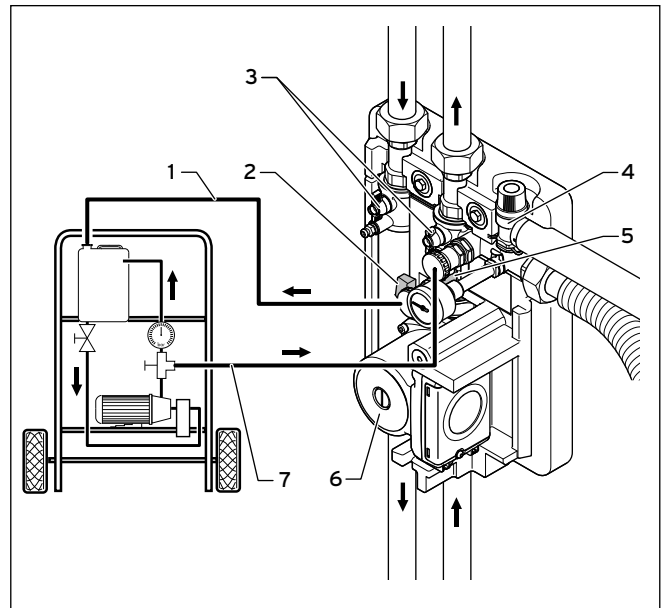
7.26 Befüllschläuche an der Solarstation montieren
