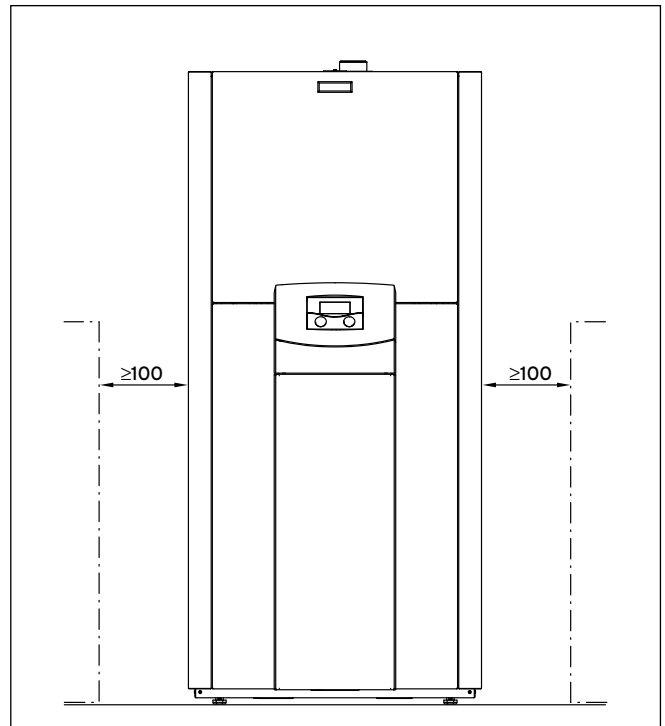
4.2 Mindestabstände (Maße in mm)
