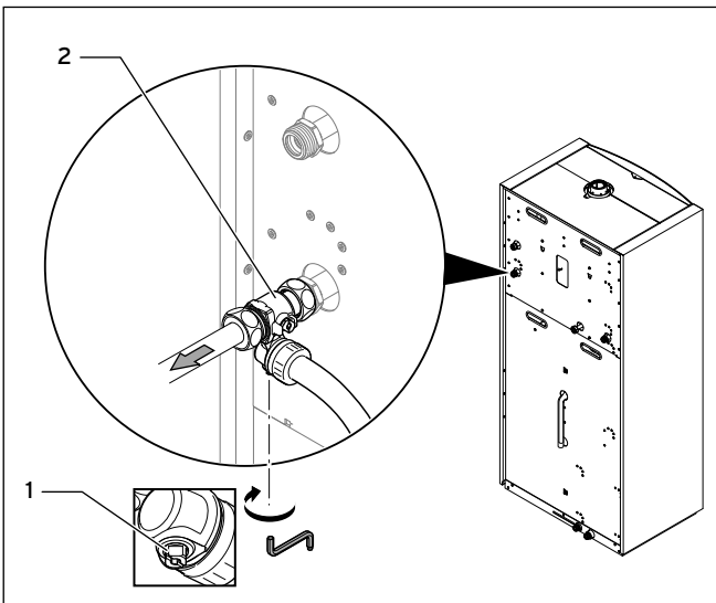
7.7 Wartungshahn am Heizungsanlauf öffnen
