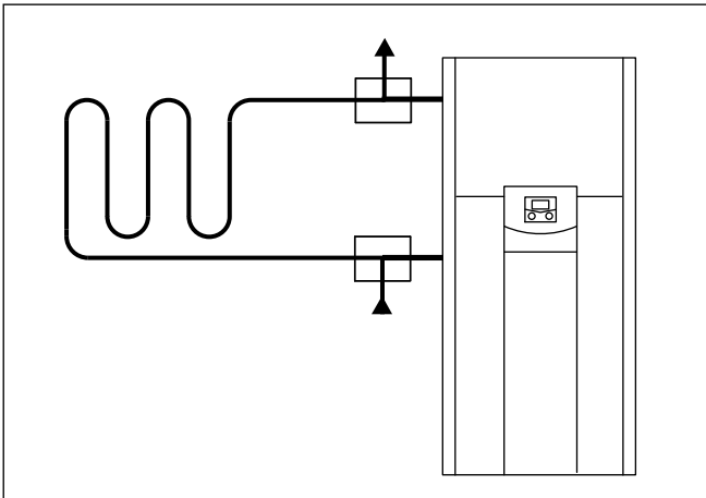
7.1 Schema Ventilstellungen am Heizungsvor- und -rücklauf beim Befüllen/Spülen des externen Heizkreises
