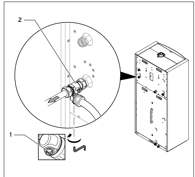
7.10 Wartungshahn am Heizungsanlauf öffnen
