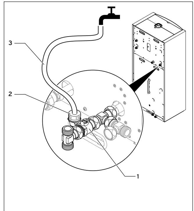
7.3 Wartungshahn im Heizungsrücklauf zum Befüllen nutzen
