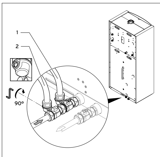
7.31 Wartungshahn schließen
