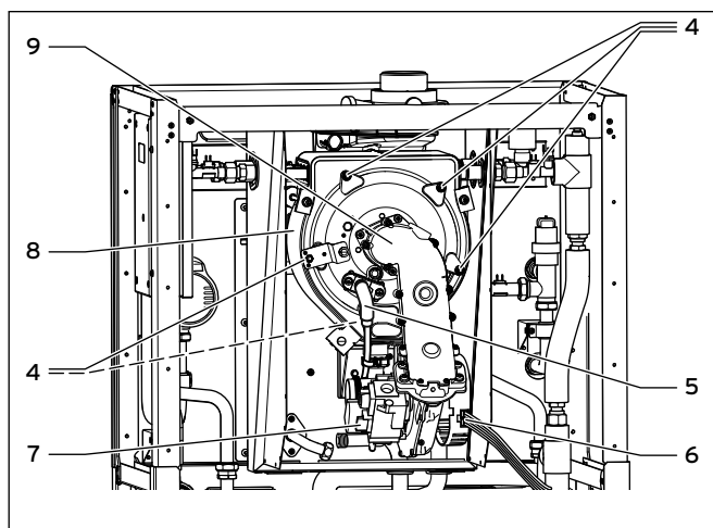
11.6 Thermo-Kompaktmodul einbauen
