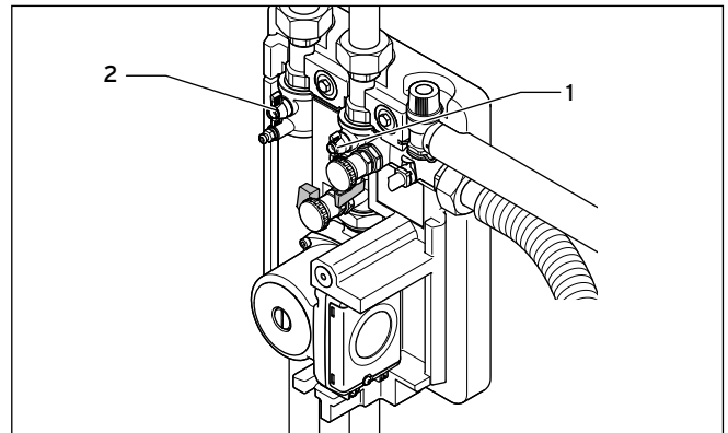
7.30 Vor- und Rücklauf an der Solarstation
