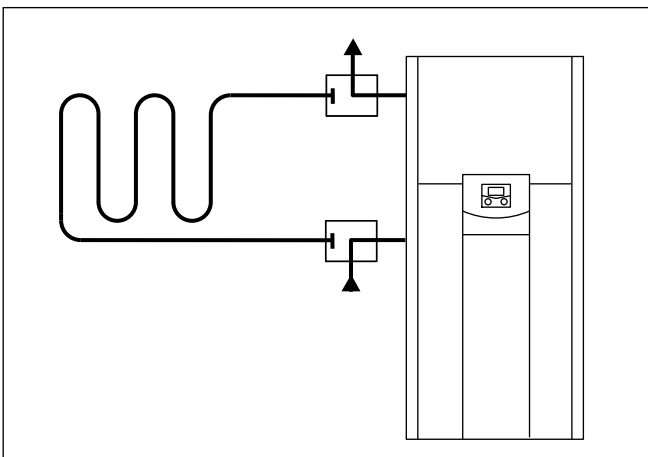
7.2 Schema Ventilstellungen am Heizungsvor- und -rücklauf beim Befüllen/Spülen des geräteinternen Heizkreises
