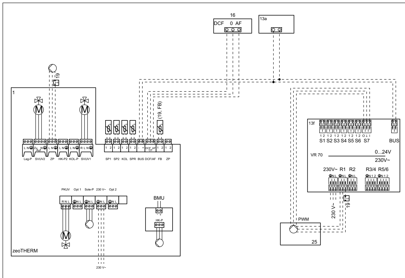
6.1 Leiterplatten Systemsteuerung und Solarstation VMS70 (mit Zirkulation)
