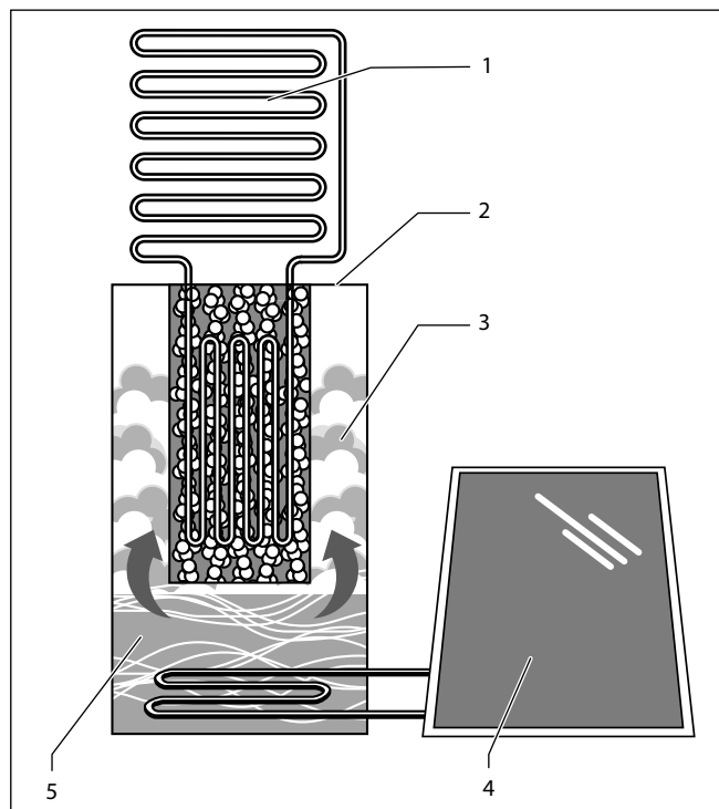
3.2 Befeuchtung des Zeolith
