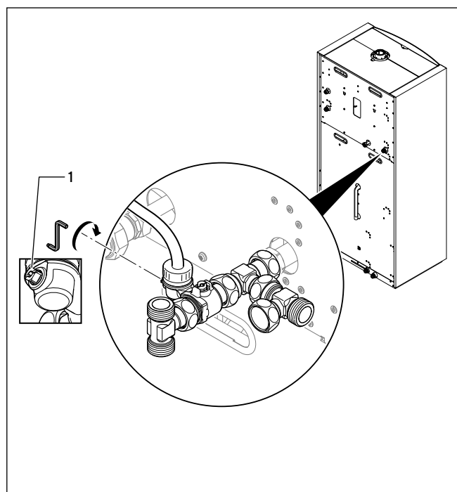
7.18 Wartungshahn am Heizungsrücklauf öffnen
