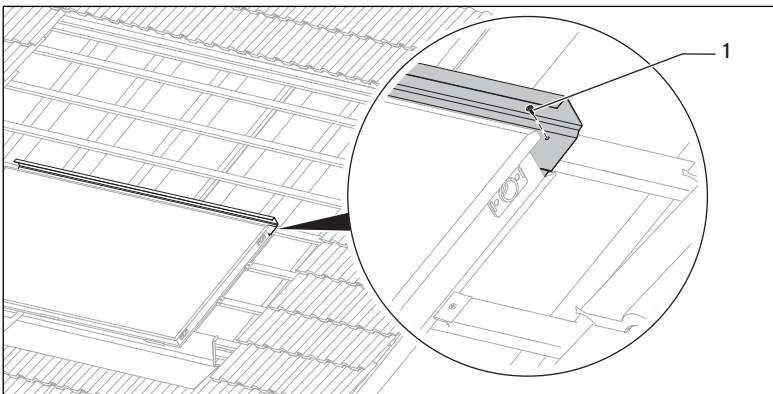
Abb. 5.16 Abstandhalter anschrauben
