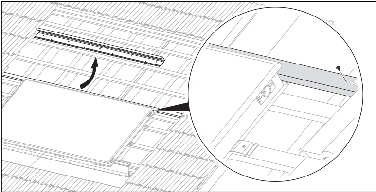
Abb. 5.15 Dachlatte anschrauben
