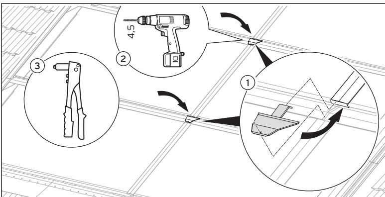
Abb. 5.29 Trapezbleche anbringen
