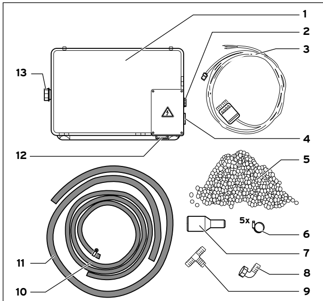
4.1 Lieferumfang der Neutralisationseinrichtung mit Förderpumpe
