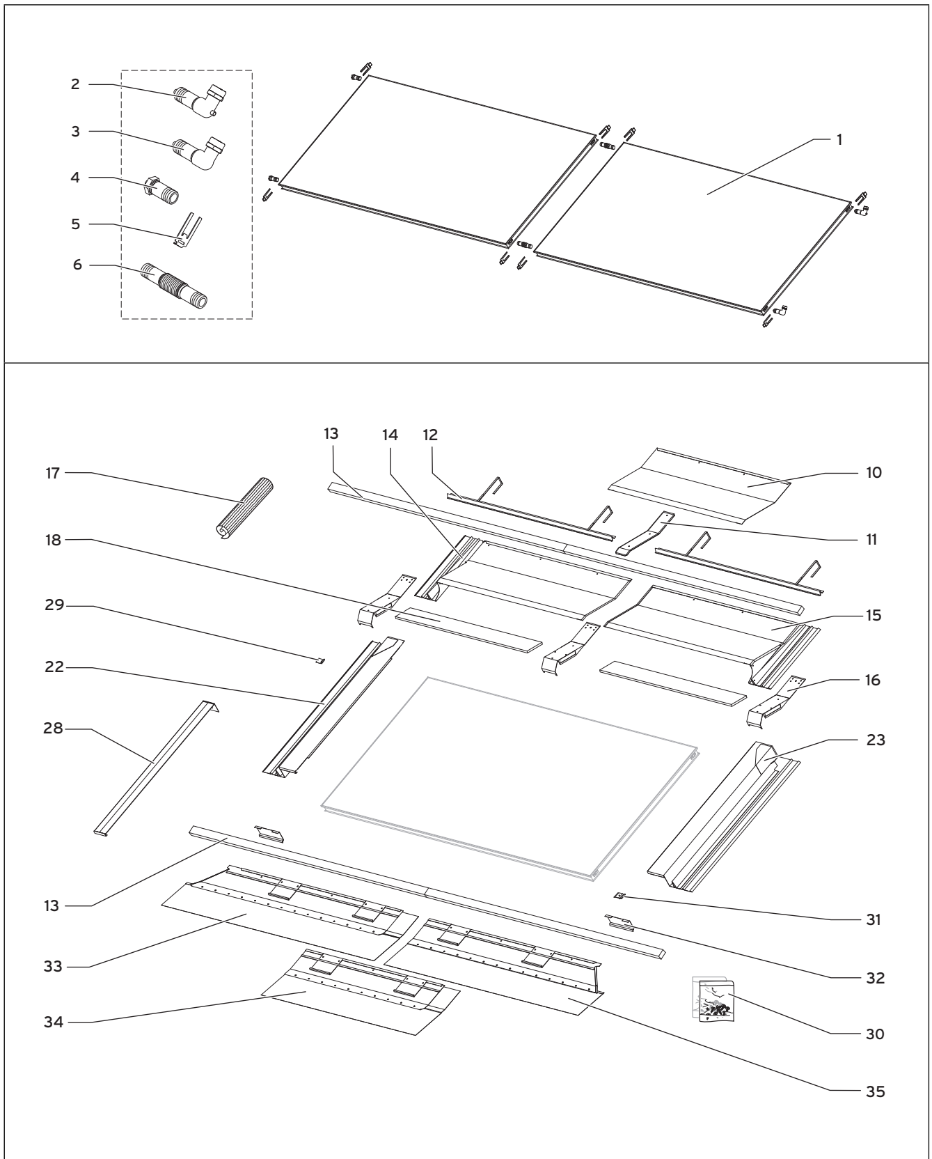
Abb. 5.5 Einbauset horizontaler Kollektor (VFK 145/2/155 H)
