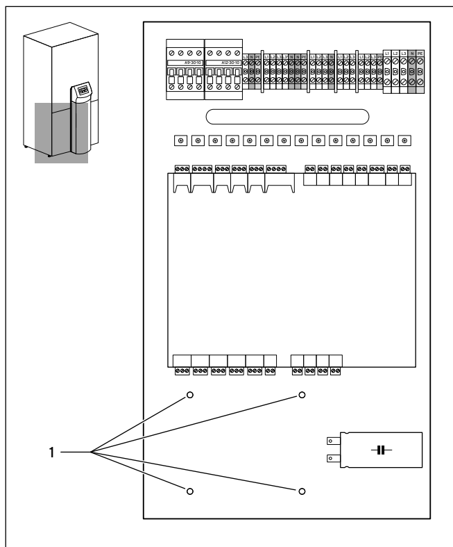
Fig. 4.1 Montering af monteringsstriker til geoTHERM VWL
