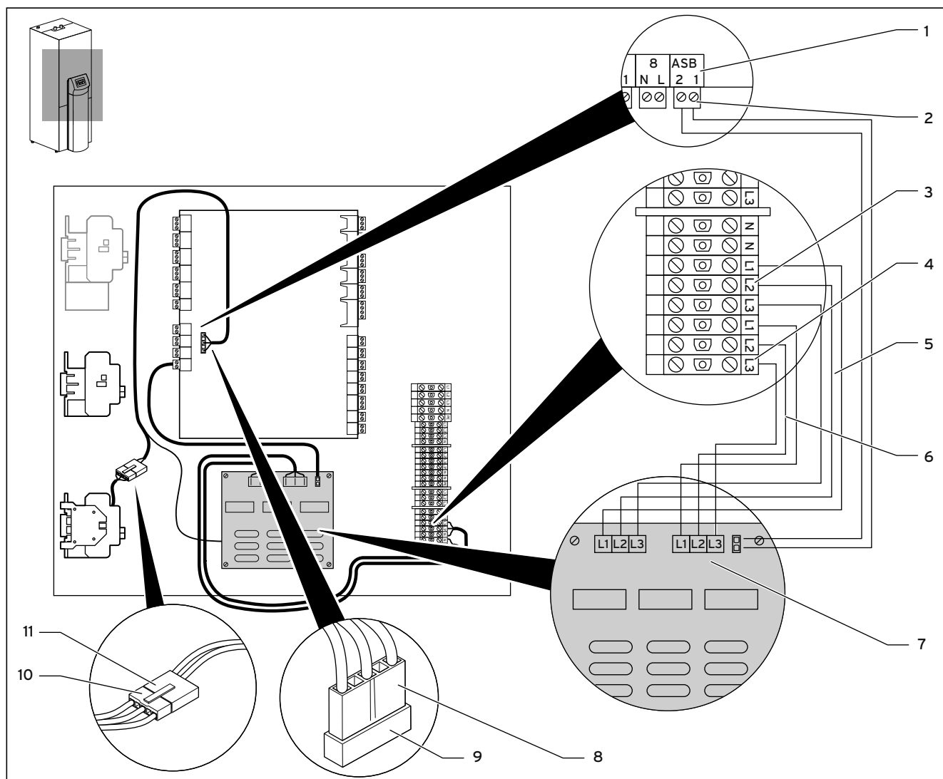
Fig. 4.9 Tilslutning af monteringskinner til geoTHERM VWS/VWL-S ..2 og VWS ..3
