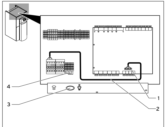
Kuva 4.5 Kompressorin vaihentarkkailun purkaminen VWS/VWW/VWL-S ..1 und VWS ..4
