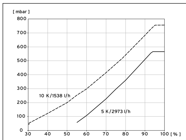
9.10 Diagramm Leistungsoptimierung Heizkreispumpe VWS 171/3
