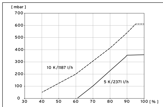
9.9 Diagramm Leistungsoptimierung Heizkreispumpe VWS 141/3
