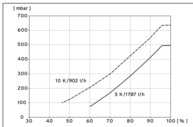
9.8 Diagramm Leistungsoptimierung Heizkreispumpe VWS 101/3
