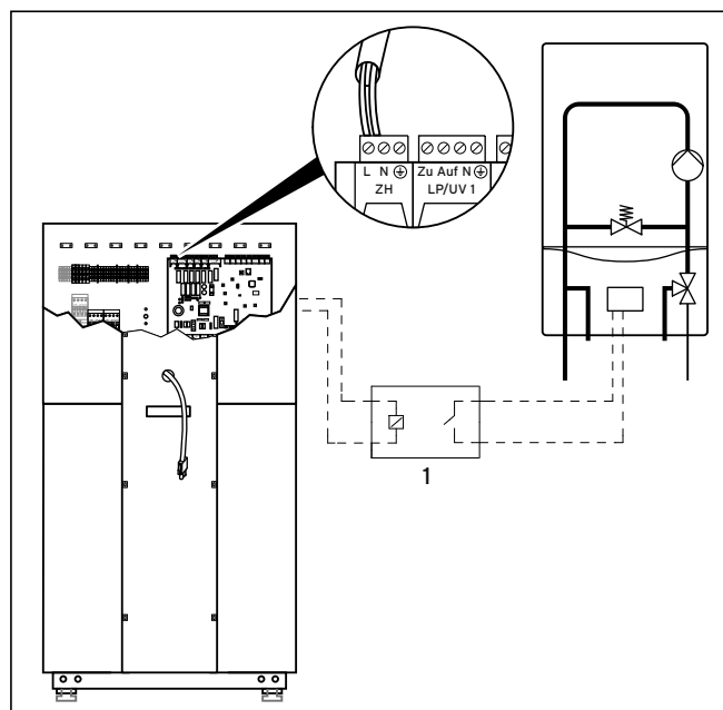
7.17 Heizgerät ohne eBUS-Schnittstelle anschließen
