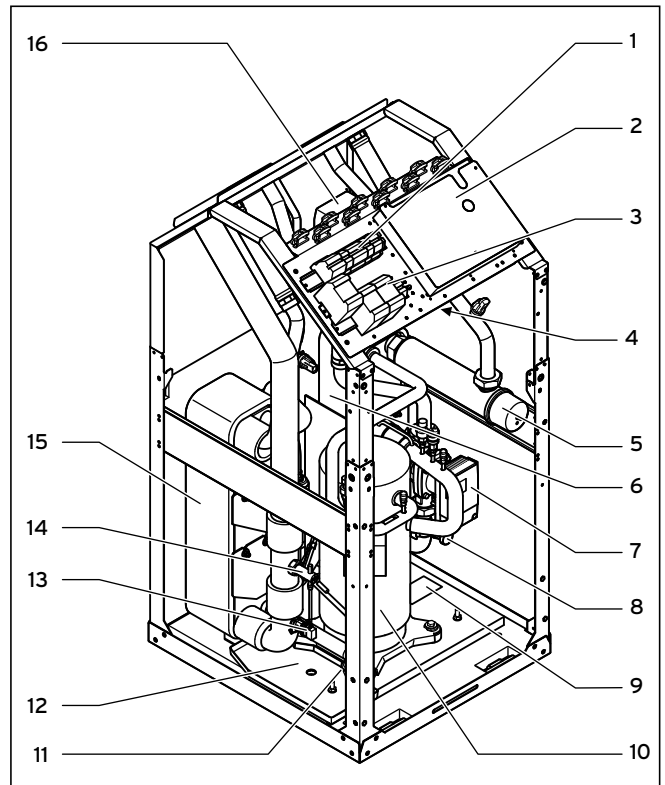
3.6 Vorderansicht geöffnet (VWW)
