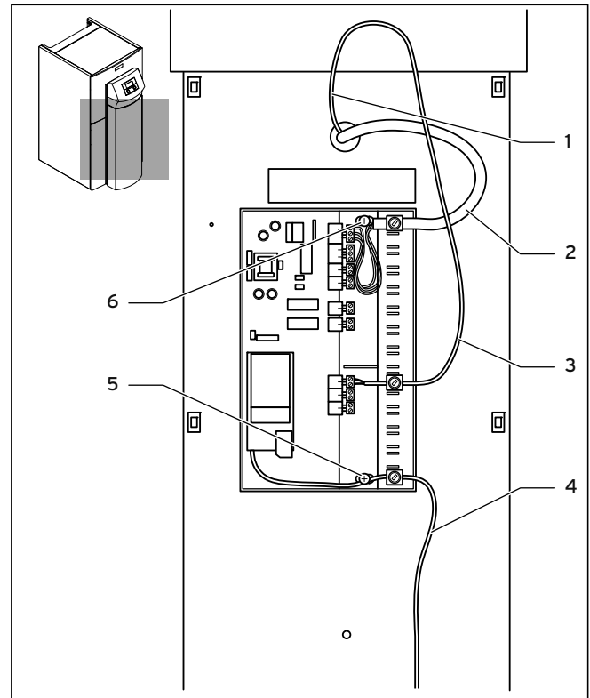
7.24 vrnetDIALOG installieren
