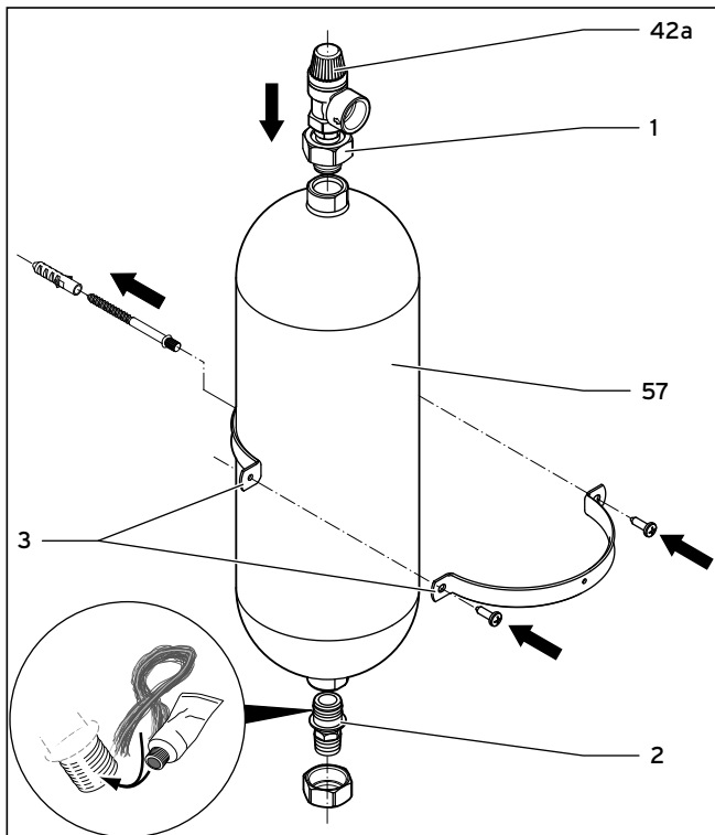
5.8 Sole-Ausgleichsbehälter montieren
