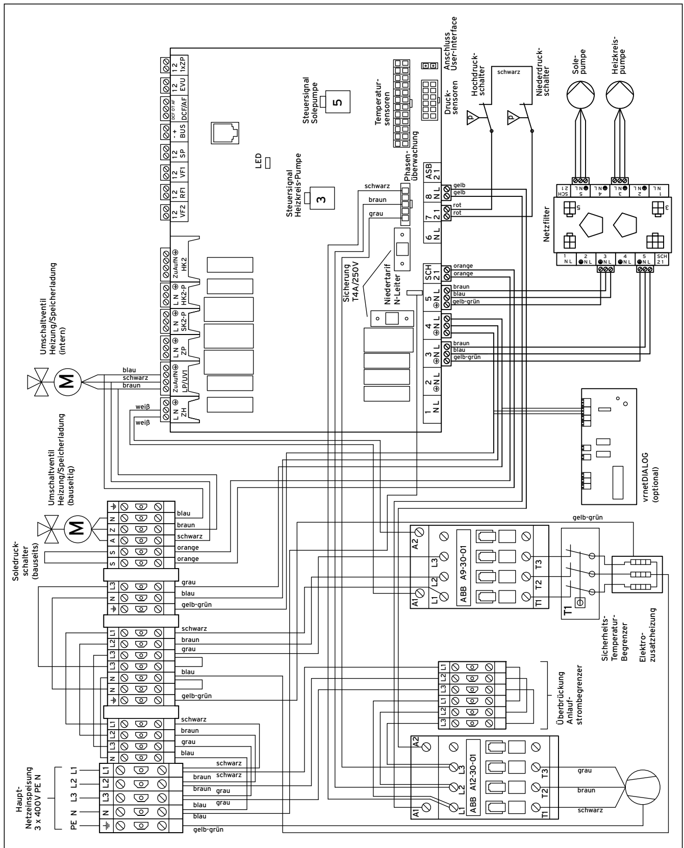
17.4 Stromlaufplan VWS 171/3
