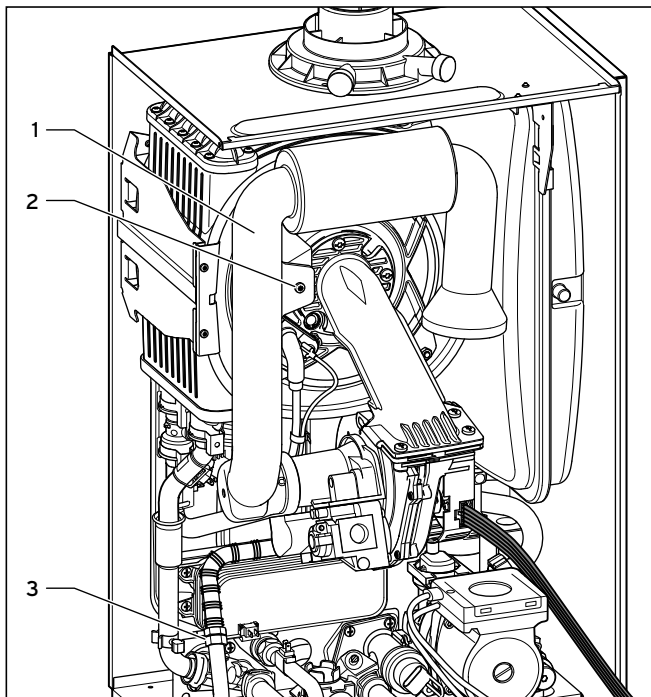
Abb. 8.1 Luftansaugrohr ausbauen
