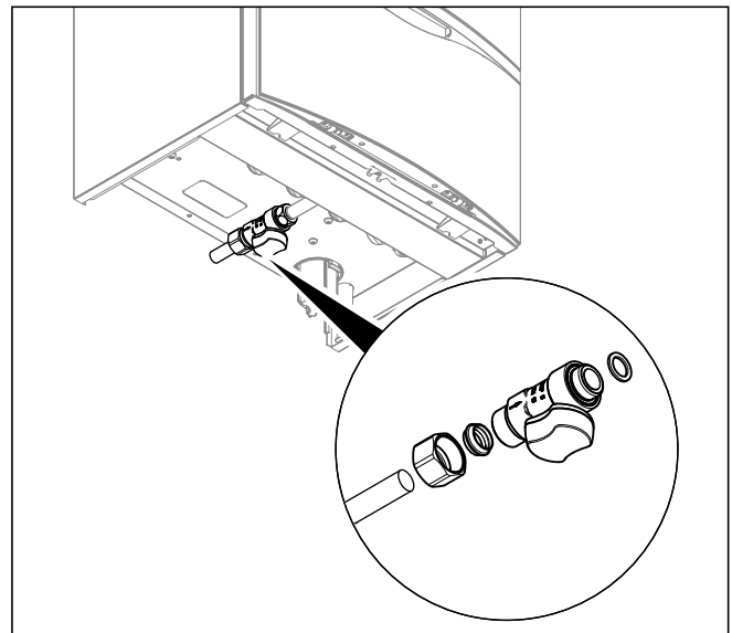
Abb. 5.1 Gasanschluss
