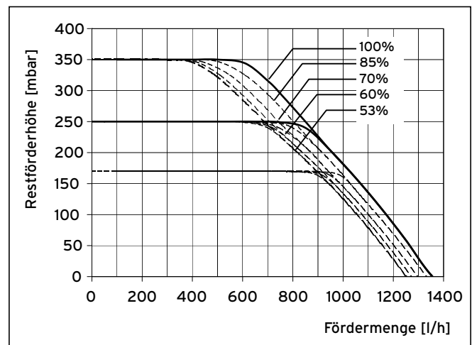
Abb. 7.2 Pumpenkennlinie ecoTEC plus VCW 196/3 - 5 A
