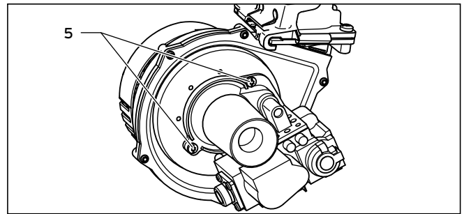
Abb 10.3 Verschraubung Gasarmatur/Gebläse
