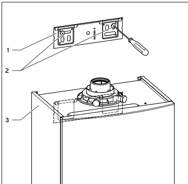
Abb. 4.3 Gerät aufhängen
