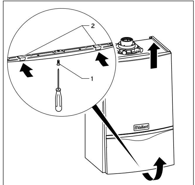
Abb. 4.4 Frontverkleidung abnehmen
