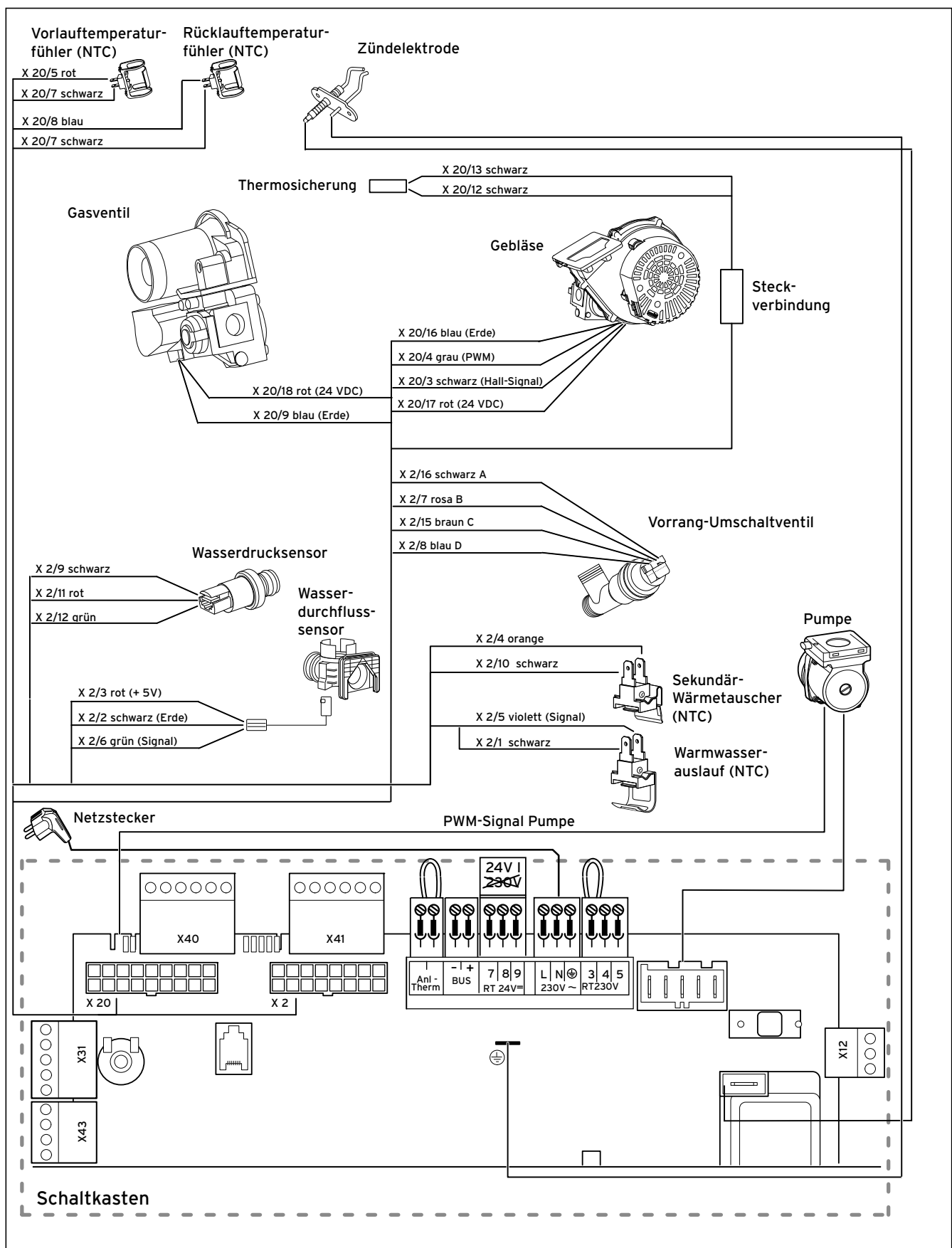
Abb. 5.11 Verdrahtungsplan
