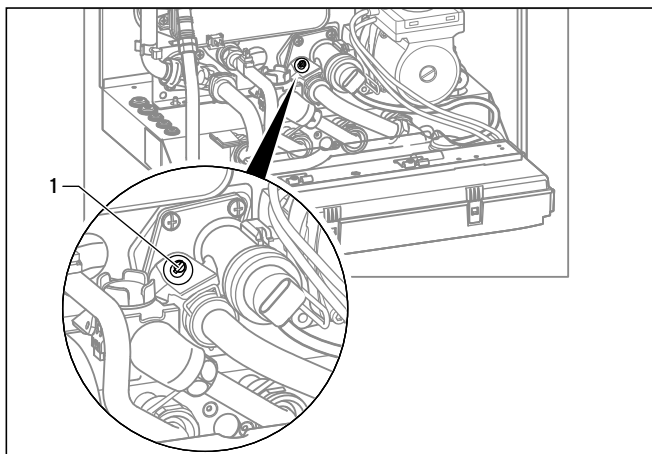
Abb. 7.3 Überströmventil einstellen
