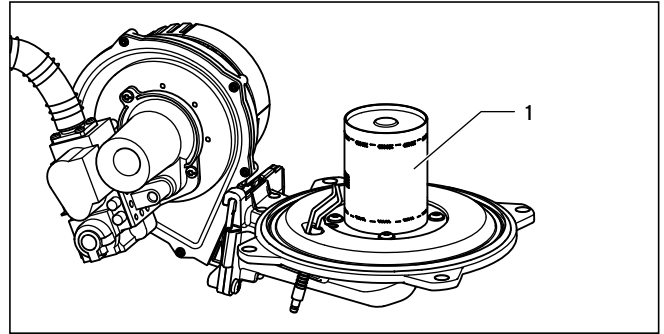
Abb. 8.4 Brenner prüfen
