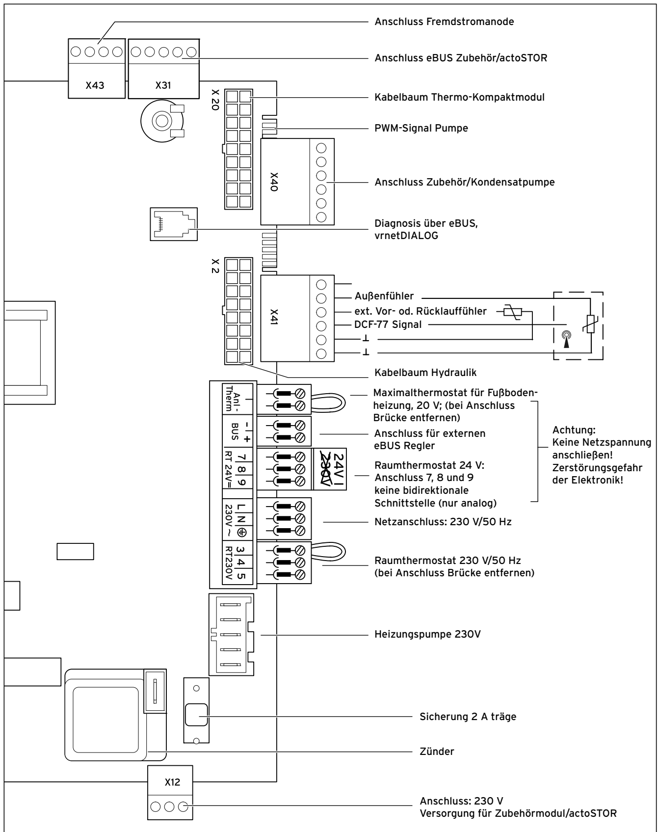
Abb. 5.10 Anschlussplan ecoTEC
