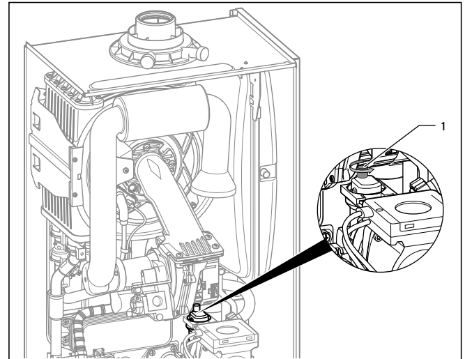
Abb. 6.2 Schnellentlüfter
