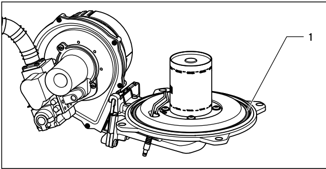
Abb. 8.5 Brenntürdichtung ersetzen
