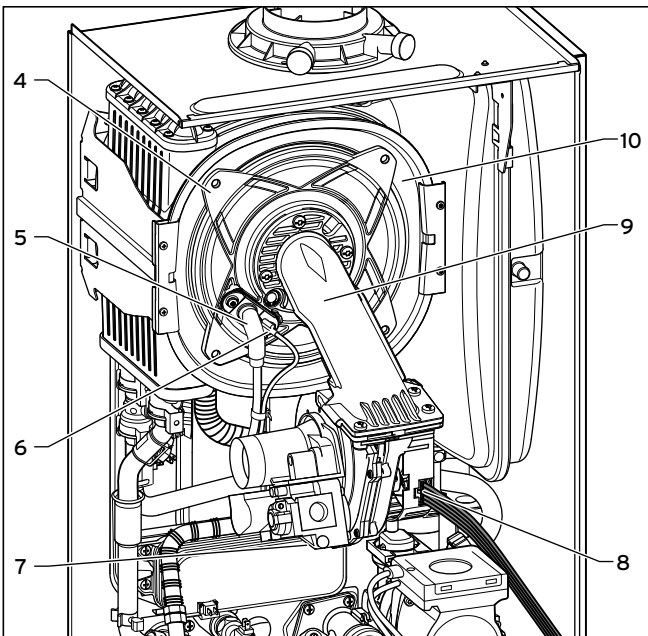
Abb. 8.6 Thermo-Kompaktmodul einbauen
