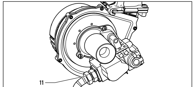
Abb. 8.8 Gasdichtheit prüfen
