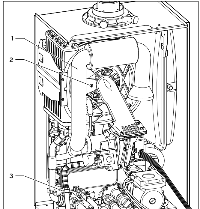
Abb. 8.7 Gaszuleitung anschließen
