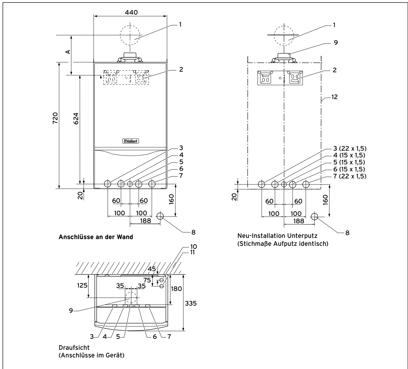
Abb. 4.2 Anschlussmaße in mm
