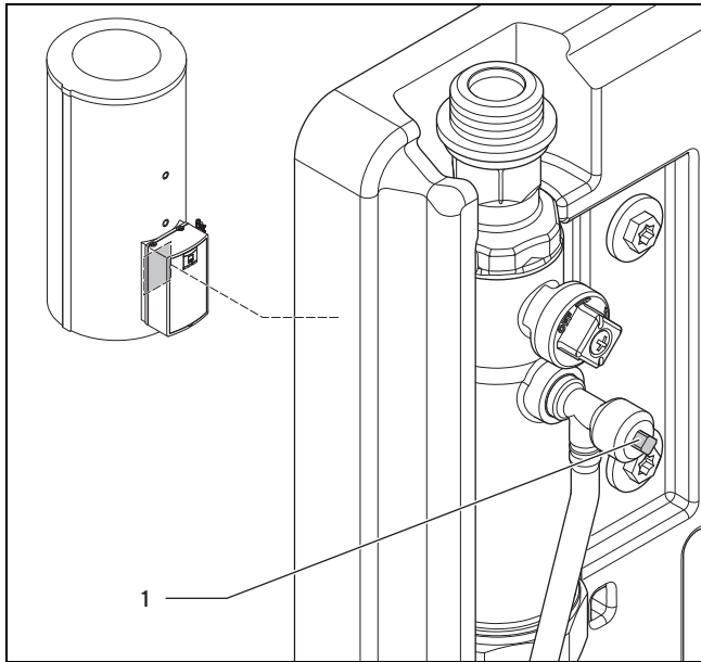
1 Entlüfterschraube
