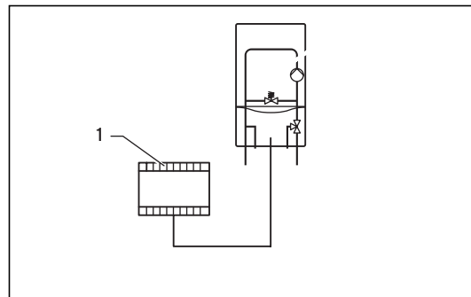
Fig. 5.1 Collegamento dell'interfaccia da 0-10 V
