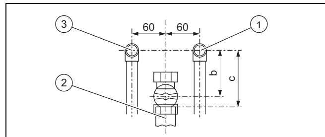
Aufputzinstallation
