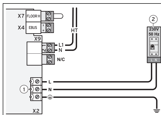
1 Netzanschlussklemmen im Produkt 2 Trennvorrichtung
