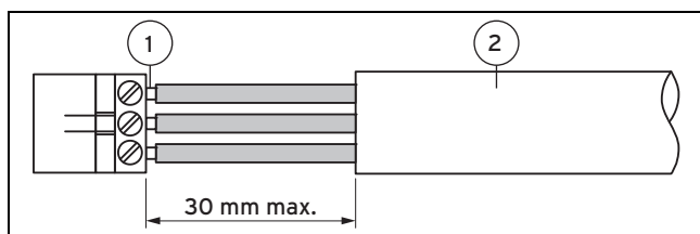
1 Anschlussdrähte 2 Isolierung
