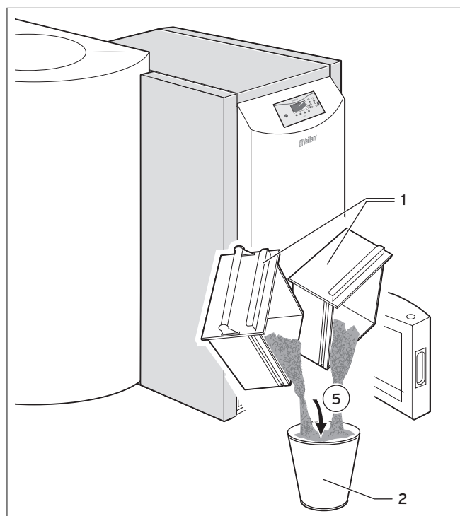
Abb. 9.11 Aschebehälter leeren
