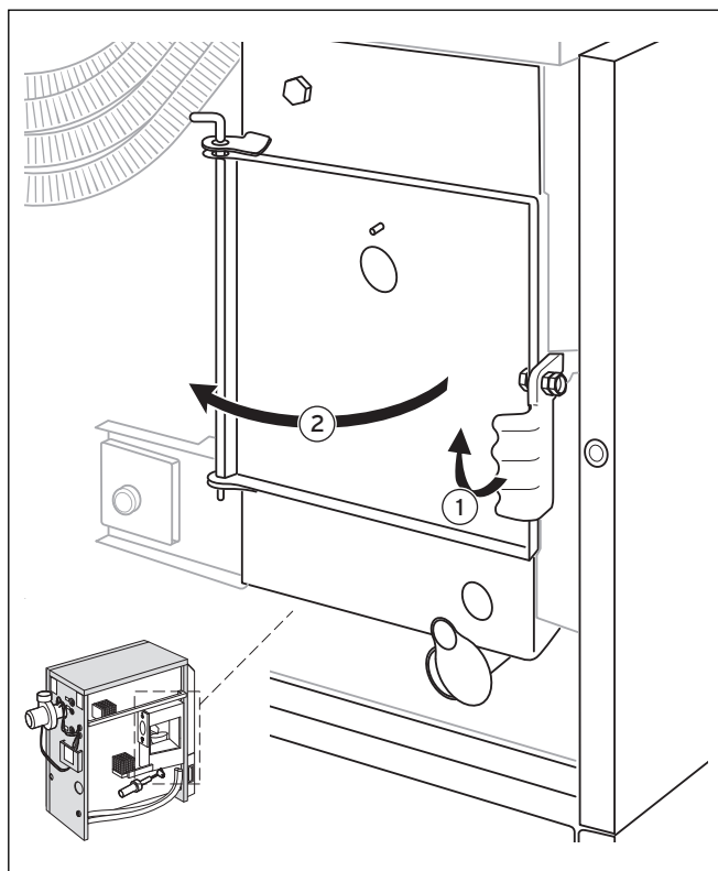
Abb. 9.6 Brennkammertür öffnen
