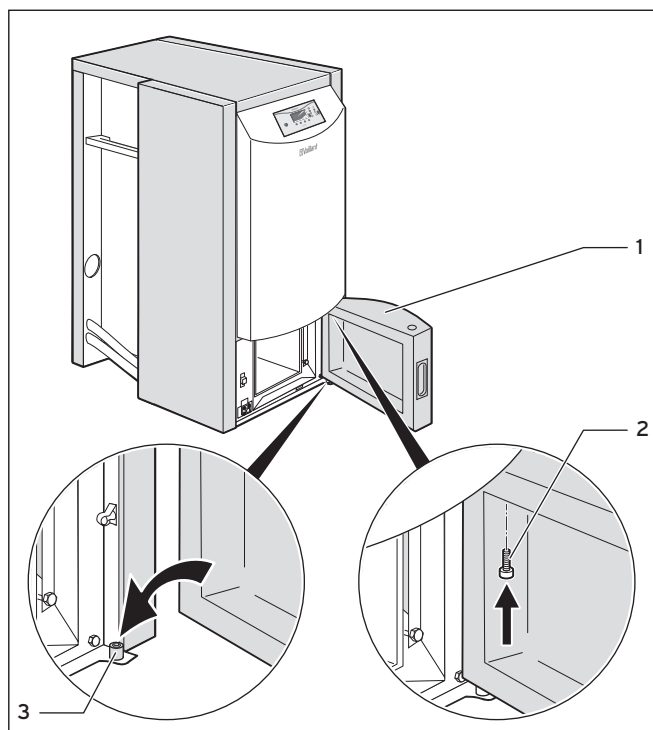
Abb. 4.5 Aschenladentür montieren
