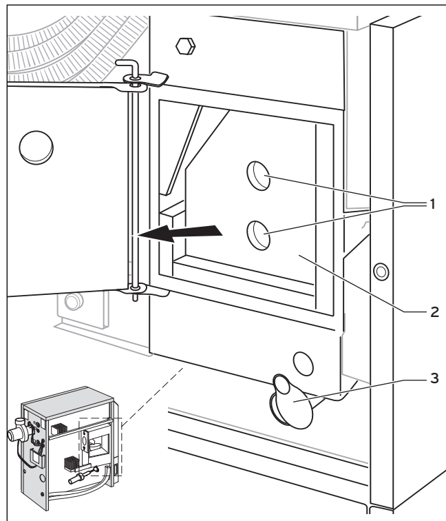
Abb. 9.7 Brennraumisolierung entfernen
