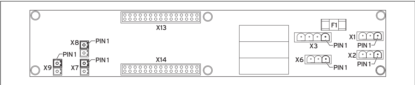
Abb. 6.14 Pufferspeichermodul
