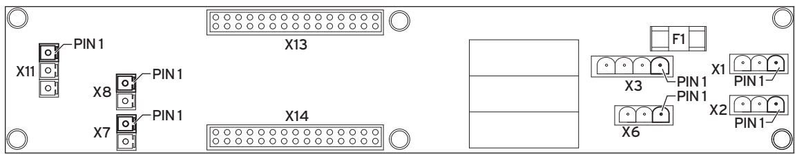
Abb. 6.12 Heizkreismodul
