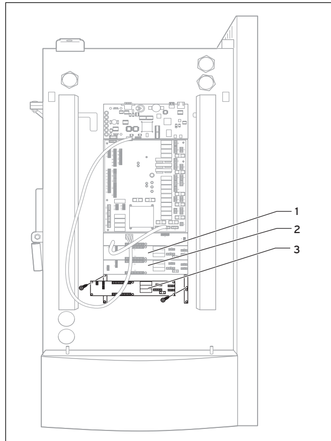
Abb. 6.13 Zubehörmodul anschließen
