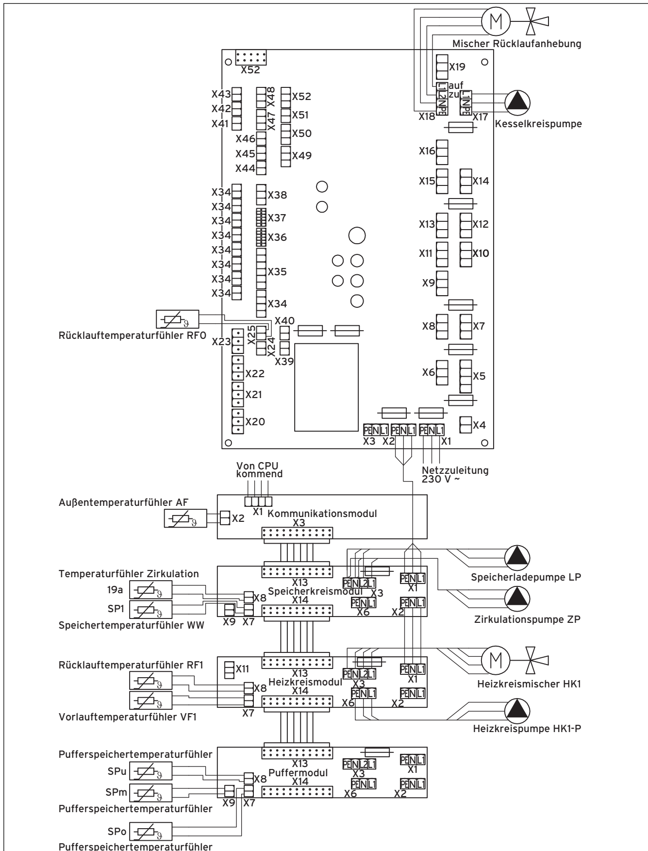
Abb. 6.16 Verdrahtungsplan 1
