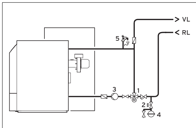
Abb. 5.2 Heizungsseitiges Anschlusschema
