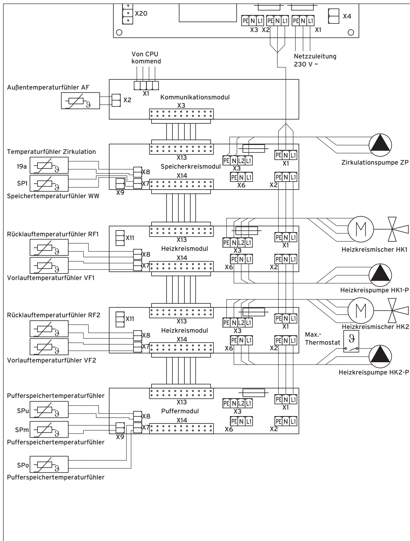
Abb. 6.24 Verdrahtungsplan 5
