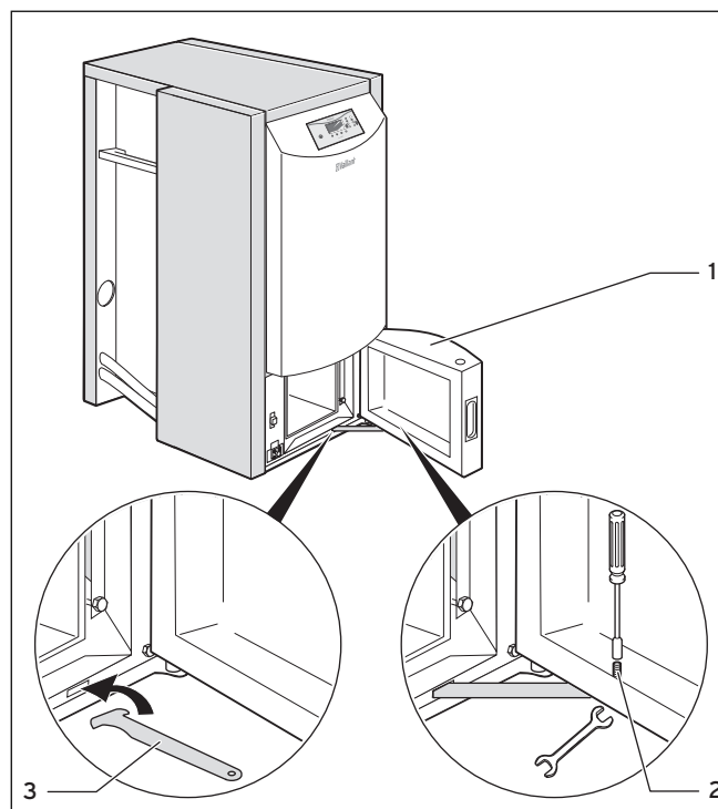
Abb. 4.6 Türstopper montieren
