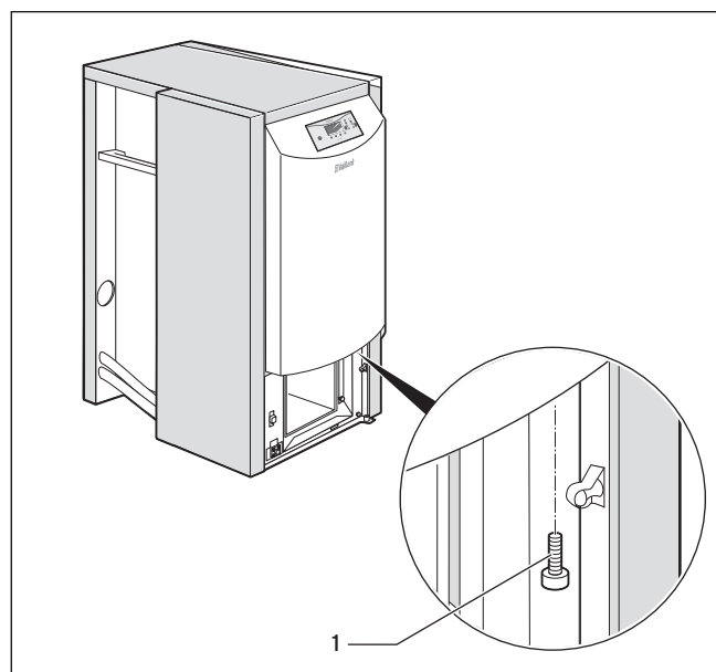
Abb. 4.4 Befestigungsschraube herausnehmen
