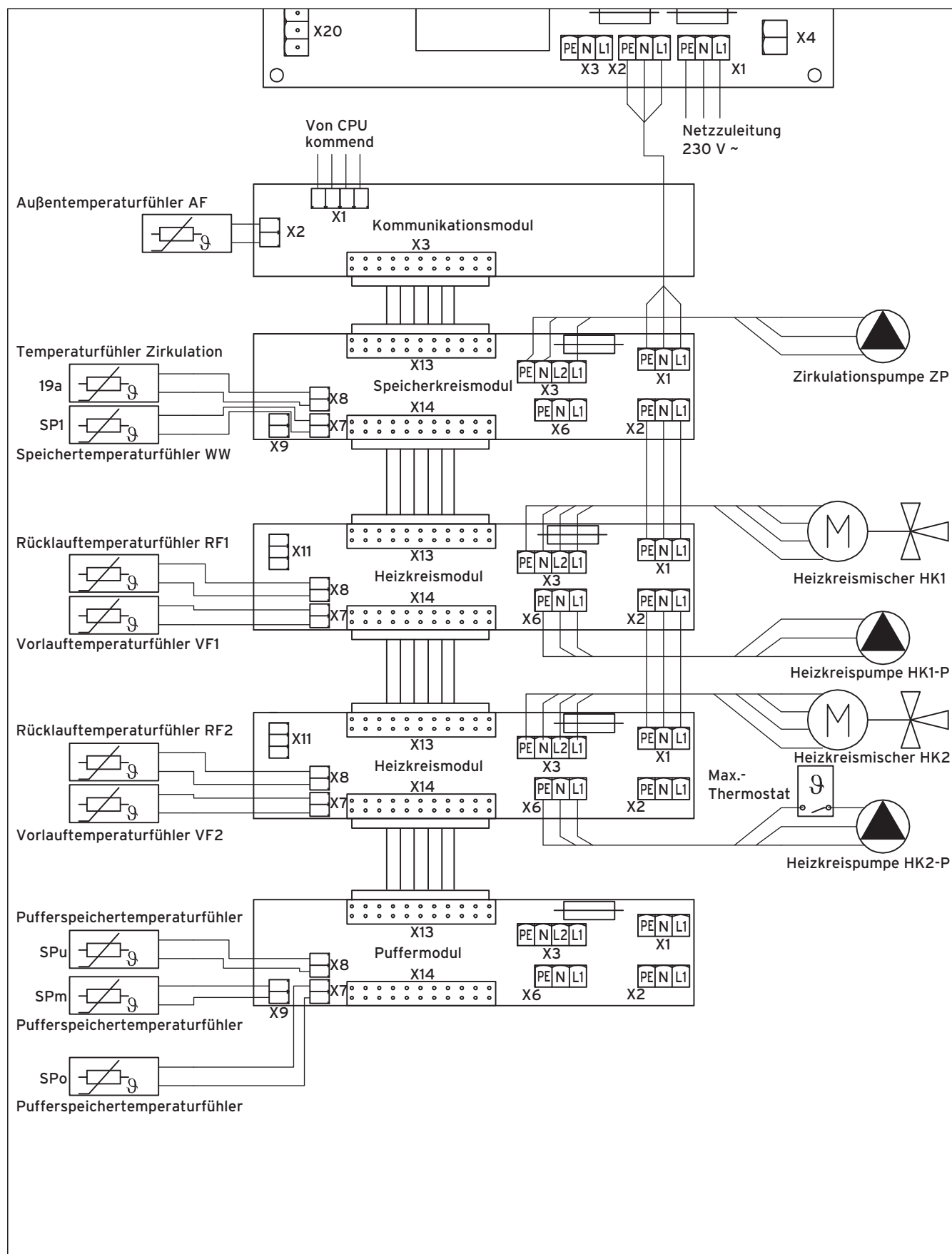
Abb. 6.22 Verdrahtungsplan 4
