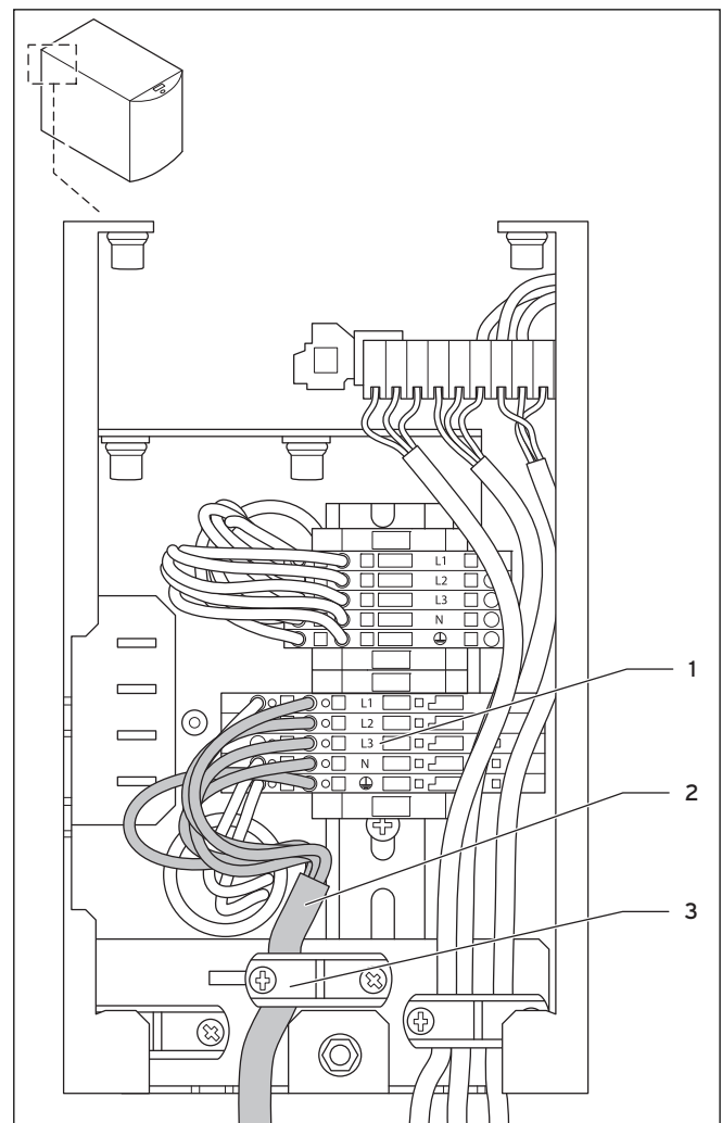
6.3 Netzanschluss herstellen
