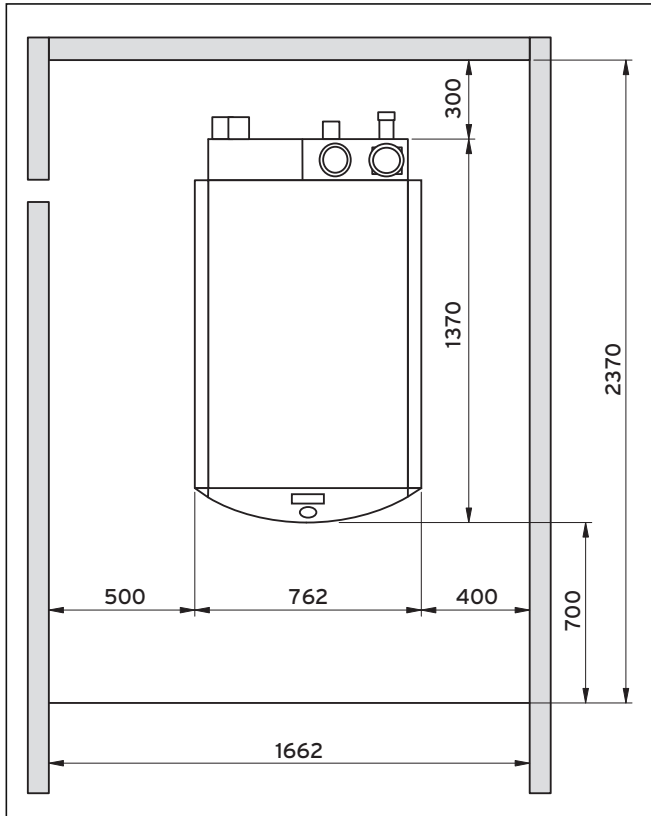
4.5 Mindestabstände seitlich
