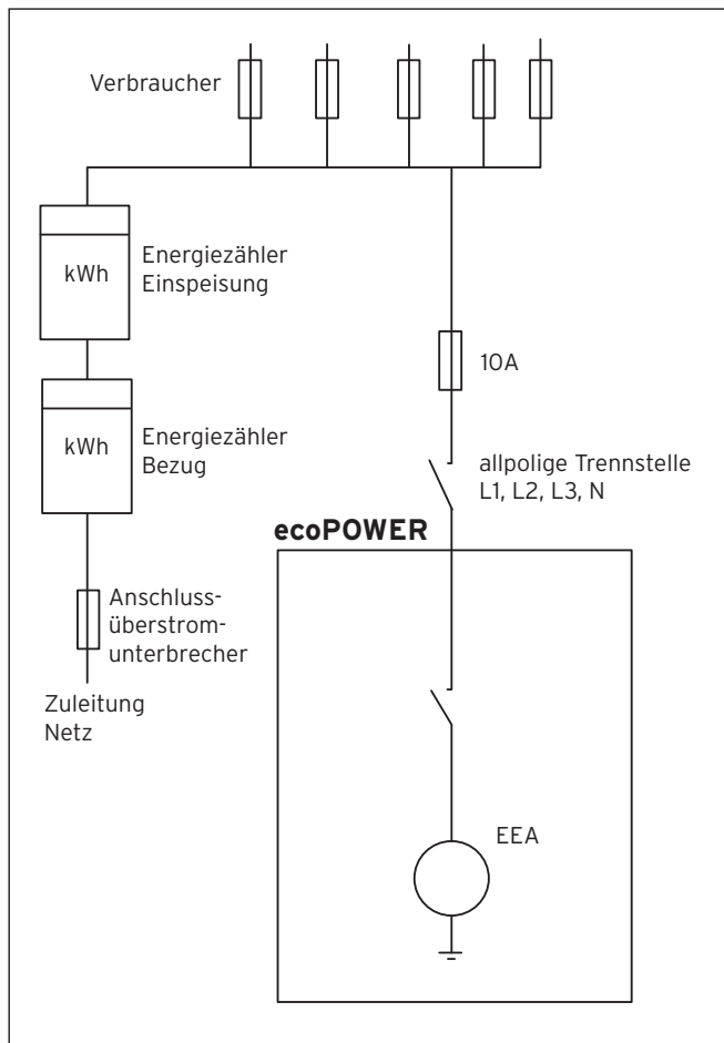
6.2 Einbindung an das öffentliche Stromnetz mit zusätzlichem Zähler
