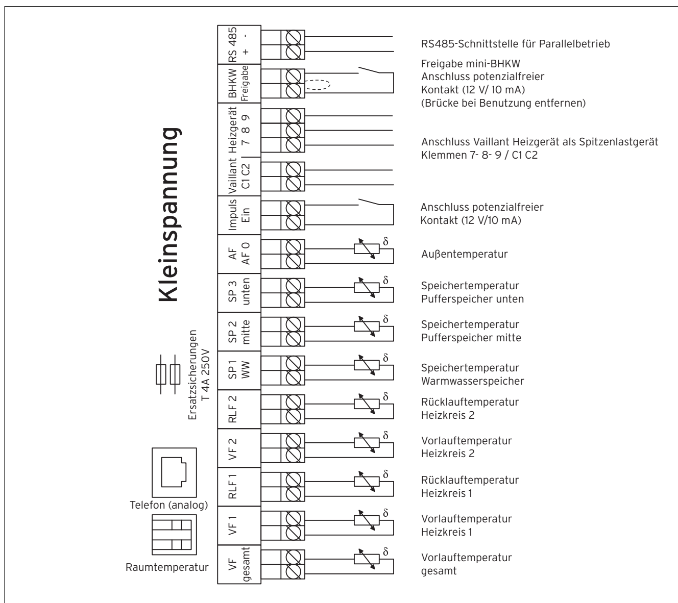
6.5 Verbindungsschaltplan: Kleinspannung
