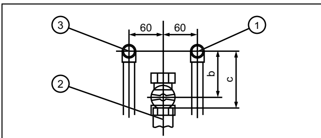
Aufputzinstallation
