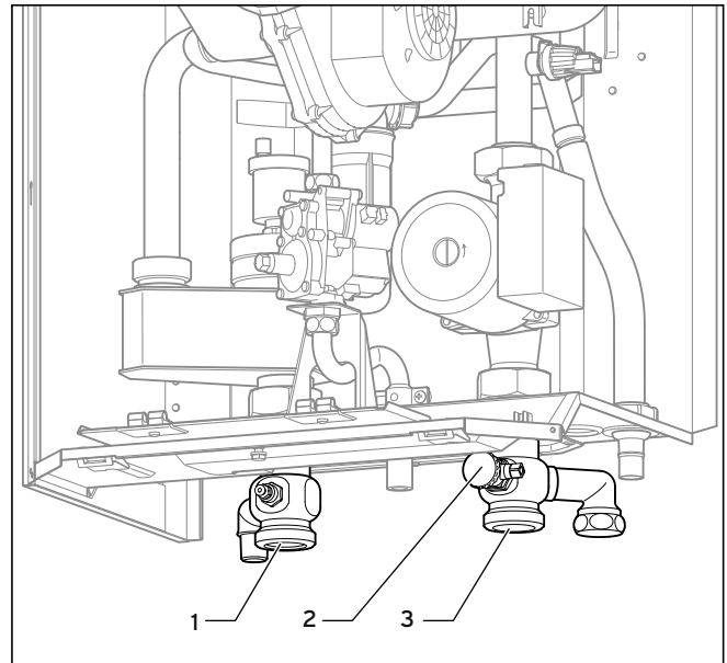
Abb. 5.11 Heizungsanschluss
