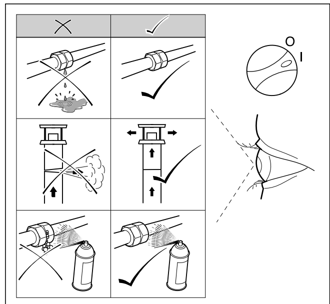
Abb. 6.6 Dichtheitsprüfung
