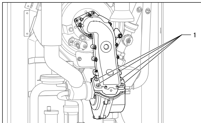
Abb. 10.2 Verschraubung Gasarmatur/Gebläse
