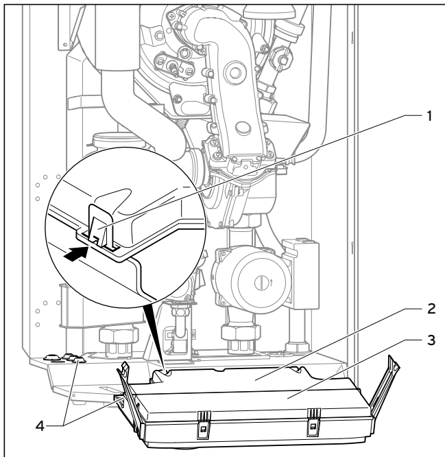
Abb. 5.15 Rückwand der Elektronikbox öffnen
