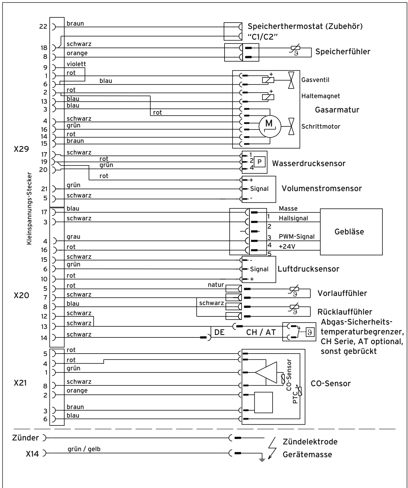
Abb. 5.17 Anschlussplan ecoTEC exclusive VC 356 (Forts. nächste Seite)
