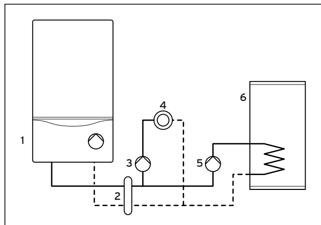
Abb. 5.7 Speichervorrangschaltung und Heizkreis über hydraulische Weiche
