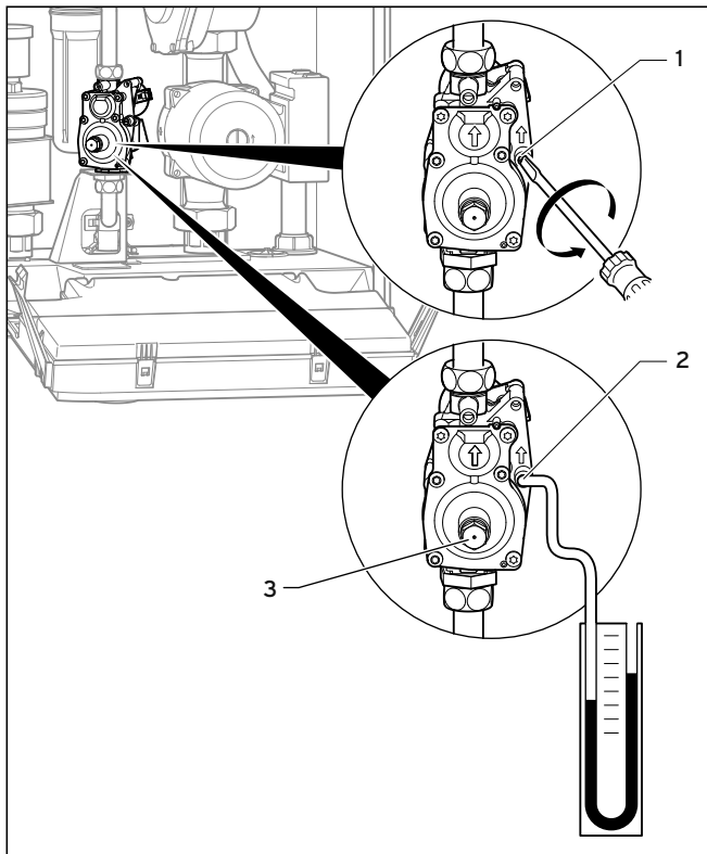
Abb. 6.5 Anschlussdruck (Gasfließdruck) messen
