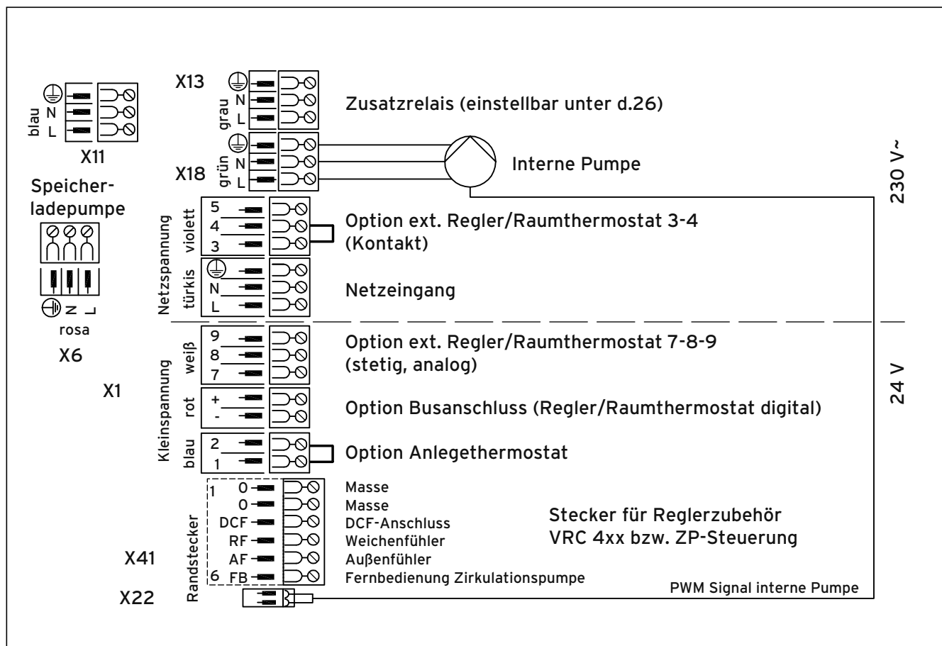
Abb. 5.17 Anschlussplan ecoTEC exclusive VC 356 (Forts.)
