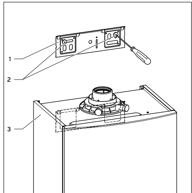
Abb. 4.4 Gerät aufhängen
