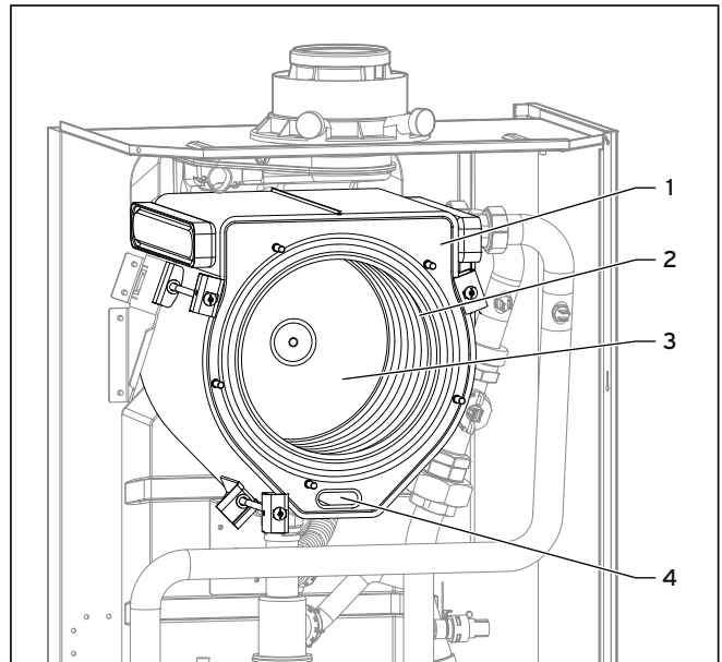
Abb. 8.2 Integral-Kondensations-Wärmetauscher reinigen
