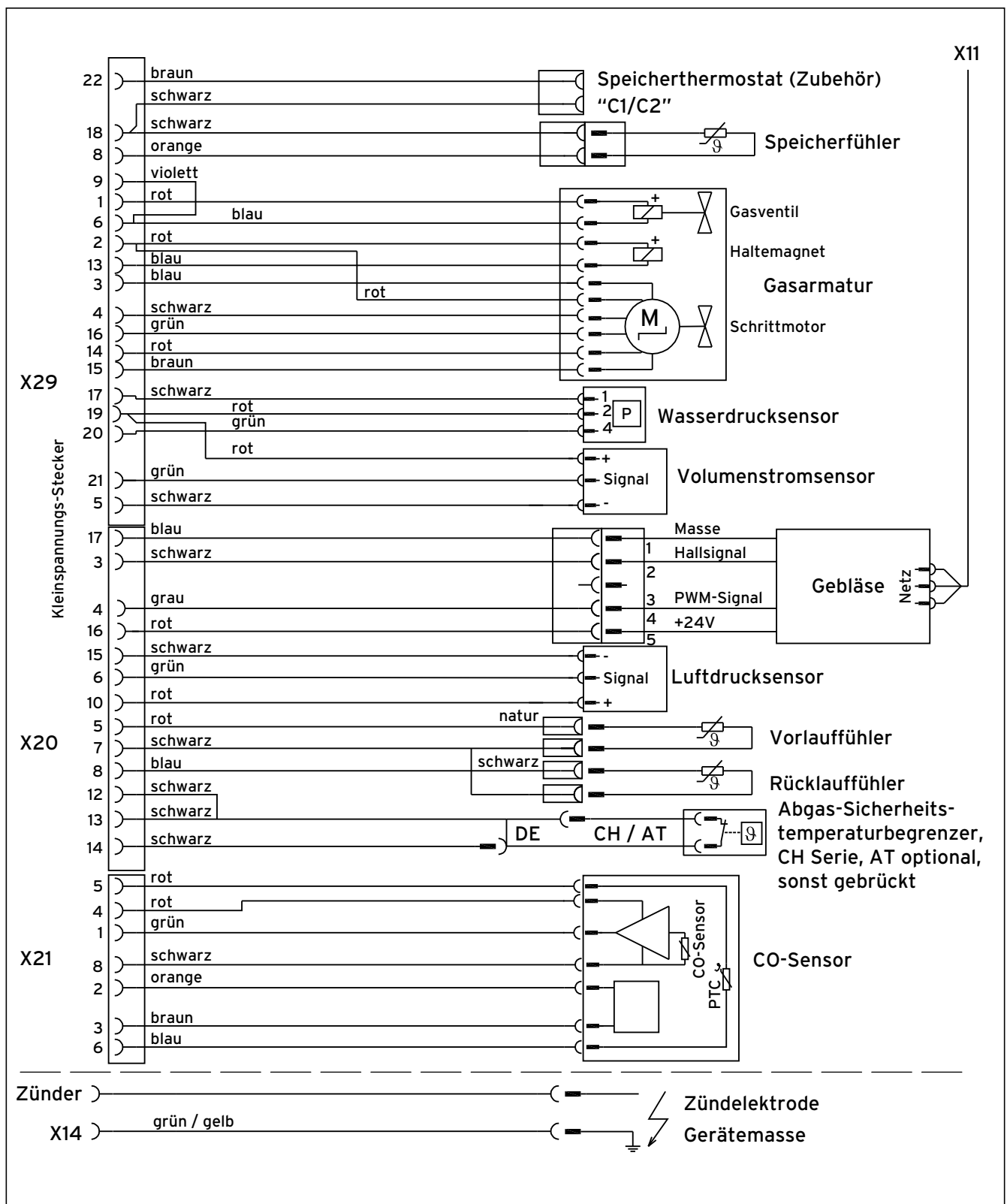
Abb. 5.18 Anschlussplan ecoTEC exclusive VC 466 (Forts. nächste Seite)
