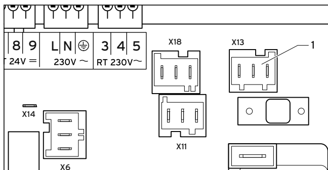
Abb. 5.2 Elektrischer Anschluss Heizpumpe hinter hydraulischer Weiche
