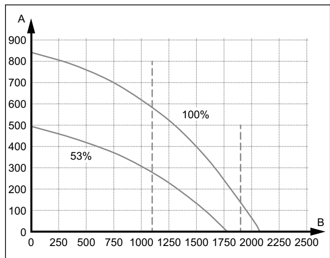
Abb. 7.2 Pumpendiagramm VC DE 356/4-7 A und VC DE 466/4-7 A
