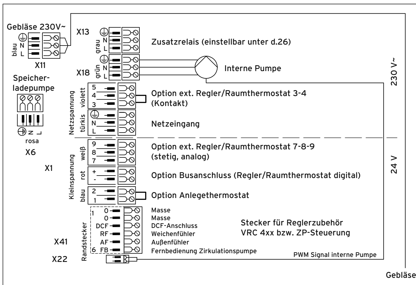
Abb. 5.18 Anschlussplan ecoTEC exclusive VC 466 (Forts.)
