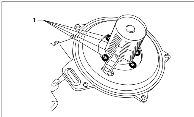
Abb. 10.1 Brenner austauschen
