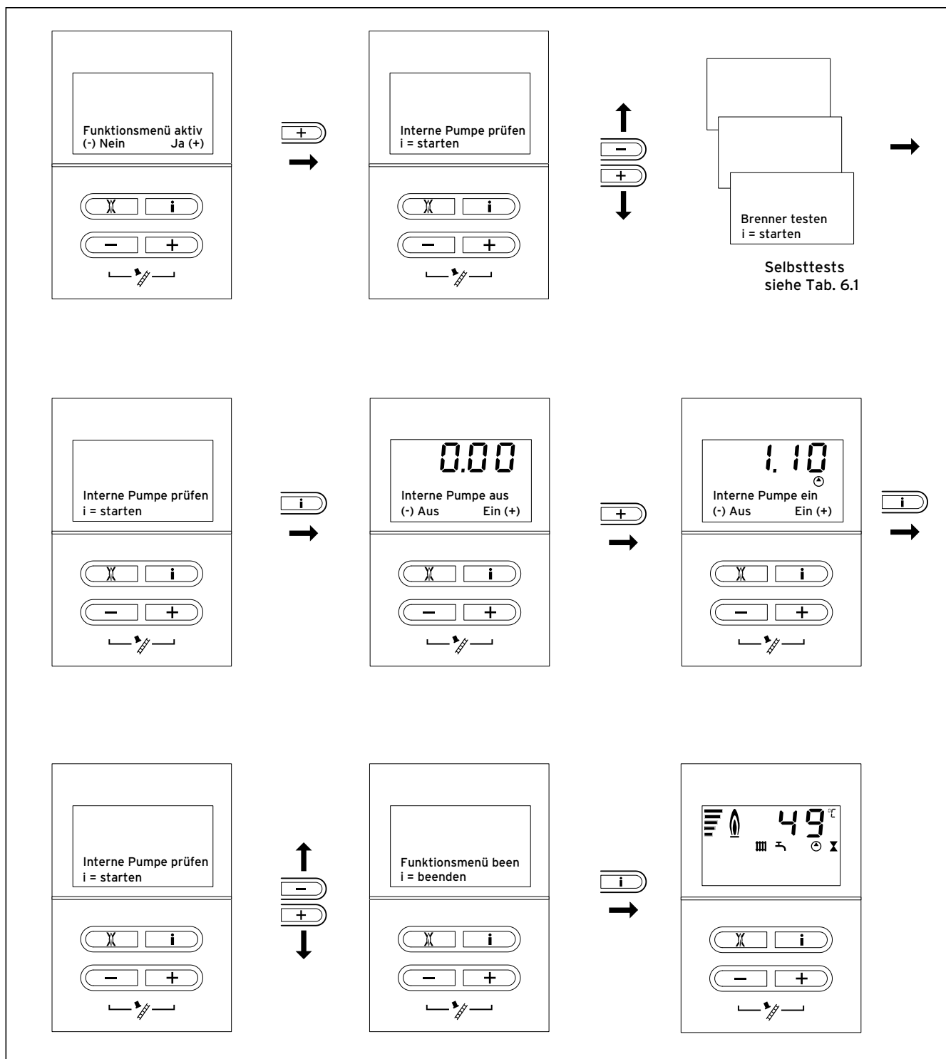
Abb. 6.1 Bedienung Funktionsmenü
