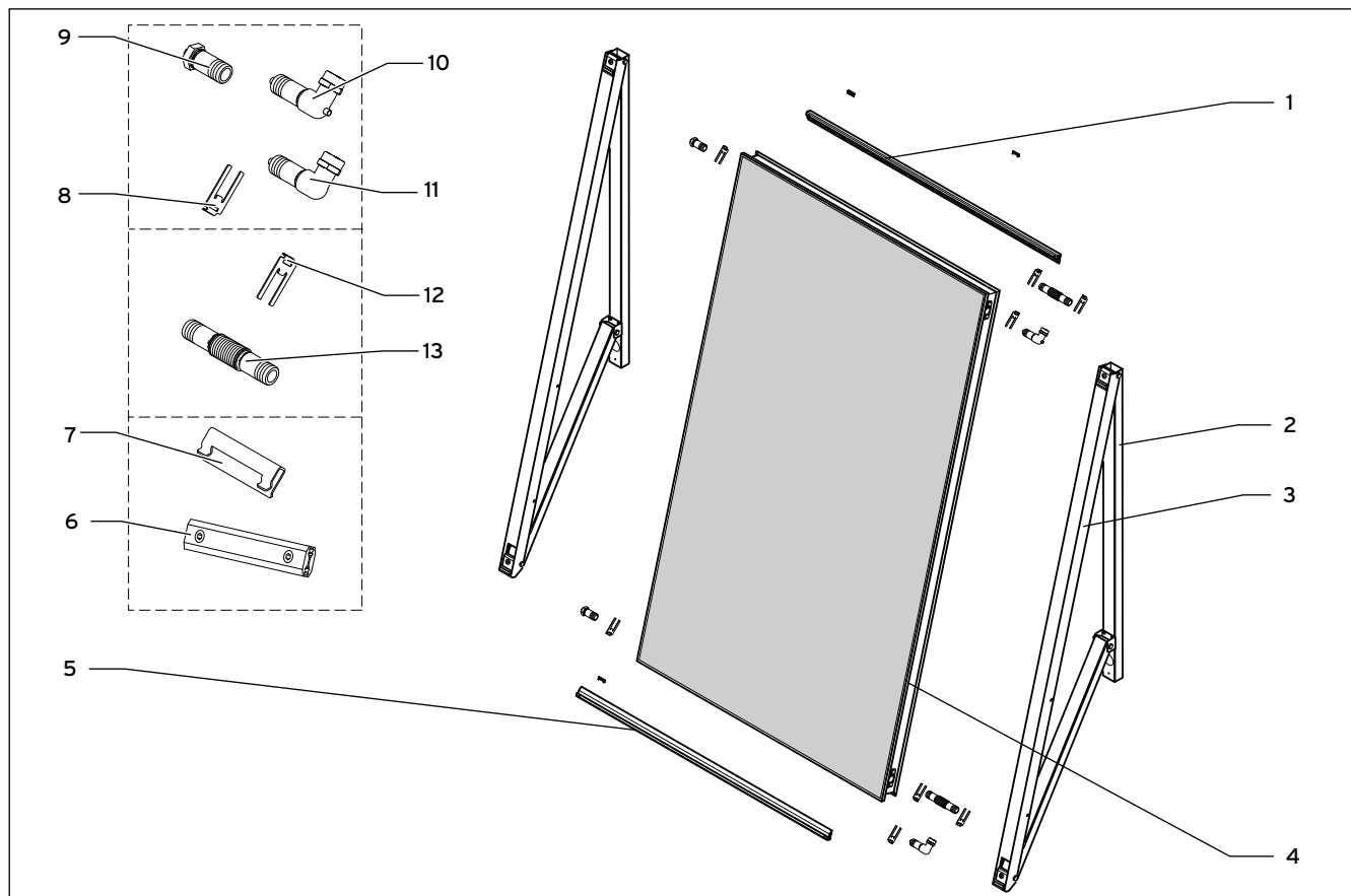
Abb. 5.2 Einbausatz
