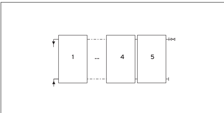
Abb. 4.2 Reihenschaltung 1 - 5 Flachkollektoren
