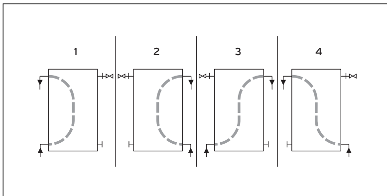
Abb. 4.1 Durchströmungsrichtung
