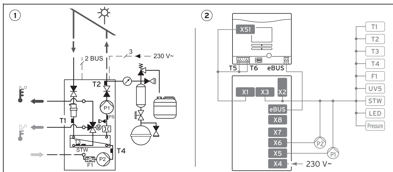
1 Hydraulikschema
