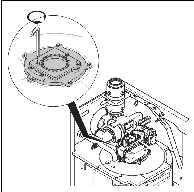
1 Ablageposition 2 Verriegelungsnase
