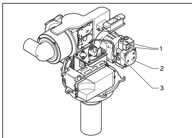
1 Magnetventile 2 Ölpumpe 3 Ölleitung
