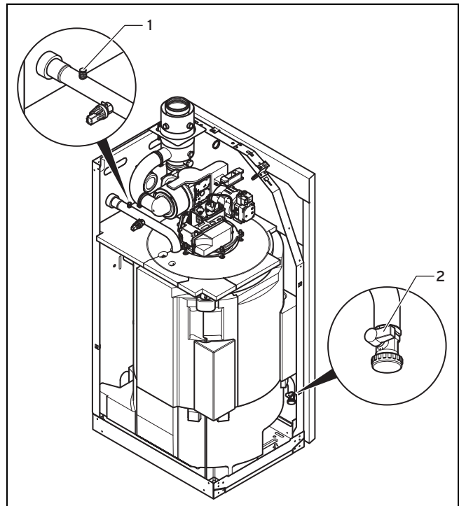
1 Entlüftungsnippel
