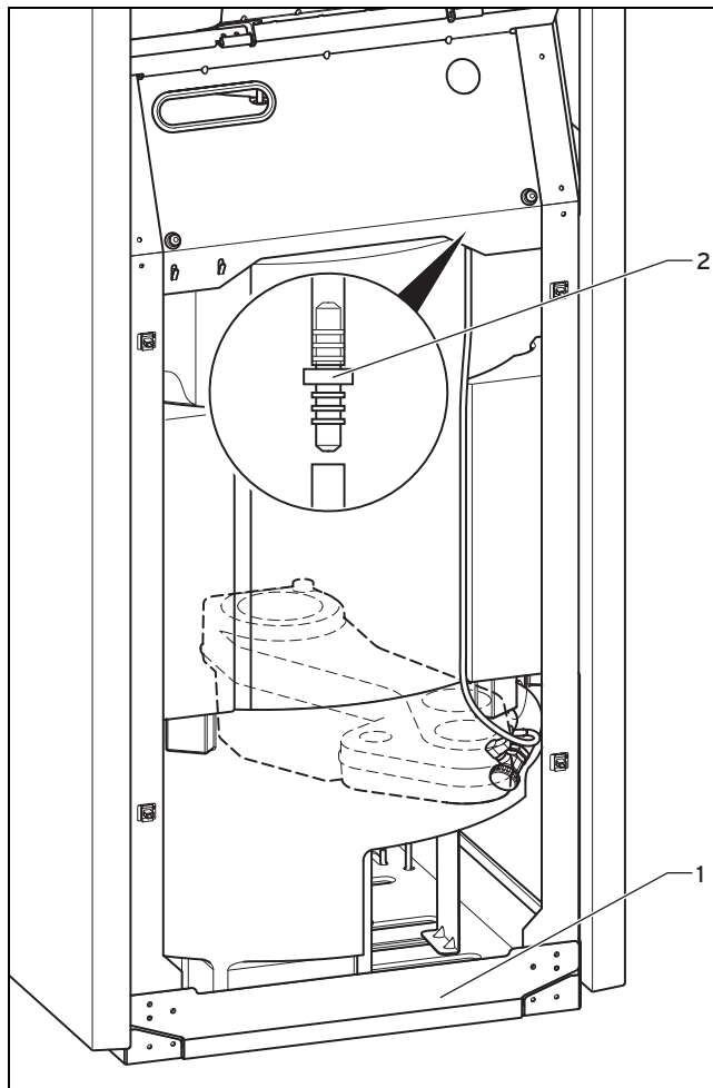
1 Strebe abschrauben 2 Schlauch trennen
