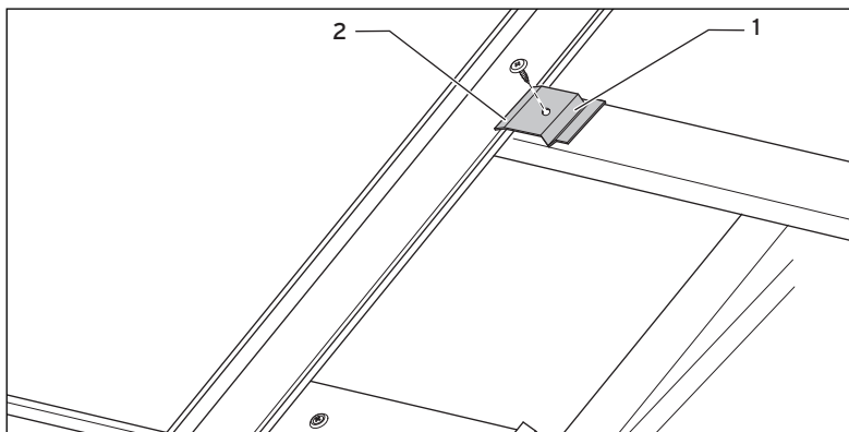
Abb. 5.12 Kollektor anschrauben
